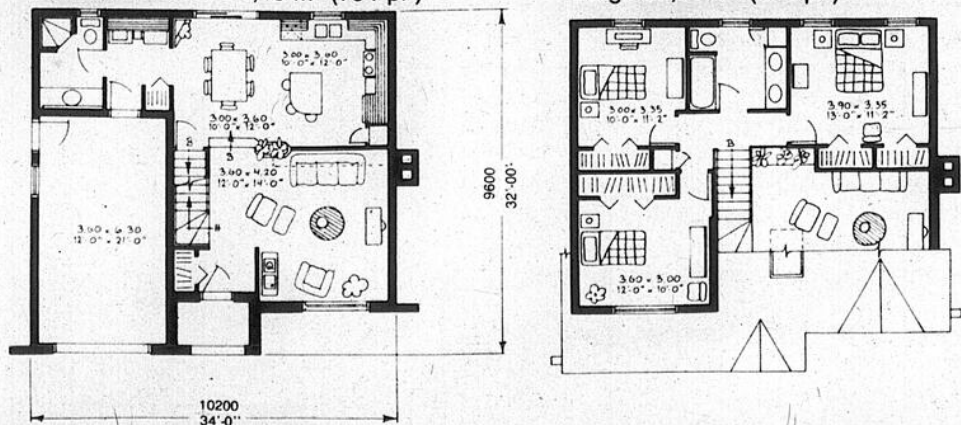
Rez-de-chaussée 71,46 m 2 (794 pi 2 )
