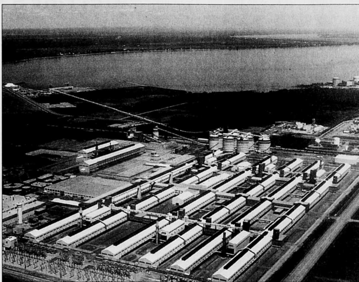
ASSOCIATION DE L'INDUSTRIE DE L'ALUMINIUM L'Aluminerie de Bécancour, la plus importante après celle de Baie-Comeau, produit 360 000 tonnes d'aluminium par an au bord du Saint-Laurent.
