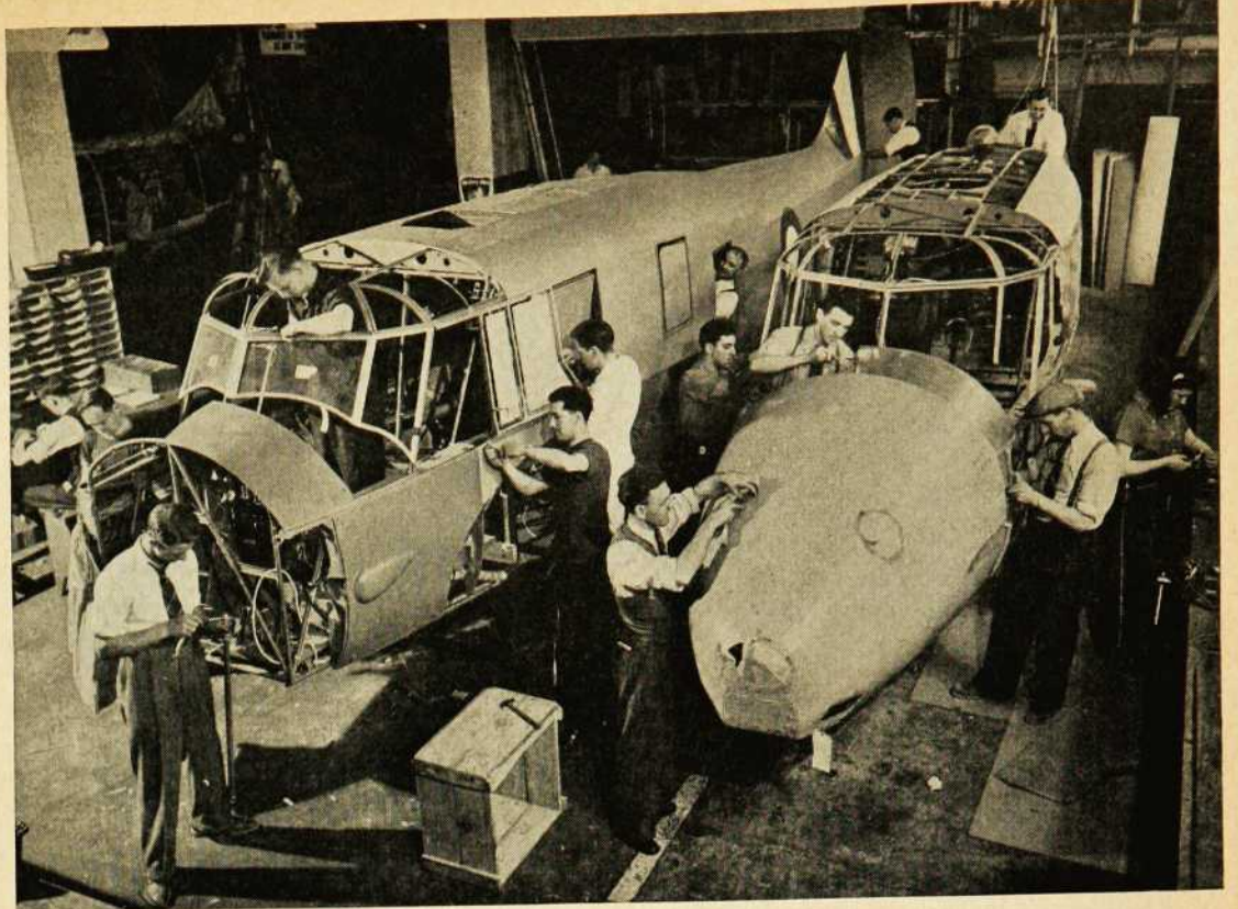
Appareil Avro-Anson en construction dans une avionnerie de Montréal.
