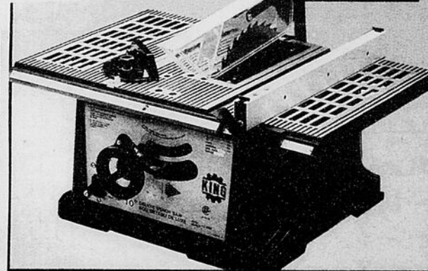
075-100 BANC DE SCIE 10" SUR ROULEMENT À BILLES. 15 AMPERES. PROTEGE-LAME ET SORTIE POUR DÉPOUSSIÉREUR. RING.
