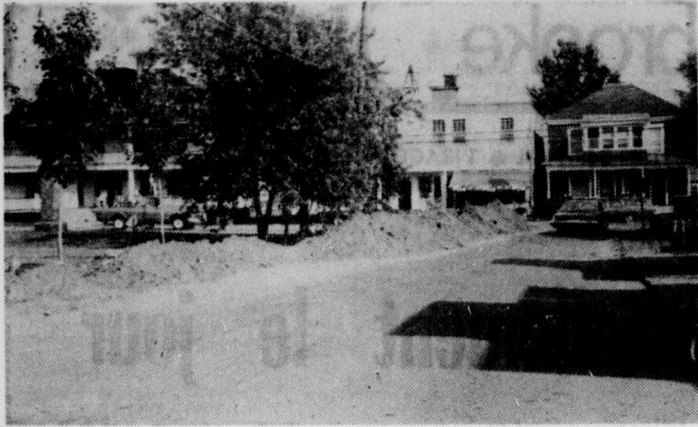
La compagnie International Water Co. qui dessert Derby Line, Vt, Rock Island et Stanstead a procédé à l'installation d'un tuyau de plus grande dimension sur une distance d'environ 80 pieds, rue Maple à Stanstead. Le nouveau tuyau mesurera 6 pouces de diamètre au lieu de 4 pouces.
