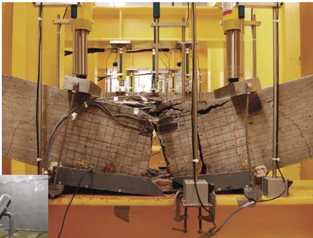
▲ Défaillance d'une poutre de pont causée par chargement couple, Laboratoire de chargement couple, CNRC Photo : CNRC
