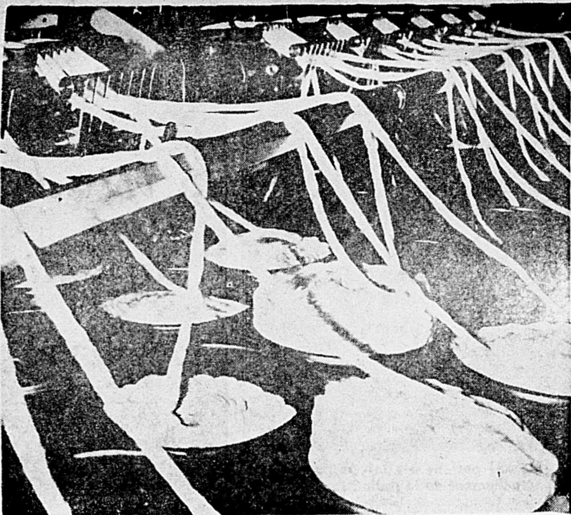
Après que le coton a passé à la cardeuse, au moulin, il doit suivre ensuite toute une série de procédés avant de devenir en fil. L'un d'eux est la tréfilerie qui consiste à presser plusieurs rubans en un seul brin.
