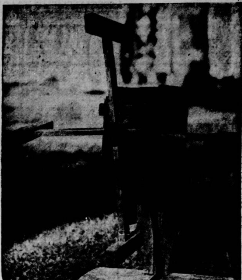
Un ancien dévidoir à laine, dont chaque tour indiquait quatre verges de longueur. Ce dévidoir était entièrement en bois, de même que le cliquet, à ressort, qui bloquait la roue dentée, également en bois.
