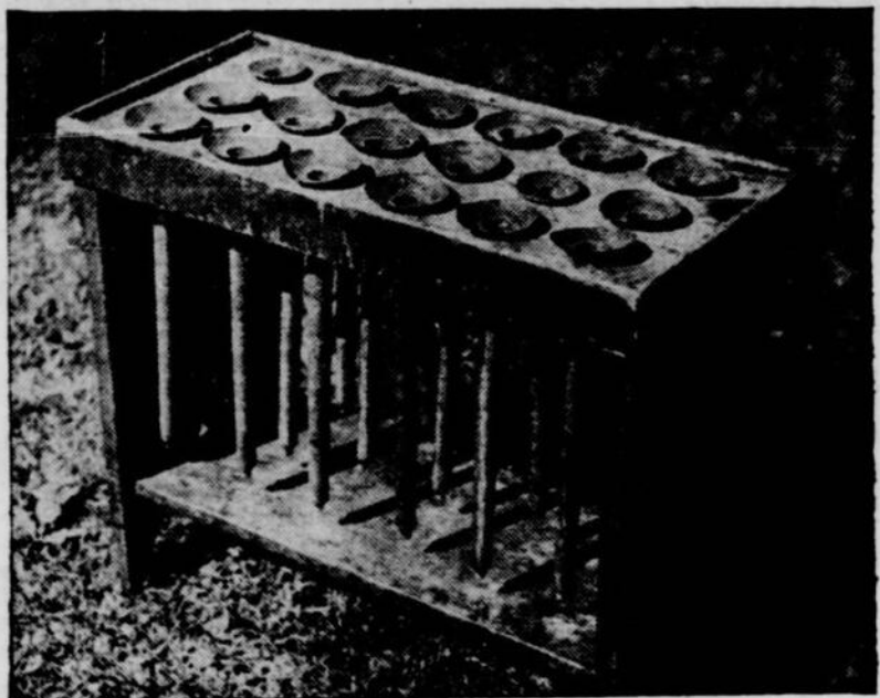
Ici, l'on voit un vieux moule à chandelles, dont les manufacturiers se servaient, vers 1860, pour couler 18 chandelles à la fois. La mèche était assujettie au bout pointu, par un simple noeud.
