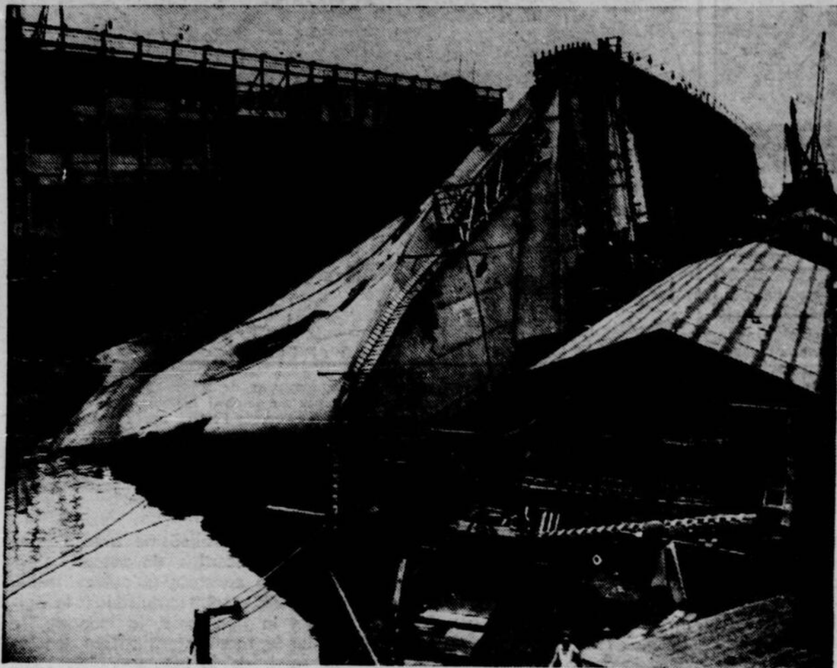
Immobile dans la boue de la rivière Hudson, depuis qu'il fut ravagé par un incendie et se pencha complètement sur le côté, à son quai, le 10 février 1942, le gigantesque océanique français "Normandie" de 79,280 tonneaux est à la veille de se remettre parfaitement d'aplomb. Au moment de l'accident, son nom avait été changé en celui du navire de guerre américain "Lafayette". Ici sa coque avait été soulevée de 13 pieds. Les travaux pour le redressement avaient commencé le 15 mai 1942
