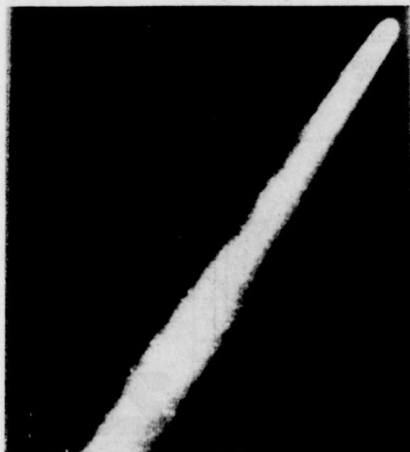
La comète de Halley telle que vue en 1910.
