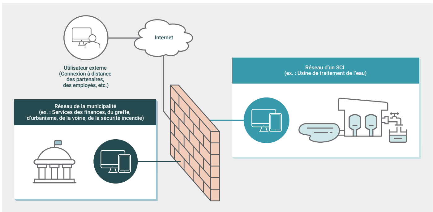
Figure 5 Exemple de cloisonnement du réseau d'un SCI
