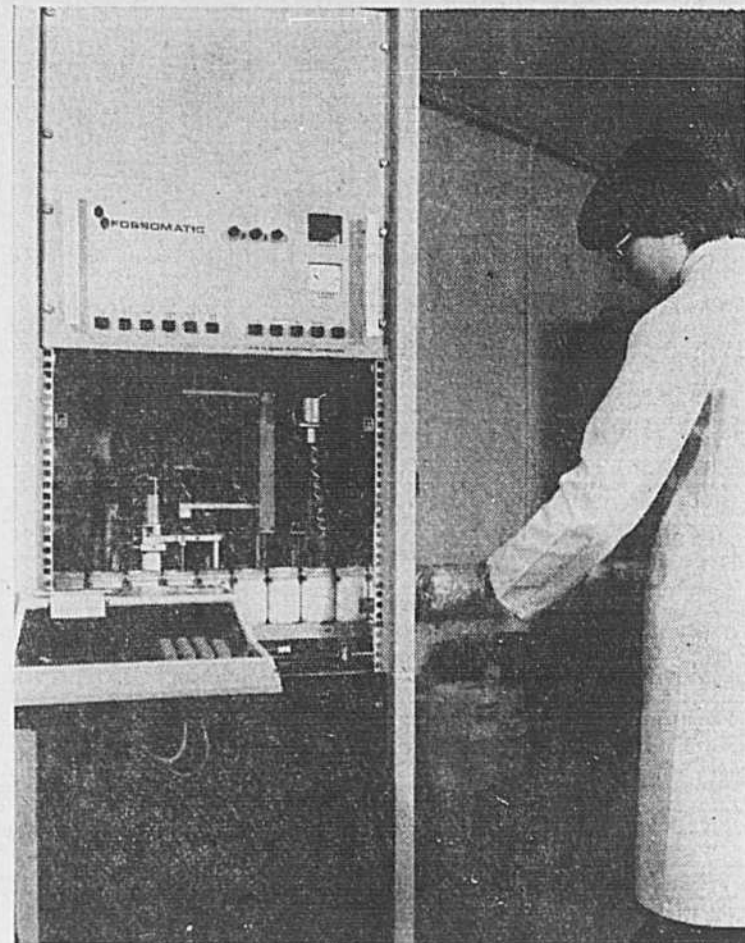
Le Service d'analyse du lait du pavillon Macdonald College de l'Université McGill utilise les instruments les plus perfectionnés. Sur la photo, Susan Peters, technicienne, se sert de l'appareil d'analyse Fossomatic, qui détermine le cas échéant la gravité de la mammité chez la vache.
