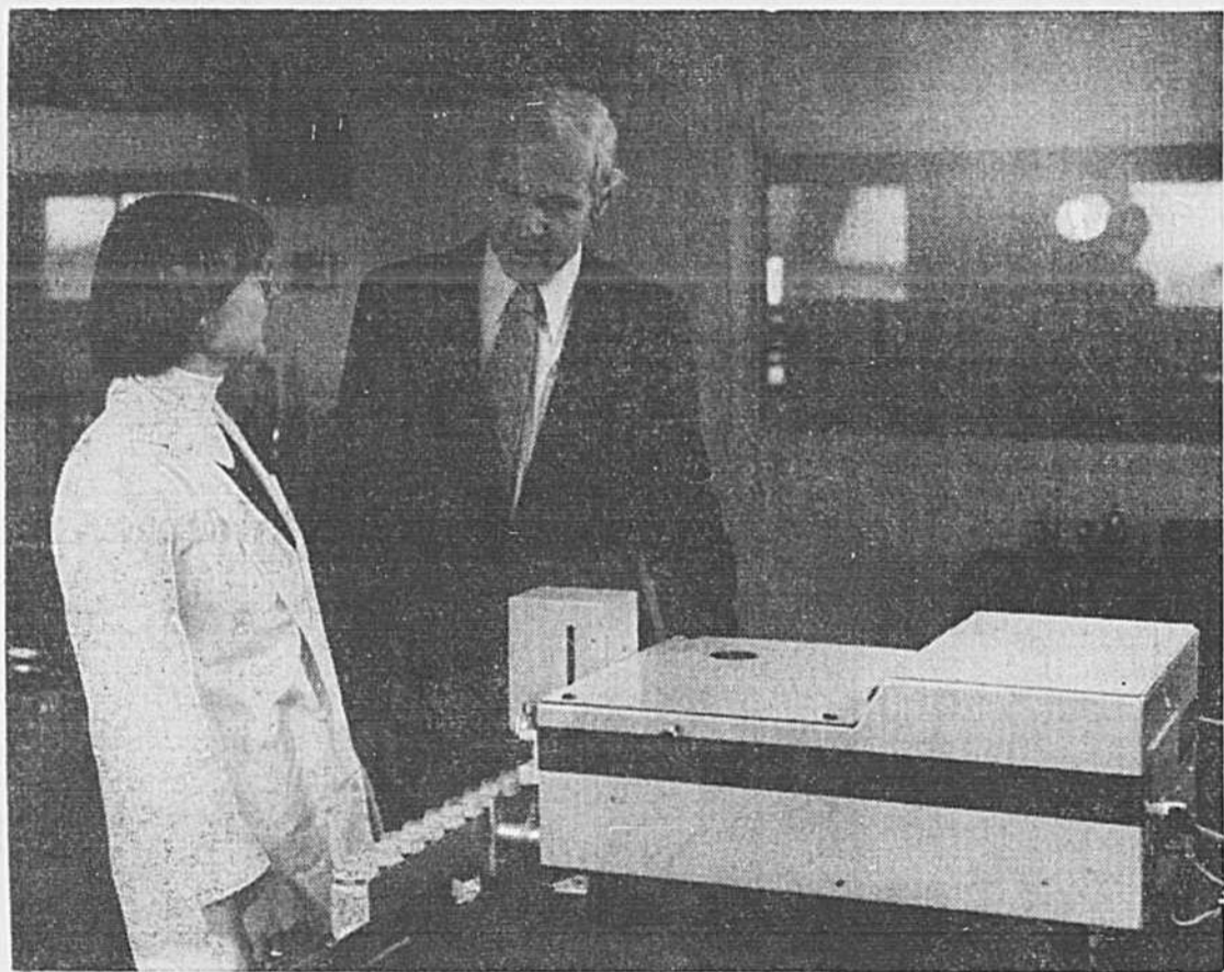
Le docteur John Moxley, directeur du Service d'analyse du lait du pavillon Macdonald College de l'Université McGill et aussi du ministère de l'Agriculture du Québec, et Susan Peters, technicienne, en train de discuter du résultat de l'appareil «Milko-Scan», un appareil complètement automatique qui sert à mesurer le gras, les protéines et le lactose contenus dans le lait.
