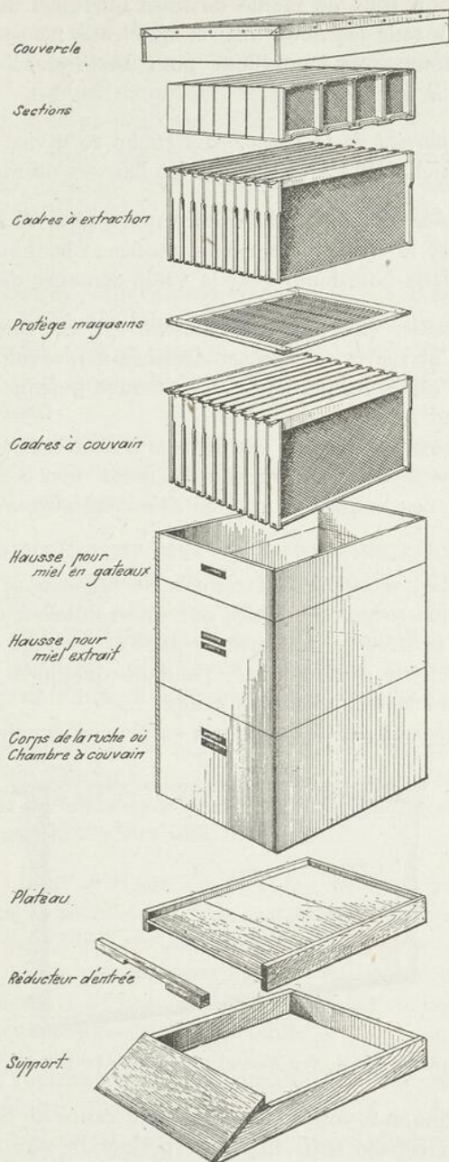
Une ruche mobile et ses parties
