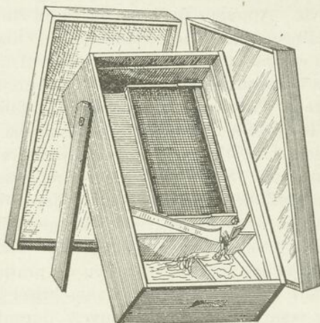
Cérificateur solaire Doolittle
