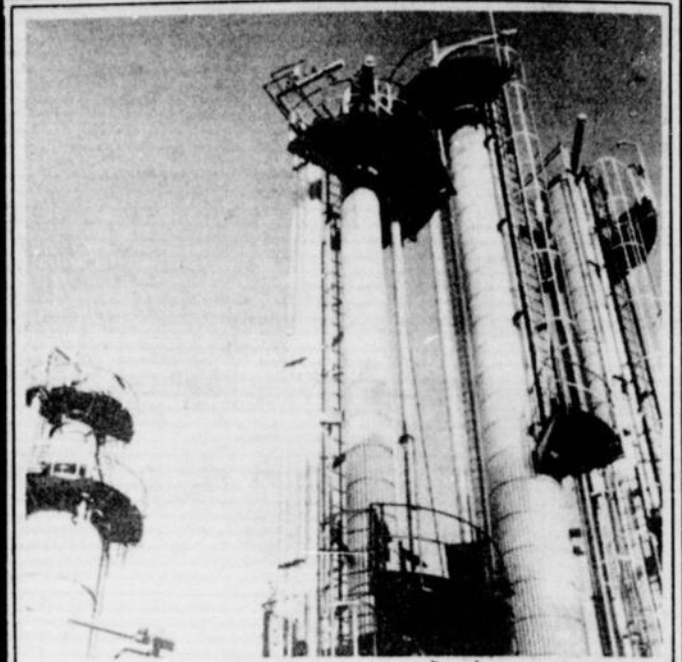
Pour raffiner le pétrole brut et le transformer en essence ou en huile à chauffage, il faut investir dans l'équipement. Cet "hydrofiner" de $6 millions a été mis en marche au début de 1973 à la raffinerie de l'Imperial Oil à Montréal-Est. Sa principale fonction est de désulfurer des produits comme l'huile de chauffage.
