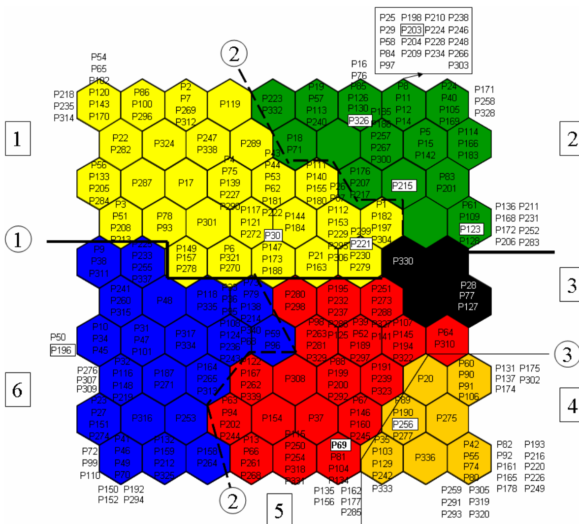
Figure 4.4 : Résultat pour les six groupes de pesticides formés à partir de la carte auto-organisatrice de Kohonen (résultats bruts de l'analyse). Les chiffres encadrés identifient les groupes de pesticides, tandis que les chiffres encerclés représentent les niveaux de différenciation des groupes établis par la U-matrix . Les nombres dans les cellules (e.g. P39) représentent les numéros d'identification des pesticides (voir ANNEXE M).
