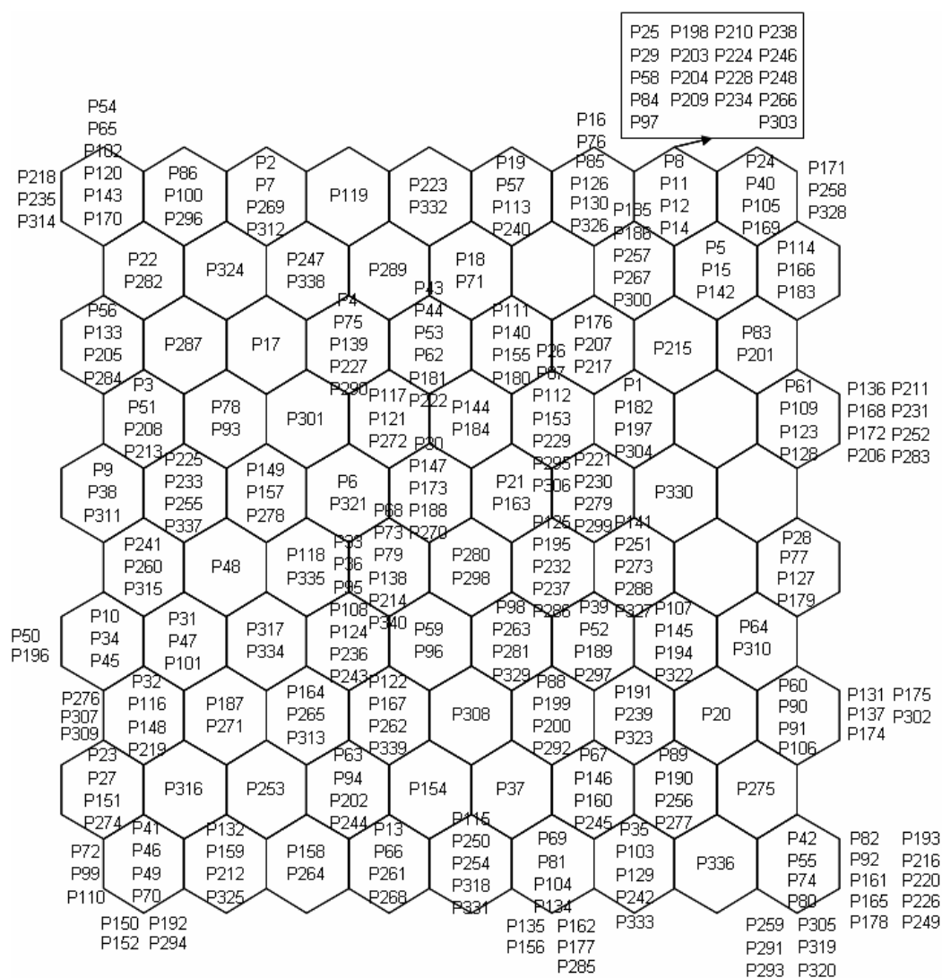
Figure 4.1 : Carte auto-organisatrice de Kohonen.
