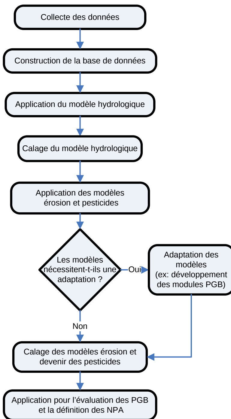
Figure 2.1 : Diagramme des différentes étapes pour l'application d'un modèle sur un bassin versant (tiré de Rousseau et al. , 2006)
