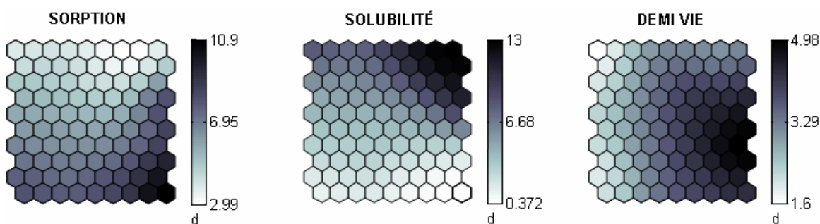
Figure 4.2 : Cartes de distribution issues de la carte auto-organisatrice de Kohonen. Les cellules foncées représentent des valeurs élevées, alors que les cellules pâles représentent des valeurs faibles. L'échelle d indique les valeurs transformées de sorption [ml/g], solubilité [mg/l] et demi-vie [jour] par le logarithme.
