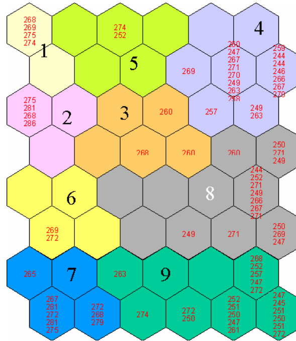
Figure L.2 : Exemple d'une carte auto-organisatrice de Kohonen.
