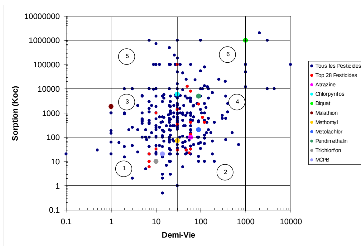
Figure N.1 : Classification (en 6 classes-groupes) des 340 pesticides (banque de données de Hornsby et al. , 1996). « Top 28 pesticides » représente les composés présents à la fois dans la banque de données et dans la liste des 50 pesticides « prioritaires » d'EC. Les composés nominatifs avec un symbole de couleur distinctive comptent parmi les 10 pesticides « Top ten » d'EC, excepté le Métolachlor et le MCPB .
