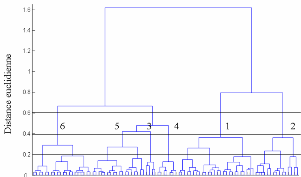
Figure 4.3 : Arbre de classification des pesticides obtenu avec la méthode des cartes auto-organisatrices de Kohonen. Les groupes N° 1 à 6 sont obtenus avec une distance de 0.4.
