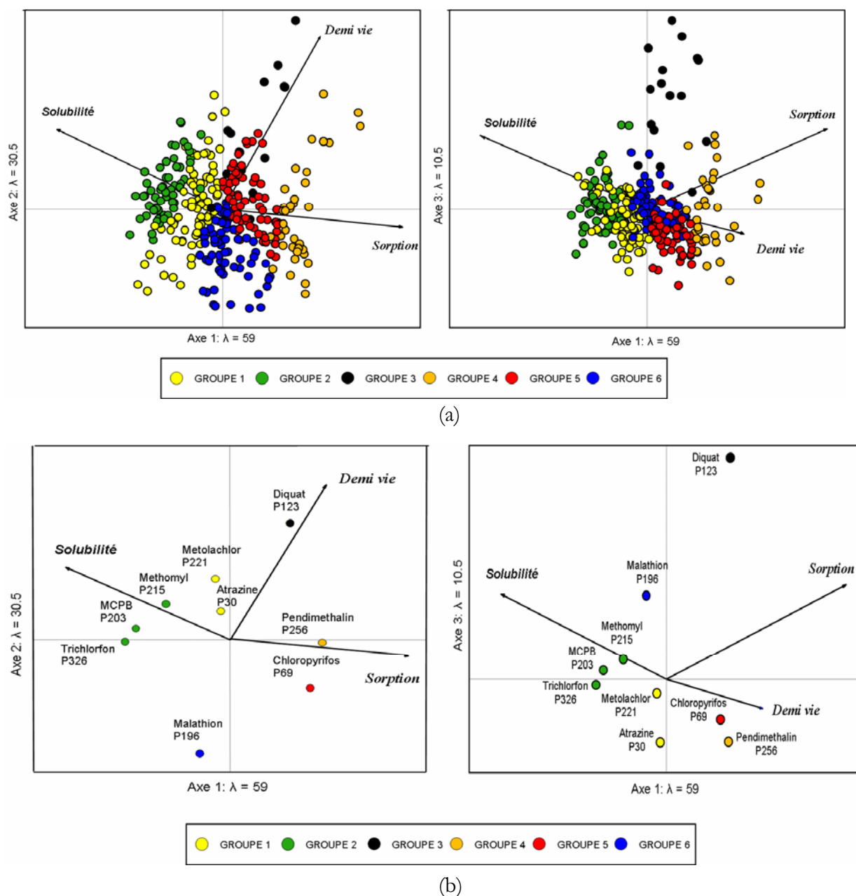
Figure 4.7 : Analyse en Composantes Principales (ACP) illustrant la position des pesticides et des groupes de pesticides en fonction des caractéristiques bio-physico-chimiques. Représentation des 340 pesticides (a) et des composés nominatifs comptant parmi les 10 pesticides « Top ten » d'EC, plus le Métolachlor et le MCPB (b). Les caractéristiques bio-physico-chimiques ont subi une transformation logarithmique afin de réduire l'effet des valeurs extrêmes. Les valeurs propres des trois premiers axes sont les suivantes : \lambda_1 = 59 ; \lambda_2 = 30.5 et \lambda_3 = 10.5 .
