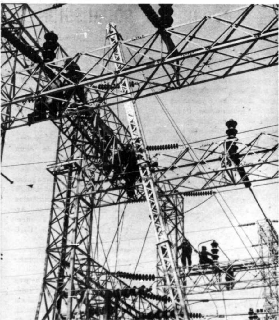
DES HOMMES du service des lignes aux Forces Motrices du Saguenay apportent ici des améliorations au poste de sectionnement de 161 volts Alcan situé près de la centrale d'Isle-Maligne. Un mât en aluminium permet la manutention des pièces d'équipement du sommet jusqu'au sol.
