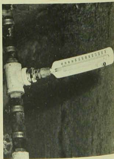
Un thermomètre installé sur le tuyau d'eau, à la sortie du serpent, indique que l'eau a été réchauffée de 10°C (15°F).
