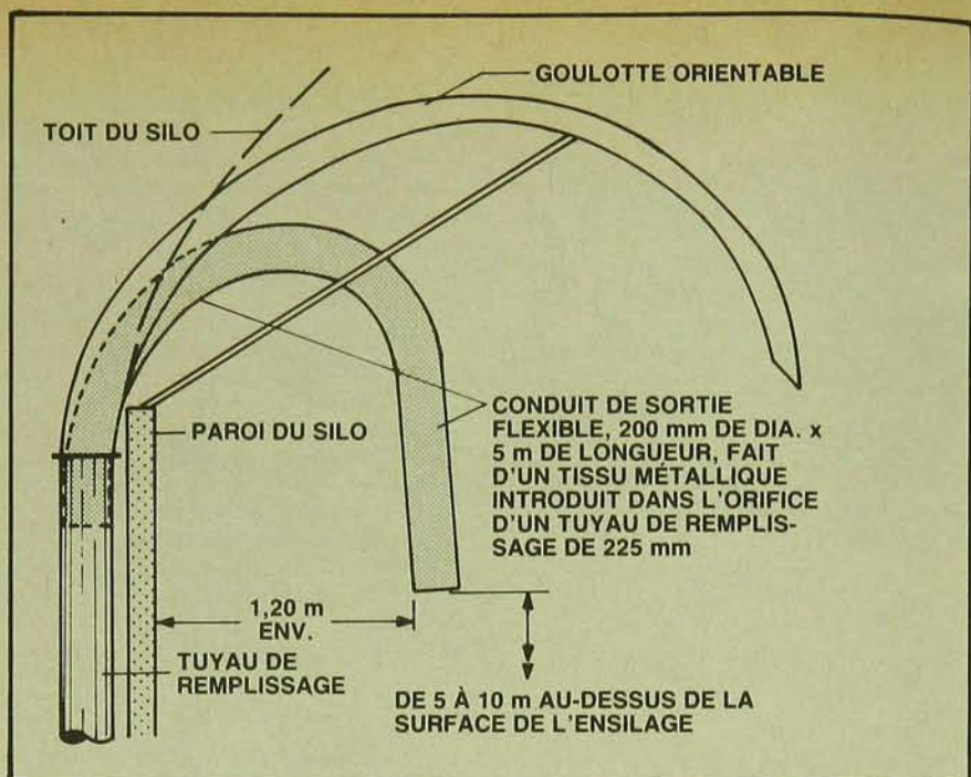
ADAPTEUR D'URGENCE POUR AMÉLIORER LA VENTILATION DE L'ESPACE LIBRE DU SILO AVEC LA SOUFFLERIE À FOURRAGE.
