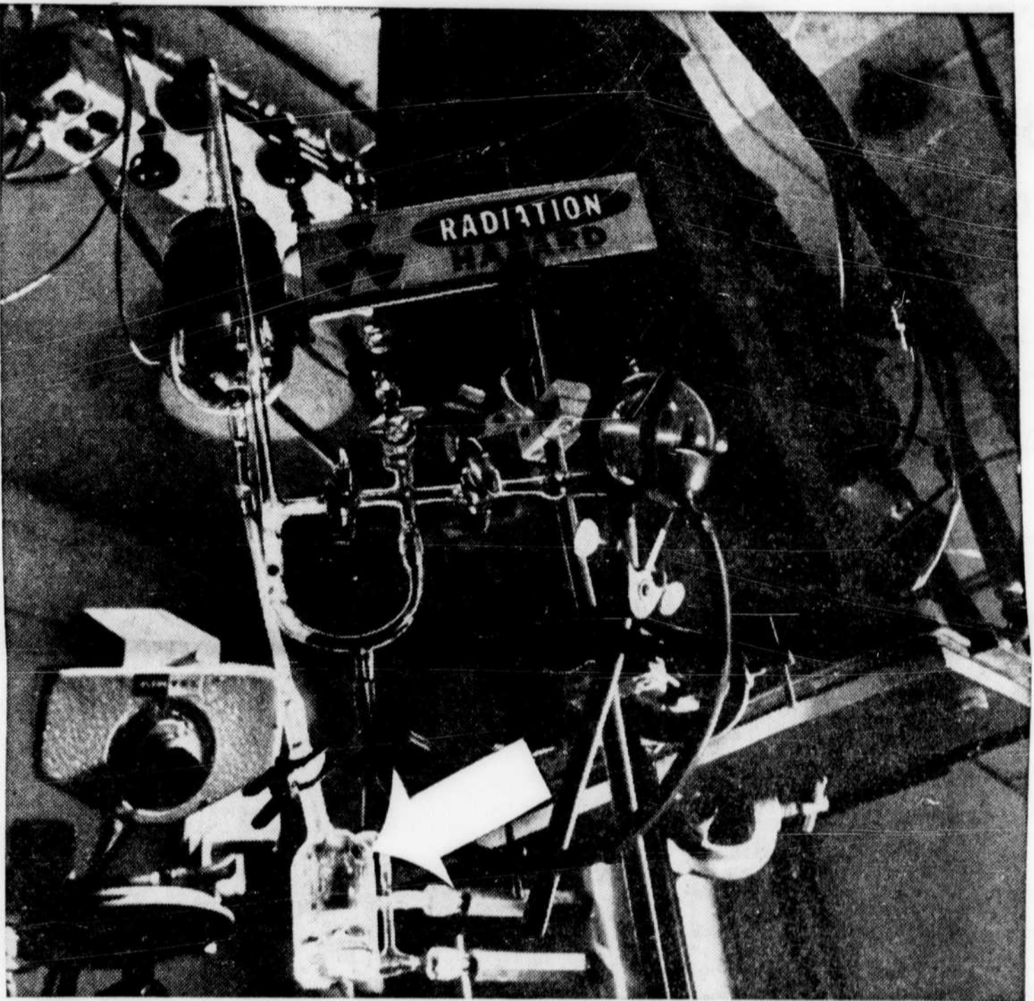
Sous l'oeil vigilant d'une caméra de télévision le mélange de pentanes passe sous un énorme accélérateur Van de Graaf. Un rayon d'électrons à haute intensité pénètre violemment dans une pellicule très mince de pentanes mélangées. Il en résulte des réactions spectaculaires bien qu'invisibles. L'analyse de ces réactions par les techniciens des laboratoires Shell fait partie d'un programme continu. Ce programme étudie tant les performances mécaniques du moteur que ses besoins en carburant.
