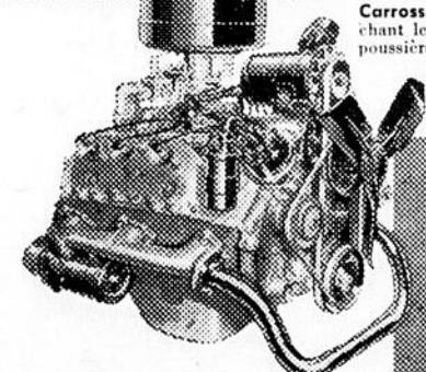
Moteur V-8 "Strato-Star" de 110 CV à haute compression. Construction perfectionnée reposant sur l'expérience acquise en fabriquant plus de moteurs V-8 que tous les autres constructeurs réunis.
