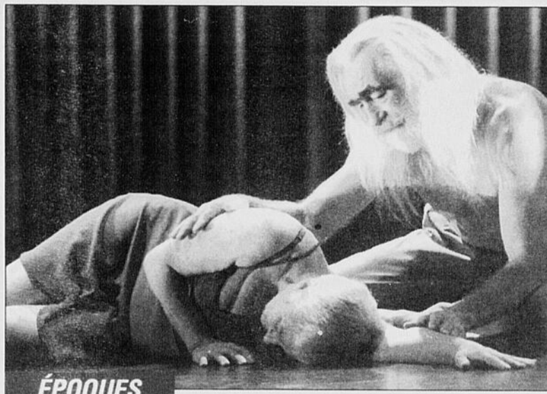
CONTRASTE
