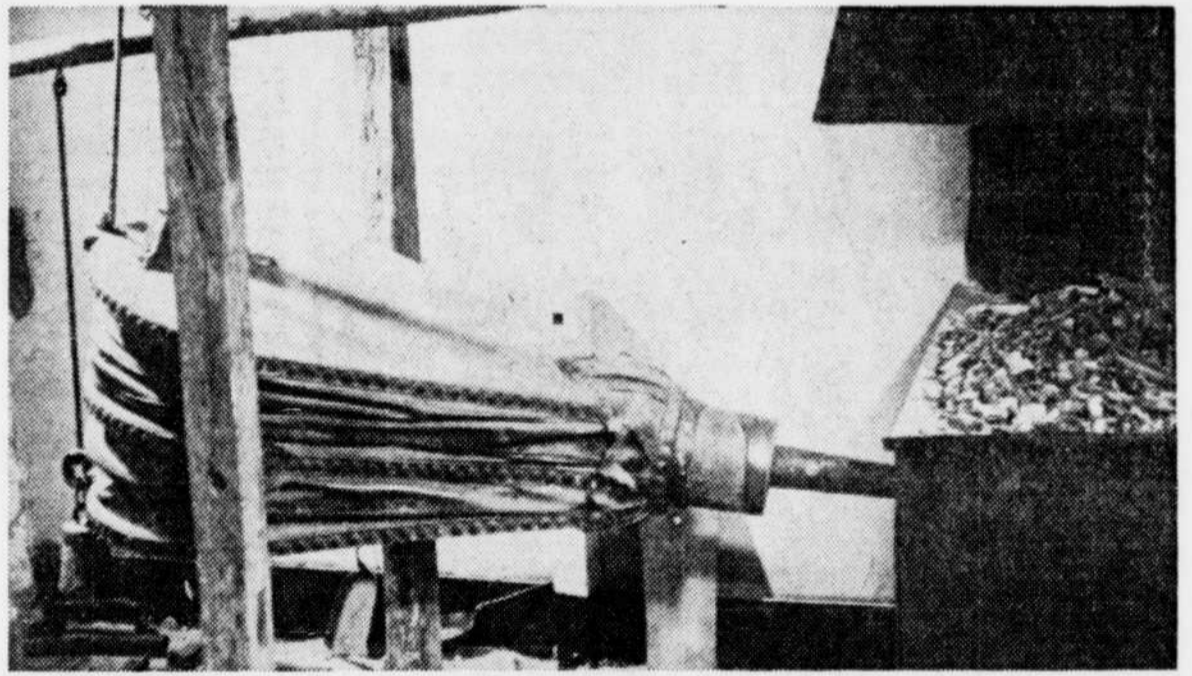
Un foyer de forge et son soufflet conservés au Fourneau Saint-Michel dans les Ardennes.
