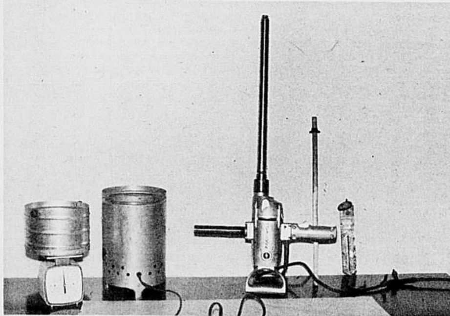
Les accessoires servant à évaluer le degré d'humidité du foin. De gauche à droite: une balance, l'appareil à sécher le foin, la sonde, le bâtonnet pour pousser le foin hors de la sonde et un échantillon de foin séché.
