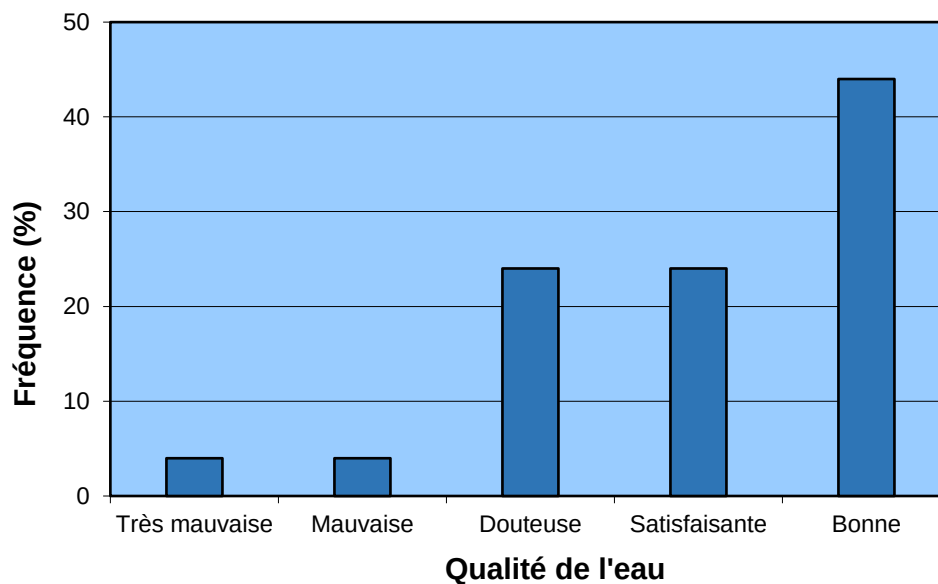
FIGURE 5 QUALITÉ DE L'EAU (IQBP 6 ) DES 25 BASSINS VERSANTS UTILISÉS POUR LA VALIDATION, PÉRIODE 2009-2012
