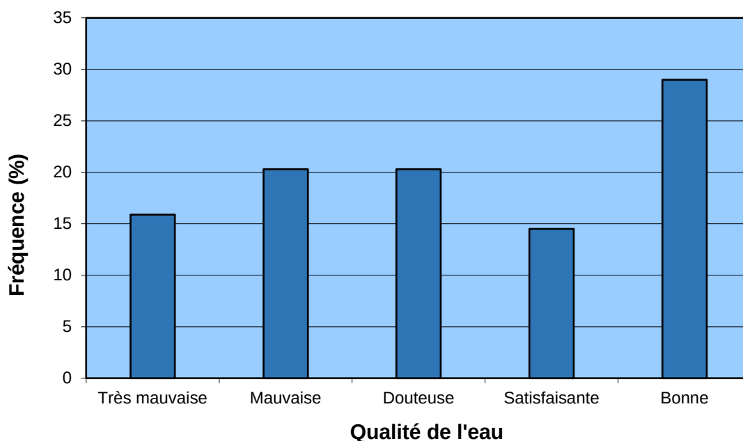
FIGURE 3 QUALITÉ DE L'EAU (IQBP 6 ) DES 69 BASSINS VERSANTS SÉLECTIONNÉS POUR LA MODÉLISATION, PÉRIODE 2009-2012
