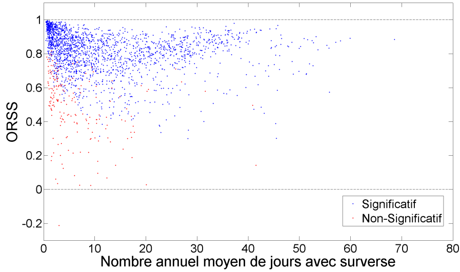
Figure 5.6: Valeurs du ORSS aux différents ODS en fonction du nombre annuel moyen de jours avec surverses pour les cas où m \geq 1 . Les durées maximisant les valeurs du ORSS à chaque ODS sont considérées.
