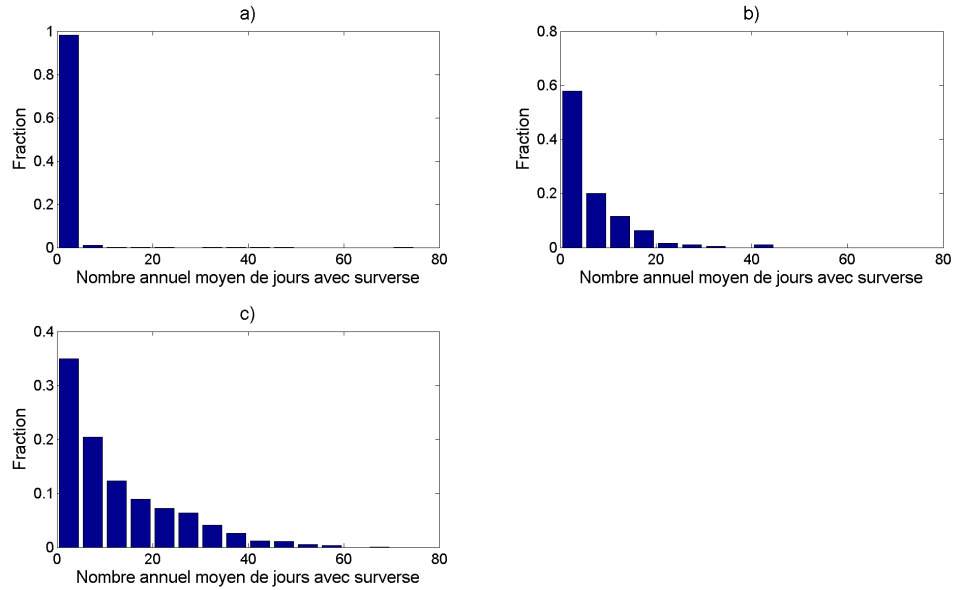
Figure 5.2: Histogrammes du nombre annuel moyen de jour avec surverse aux différents ODS pour les cas où : (a) 0 \geq m < 1 ; (b) m \geq 1 et pouvoir prévisionnel non significatif à 99% ; et (c) m \geq 1 et pouvoir prévisionnel significatif à 99%.
