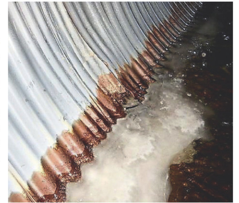
La corrosion du ponceau est l'un des éléments cité dans le rapport d'inspection pour justifier la fermeture de la route.
