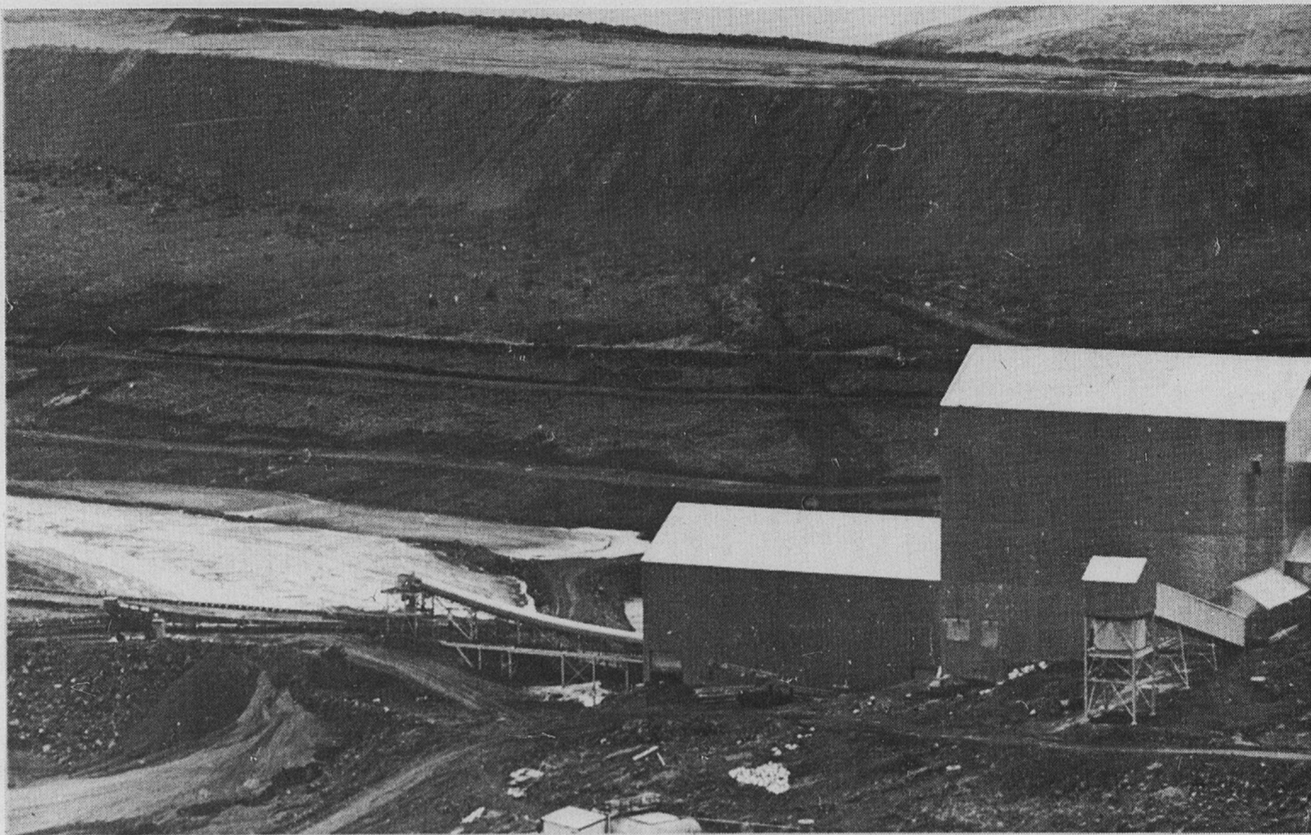
L'usine de concassage largement automatisée de la mine. Dans le fond se dessinent les montagnes de Maluti au sommet desquelles est installée la mine.
