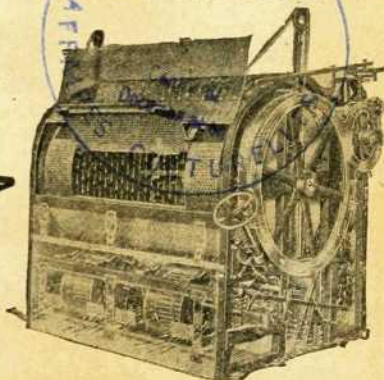
Séchoir Rotatif Secoueur
