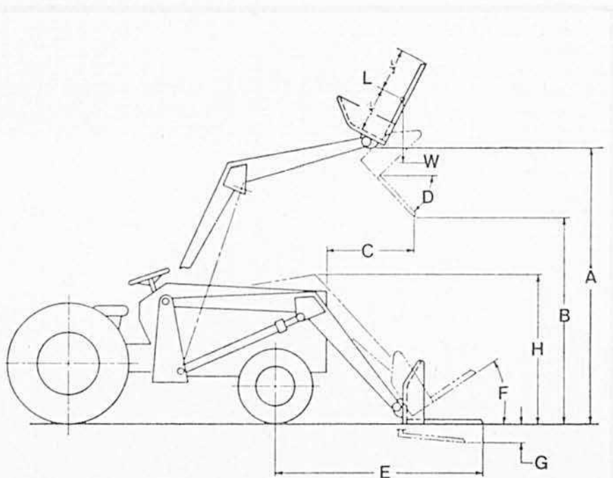
Principales cotes d'un chargeur frontal (Normes ASAE, S301)
