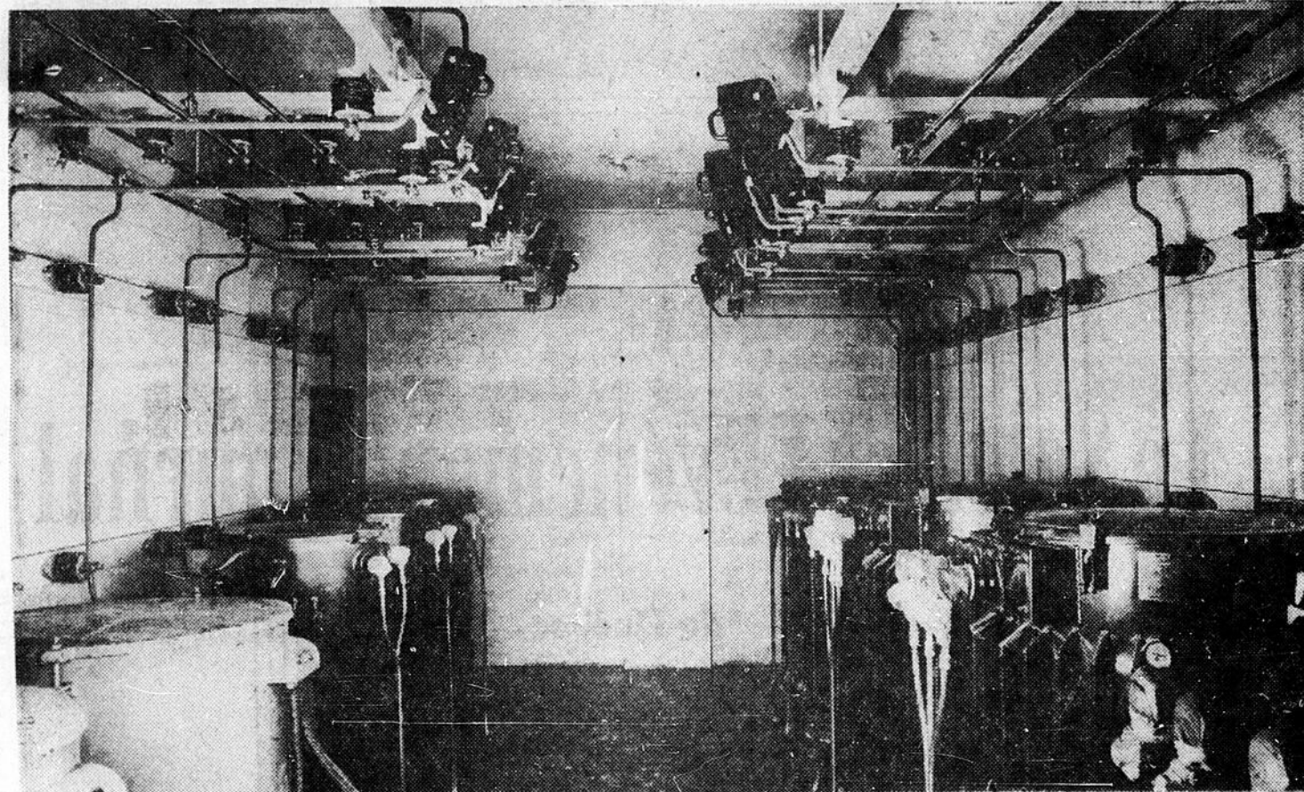
L'installation électrique.
