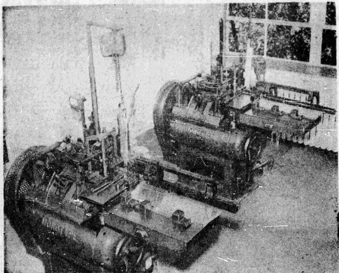
Ces appareils, appelés monotypes, fabriquent les lisières de plomb employées pour séparer les colonnes dans les formes à journal, etc. Elles consomment à elles seules quelque 5,000 livres de plomb par semaine.
