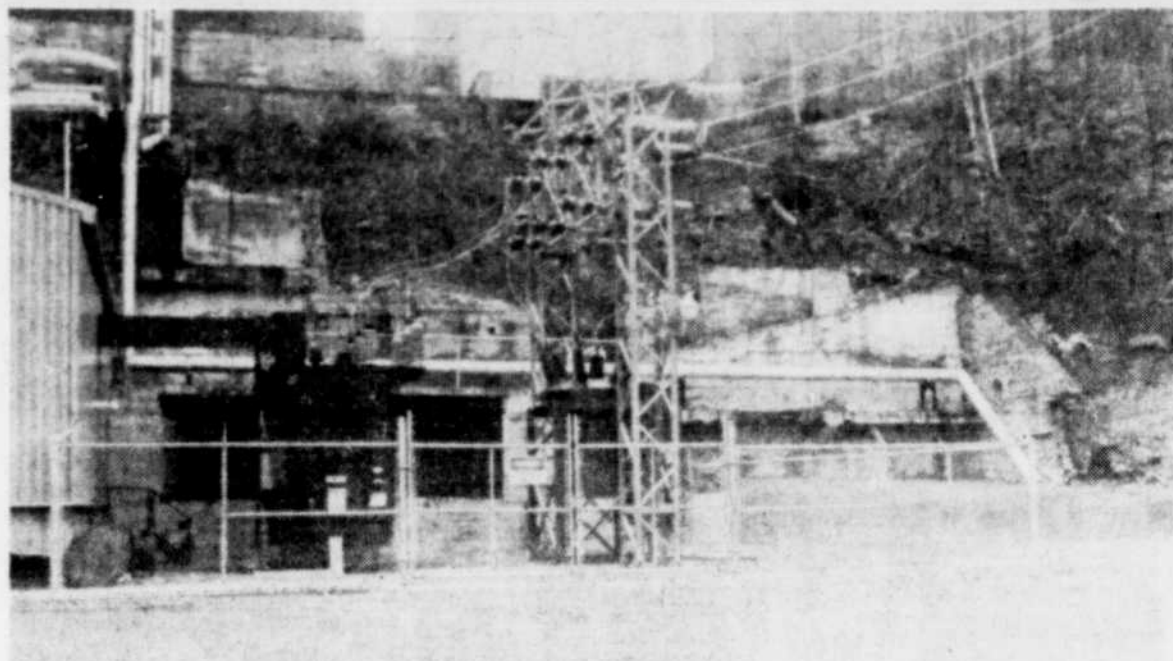
Point d'arrivée de la ligne de 69,000 volts construite spécialement pour alimenter la nouvelle chaudière électrique de l'usine.
