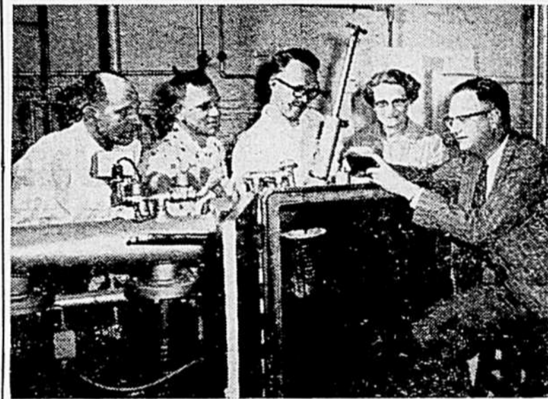
Des professeurs dans les écoles secondaires du Québec et des Maritimes examinent une installation de fusion par induction et moulage sous vide à l'École de génie chimique et métallurgique de l'Université Cornell. Le professeur Julian C. Smith explique que l'installation enlève les impuretés des métaux en chauffant ces derniers, sous vide, à des températures aussi élevées que 3,200°F. Les professeurs sont, de gauche à droite, J.-A. Flemming, St. John High School, Nouveau-Brunswick; le Révérend Père Albert Anctil, Collège de Ste-Anne de la Pocatière, Québec; Norman Chadwick, Pictou Academy, Nouvelle-Ecosse et Mlle Lena Reinhardt, West Kings District High School, Aylesford, Nouvelle-Ecosse. Ils sont au nombre de six professeurs de l'Est du Canada qui suivent à l'Université Cornell, grâce à une bourse pour mérite Shell, un cours d'été de six semaines commandité par la Shell Oil Company of Canada, Limited. Le programme de bourses pour mérite Shell est conçu pour aider les professeurs remarquables de chimie, de physique et de mathématiques dans les écoles secondaires à être au courant des derniers perfectionnements dans leur domaine respectif et dans les méthodes d'enseignement. Des cours semblables sont donnés aux professeurs de l'Ouest du Canada à l'Université Stan-
