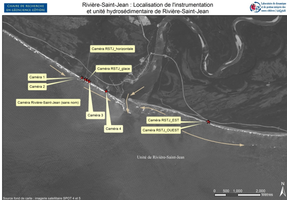
Figure 11 Localisation de l'instrumentation sur les sites de Rivière-Saint-Jean
