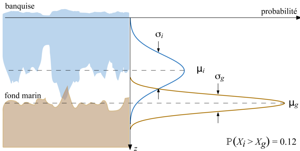
Figure 85 Schéma de la méthode de calcul de la probabilité de contact entre la glace et le fond à partir des densités de probabilité suivant des lois normales. Dans cet exemple, la probabilité que x_i soit plus grande que x_g est non nulle et, une fois calculée, la probabilité de contact entre la glace et le fond s'élève à 12 %, que l'on interprète comme la portion de la surface du couvert de glace d'une cellule qui est en contact avec le fond
