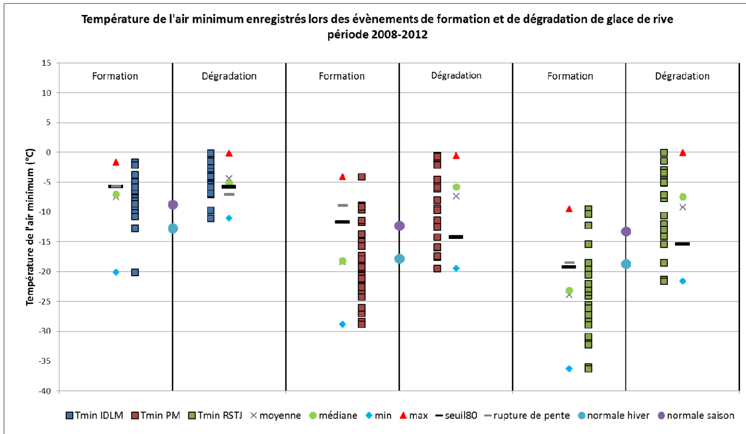
Figure 126 Températures de l'air minimum enregistrées lors des évènements de formation et de dégradation
