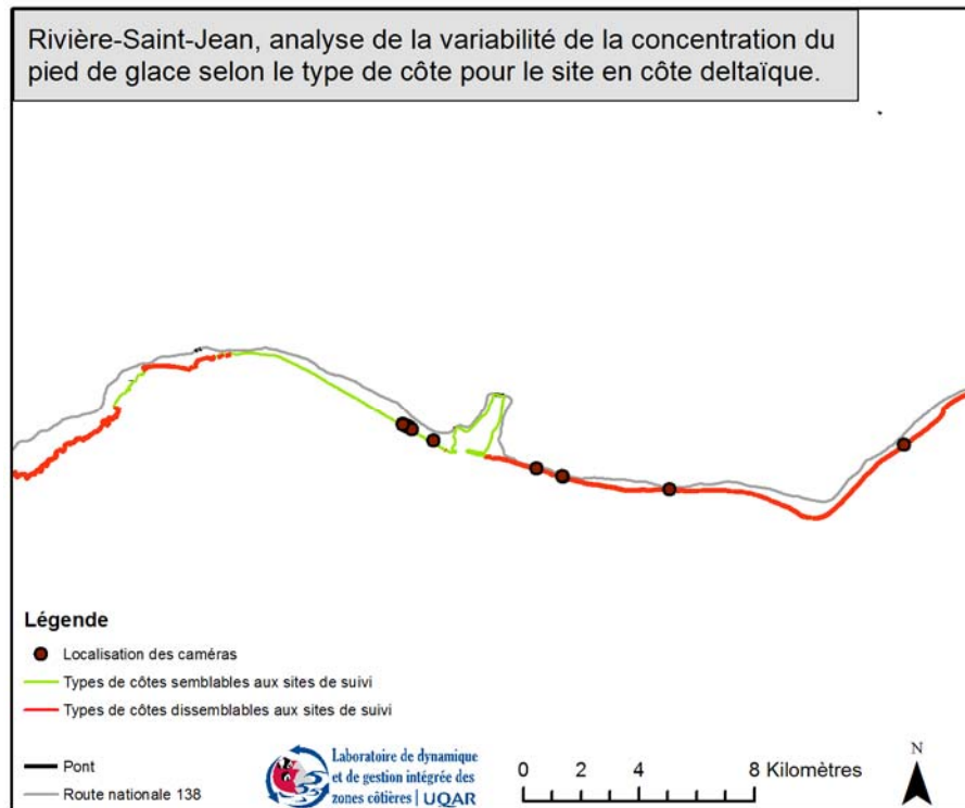
Figure 76 Cartographie de l'analyse de la variabilité spatiale du pied de glace de la région de l'embouchure de la rivière Saint-Jean pour le site situé en côte deltaïque
