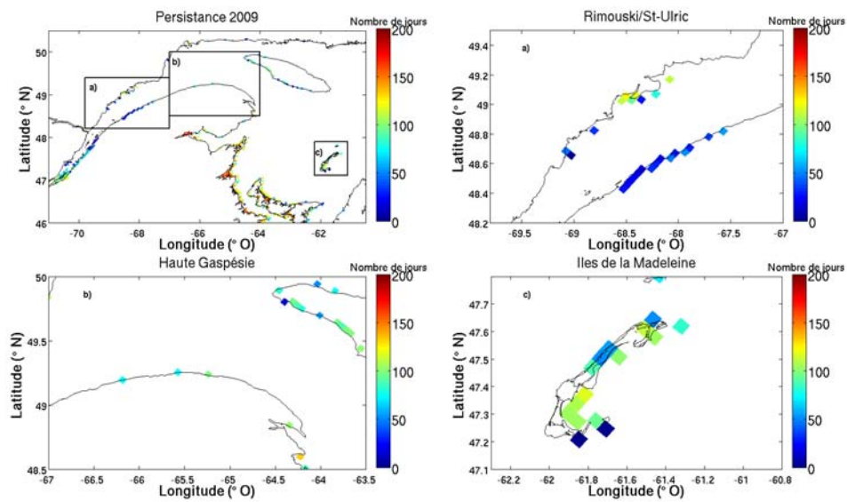
Figure 91 Carte de la persistance du pied de glace en nombre de jours pendant lesquels la contrainte au fond a dépassé 0,1 Pa pour le golfe et l'estuaire (en haut, à gauche) au cours de l'hiver 2008-2009 (agrandissement a, b et c représentant respectivement l'estuaire maritime, la côte nord de la Gaspésie et les îles de la Madeleine)
