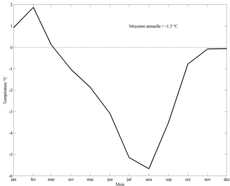
Figure 144 Biais mensuels de température de l'air (MRCC-GEM) moyennés sur l'ensemble du domaine du modèle numérique pour la simulation climatique MRCC-AEV
