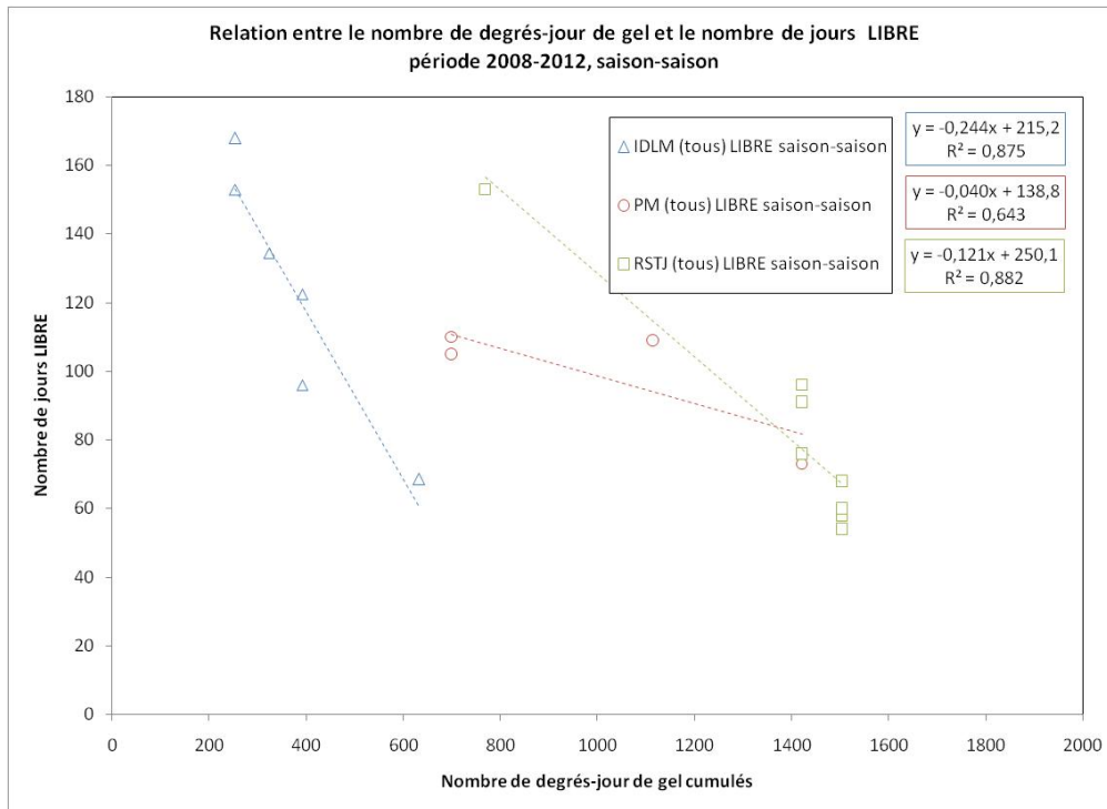
Figure 140 Relation entre le nombre de degrés-jours de gel et le nombre de jours LIBRE durant la saison, période 2008-2012
