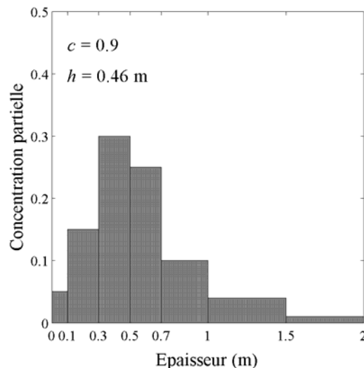
Figure 84 Exemple de distribution d'épaisseur que l'on peut retrouver à un moment donné à un point de la grille du modèle. C'est à partir de cette distribution déterministe g(h) que l'on infère la distribution X_i = N(\mu_i, \sigma_i) de la variable aléatoire x_i
