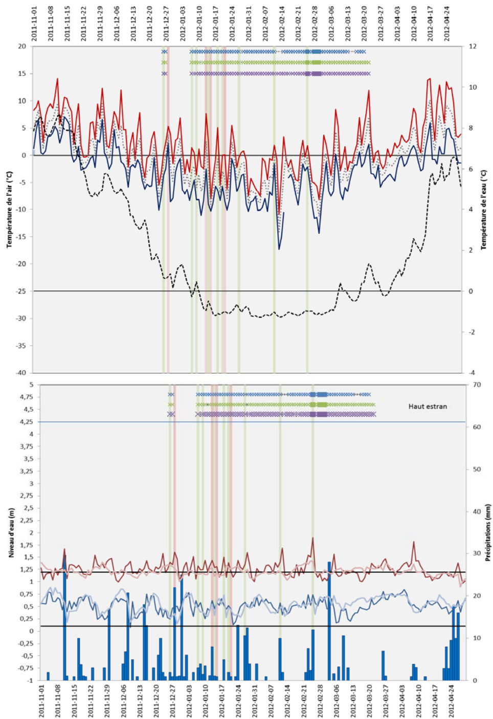
Figure 20 Saison glacielle 2011-2012, La Martinique, Îles-de-la-Madeleine
