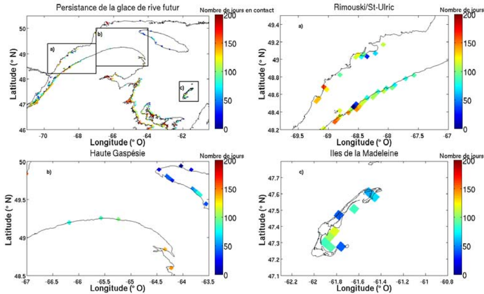
Figure 98 Carte de la persistance moyenne du pied de glace en nombre de jours pendant lesquels la contrainte au fond a dépassé 0,1 Pa pour le golfe et l'estuaire (en haut, à gauche) pour le climat futur (2042-2067) (agrandissement a, b et c représentant respectivement l'estuaire maritime, la côte nord de la Gaspésie et les îles de la Madeleine)
