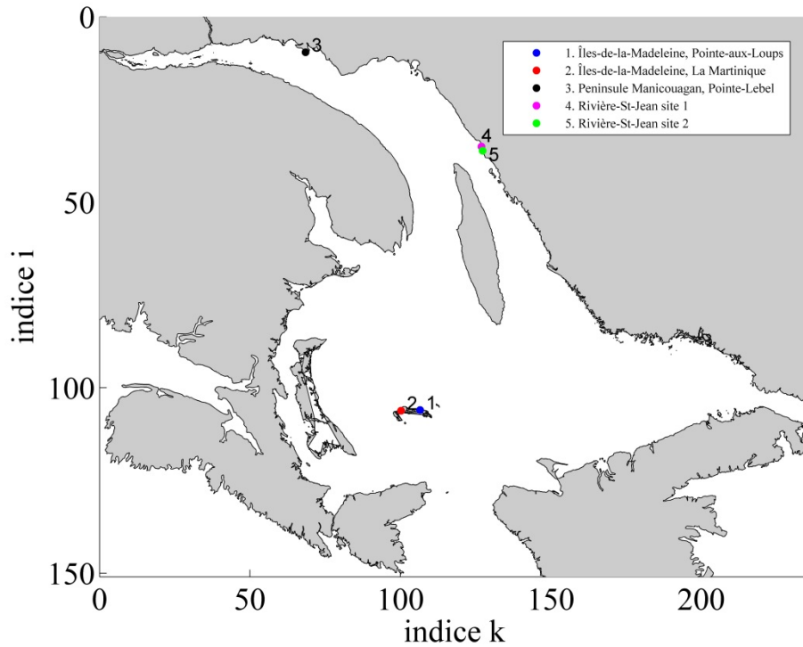
Figure 33 Emplacement des différents sites d'observations
