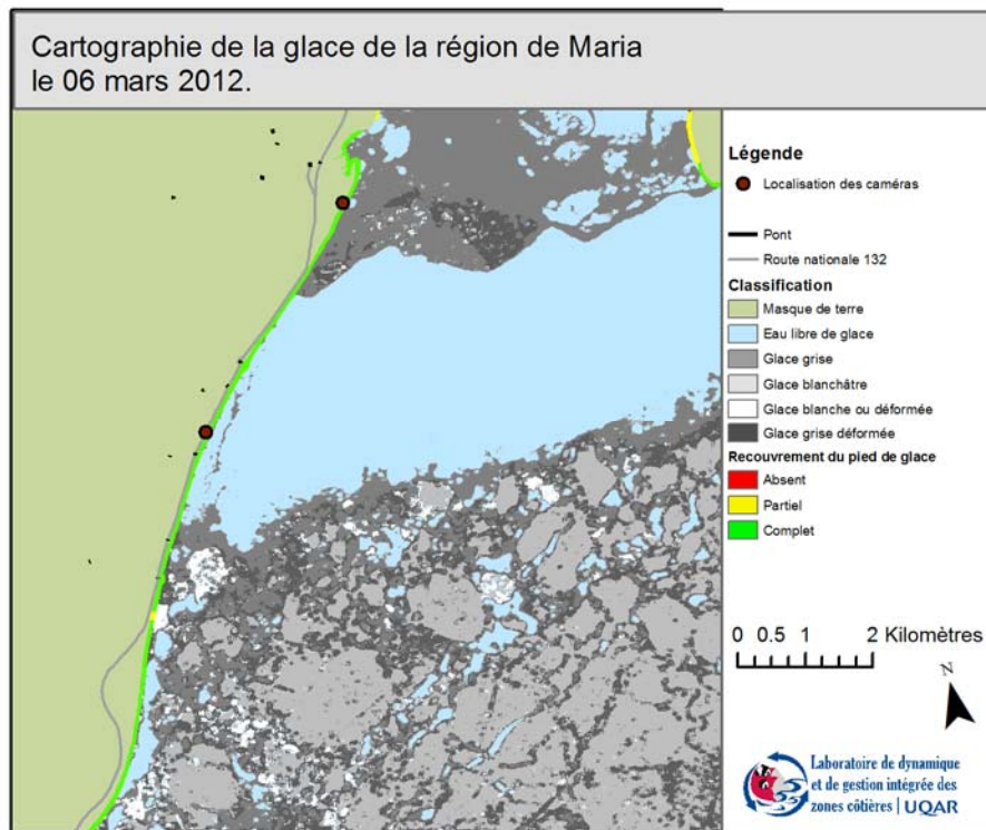
Figure 169 Agrandissement de la cartographie de la glace littorale de la région de l'embouchure de la baie de Maria
