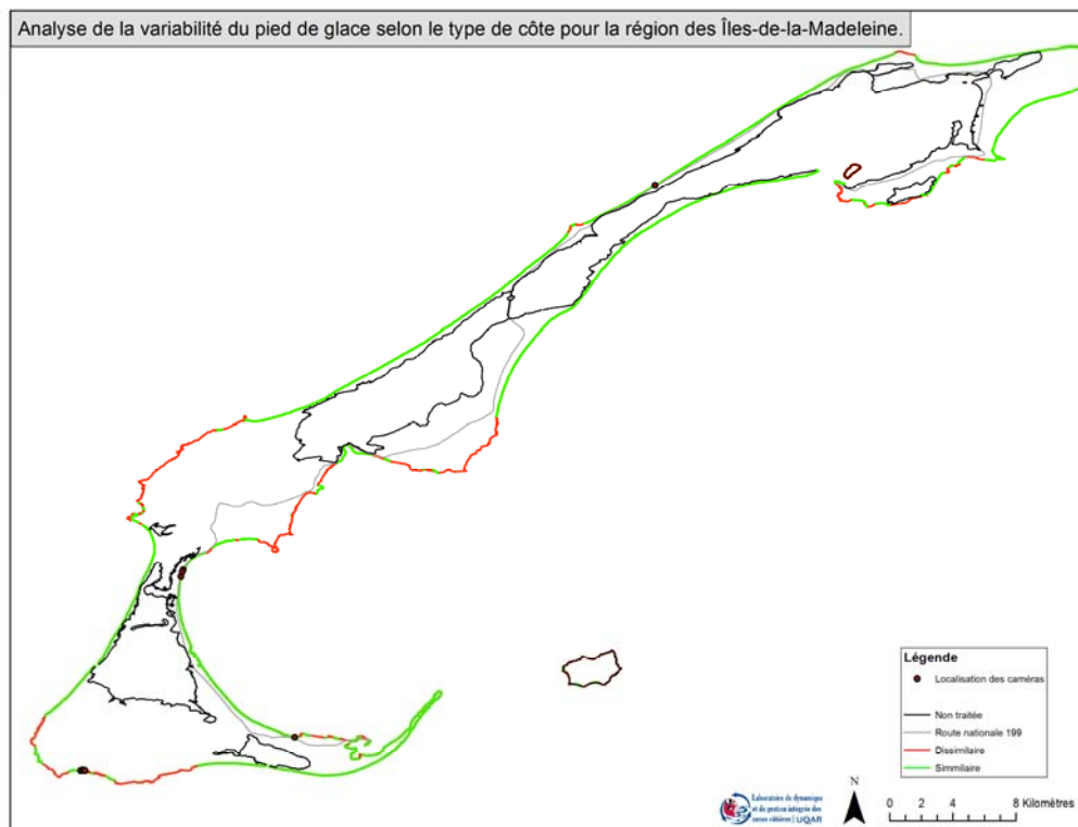
Figure 83 Cartographie de l'analyse de la variabilité spatiale du pied de glace de l'archipel des îles de la Madeleine
