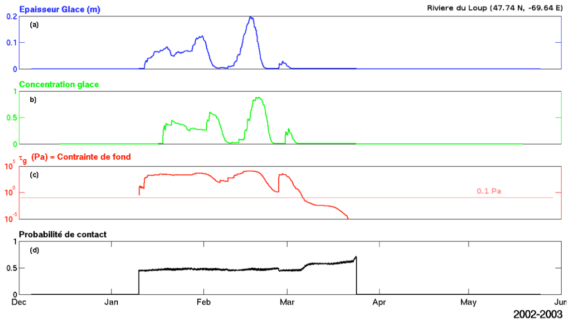
Figure 87 Séries temporelles de a) l'épaisseur, b) la concentration, c) contrainte au fond et d) la probabilité de contact au point de grille (47,74°N, 69,64°O), près de Rivière-du-Loup, pour l'hiver 2002-2003
