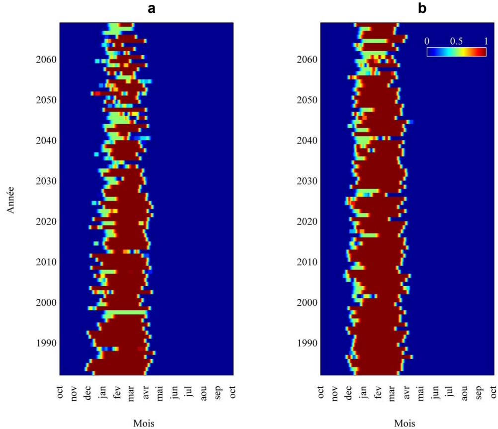
Figure 54 Séries temporelles du PDG à Rivière-Saint-Jean, site 2, pour la simulation MOR-AEV-bTq (a) et la simulation MOR-AHJ (b). Les années sont sur l'axe vertical (de 1981 à 2070), les mois, sur l'axe horizontal, et l'échelle de couleurs représente la fraction de la région couverte par le PDG
