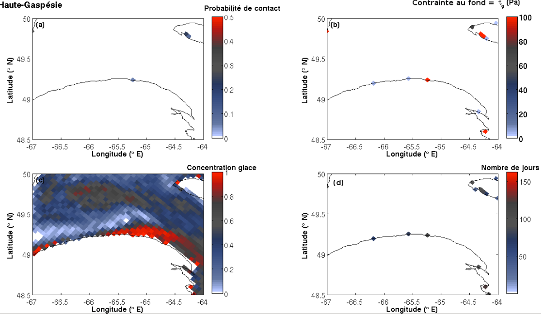
Figure 93 a) Probabilité de contact b) contrainte au fond et c) concentration de glace au 26 février 2003. Le panneau d) indique la persistance en nombre de jours du pied de glace dans l'estuaire maritime au cours de l'hiver 2002-2003 (agrandissement de la Figure 90)
