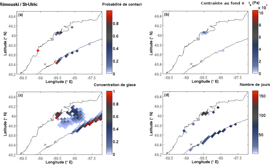
Figure 92 a) Probabilité de contact b) contrainte au fond et c) concentration de glace au 26 février 2003. Le panneau d) indique la persistance en nombre de jours du pied de glace dans l'estuaire maritime au cours de l'hiver 2002-2003 (agrandissement de la Figure 90)
