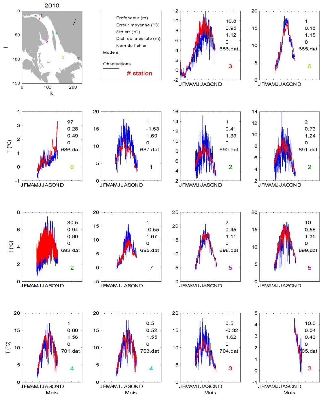
Figure 146 Comparaison entre les résultats du modèle (en rouge) et les observations (en bleu) pour une série de thermographes en 2010. Une carte, en haut à gauche, et l'encadré à sa droite permettent de positionner et d'interpréter les comparaisons
