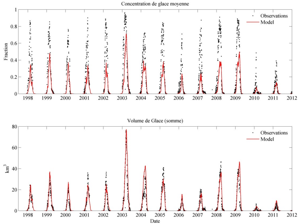
Figure 152 Comparaison de la concentration moyenne et du volume total de glace de mer. Les valeurs tirées du modèle sont en rouge et les observations obtenues des cartes de glace sont en noir
