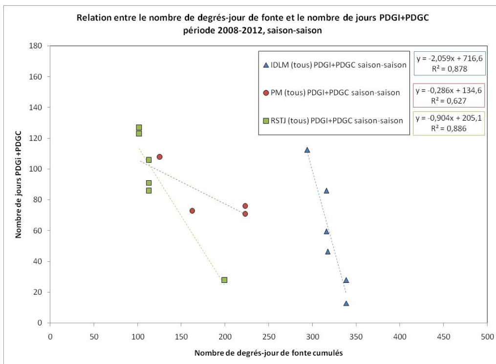
Figure 143 Relation entre le nombre de degrés-jours de fonte et le nombre de jours PDGI+PDGC durant la saison, période 2008-2012
