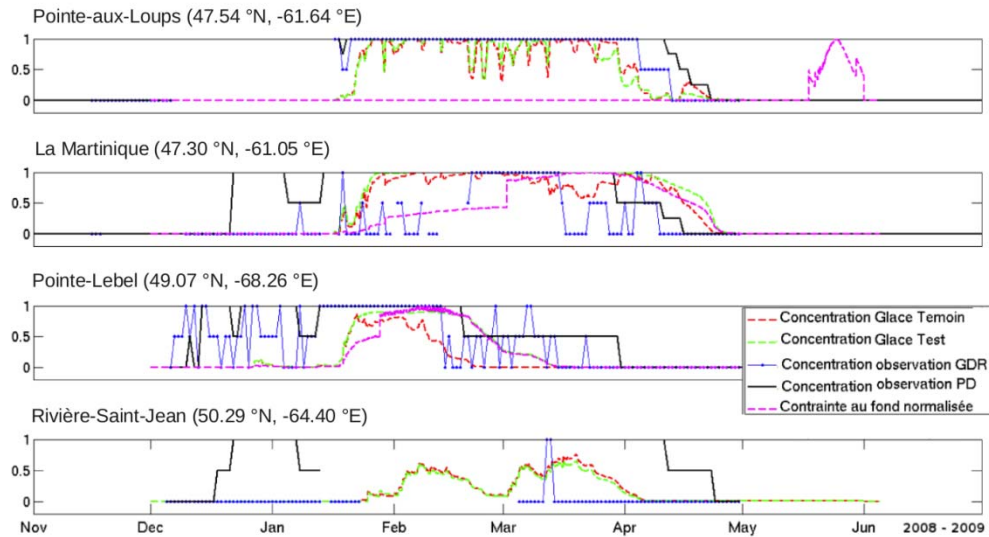
Figure 95 Comparaison entre la simulation témoin (concentration), la simulation test (concentration et contrainte au fond normalisée) et les observations du pied de glace (PDG) pour les quatre sites d'intérêt, Pointe-aux-Loups, La Martinique, Pointe-Lebel et Rivière - Saint-Jean (les concentrations sont exprimées de 0 à 1, signifiant de l'absence jusqu'au couvert total de glace)
