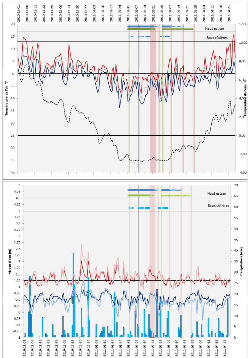
Figure 19 Saison glacielle 2010-2011, Pointe-aux-Loups, Îles-de-la-Madeleine
