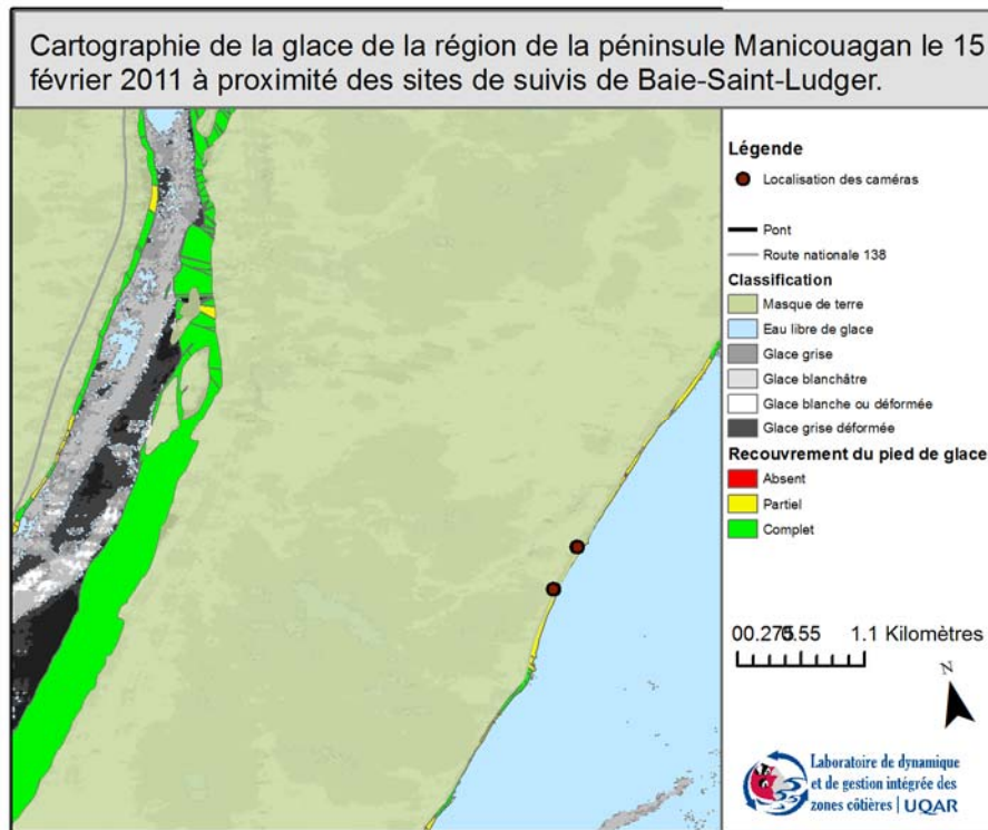
Figure 160 Agrandissement de la cartographie de la glace littorale de la région de la péninsule Manicouagan centrée sur le site de Baie-Saint-Ludger
