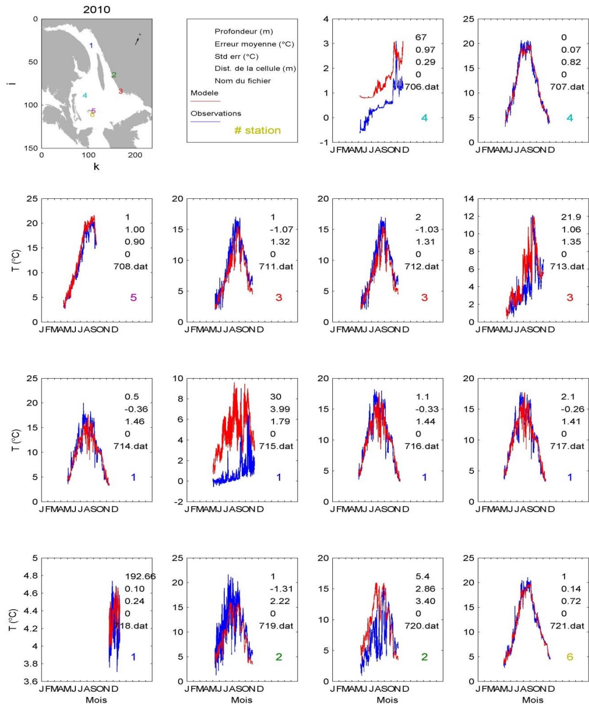
Figure 147 Comparaison entre les résultats du modèle (en rouge) et les observations (en bleu) pour une série de thermographes en 2010. Une carte, en haut à gauche, et l'encadré à sa droite permettent de positionner et d'interpréter les comparaisons
