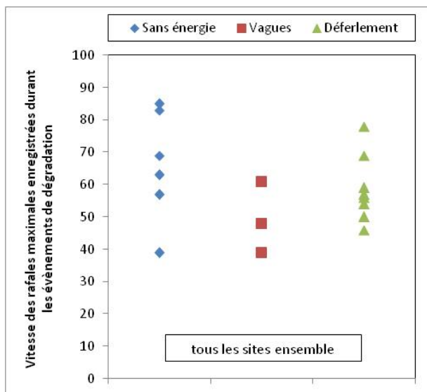
Figure 121 Vitesse des rafales maximales enregistrées lors des évènements de dégradation post-PDGC lorsque les vents soufflaient vers la côte selon le niveau d'énergie déployée contre la glace
