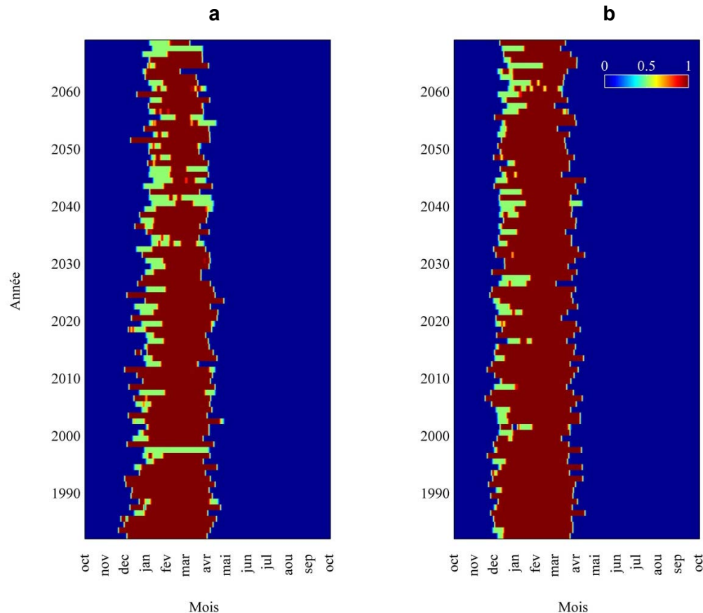
Figure 52 Séries temporelles du PDG à Rivière-Saint-Jean, site 1, pour la simulation MOR-AEV-bTq (a) et la simulation MOR-AHJ (b). Les années sont sur l'axe vertical (de 1981 à 2070), les mois, sur l'axe horizontal, et l'échelle de couleurs représente la fraction de la région couverte par le PDG
