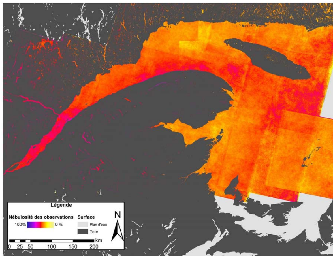
Figure 63 Répartition spatiale de la nébulosité, f_{\text{nuage}} , pour l'EGSL pour la période hivernale de 1996 à 2012
