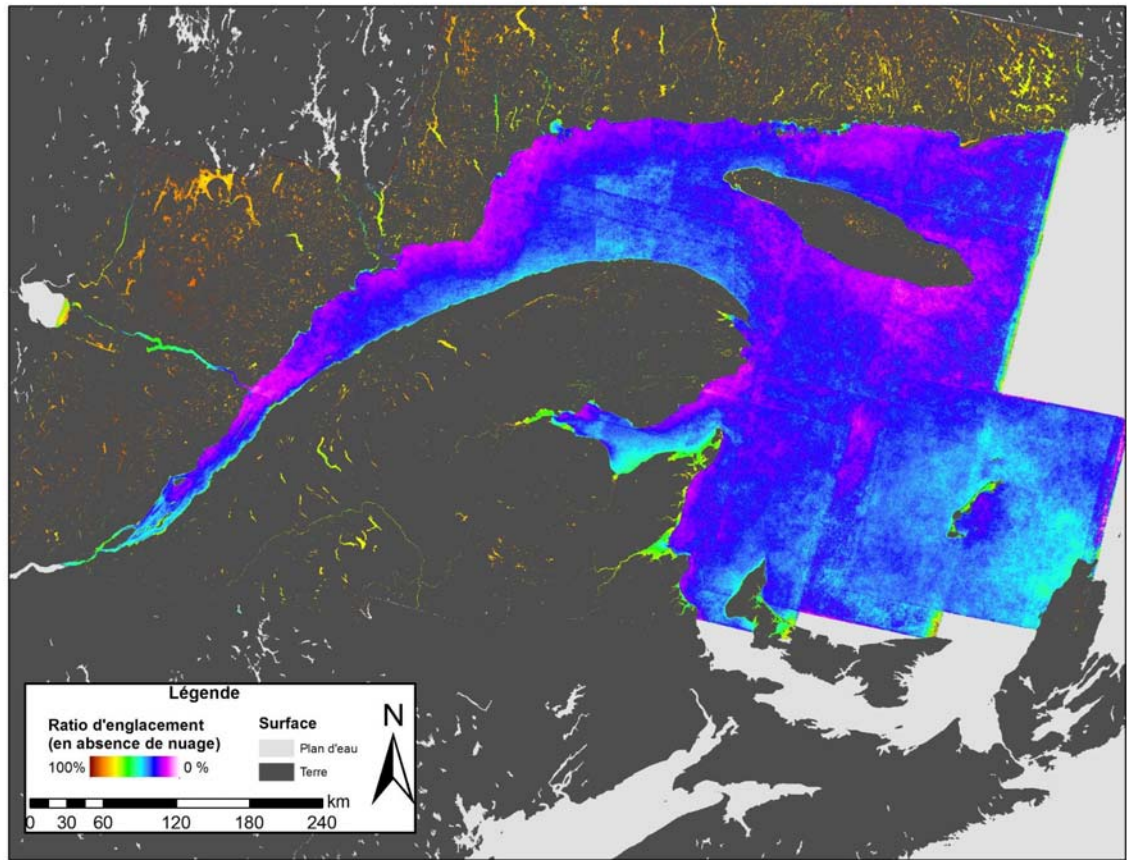
Figure 64 Ratio d'englacement, f_{\text{glace}} , pour l'ensemble de l'EGSL calculé à partir des données hivernales de Landsat, de 1996 à 2012 (voir A3.2 pour plus de détails)
