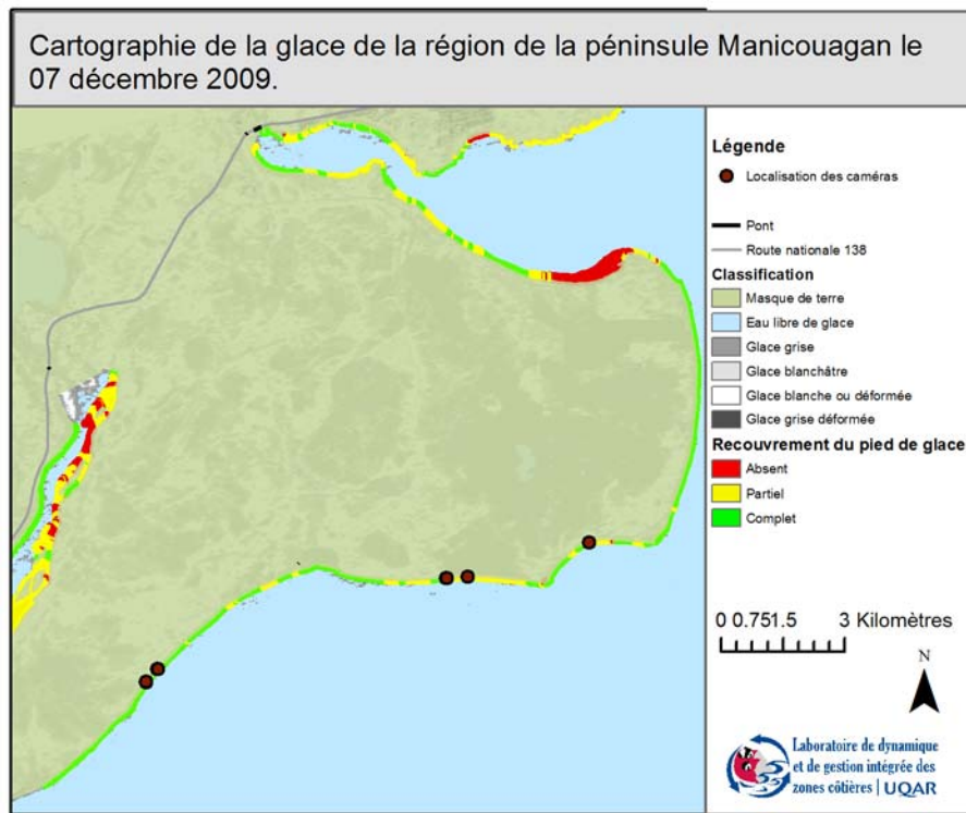
Figure 161 Cartographie de la glace littorale de la région de la péninsule de Manicouagan, le 7 décembre 2009
