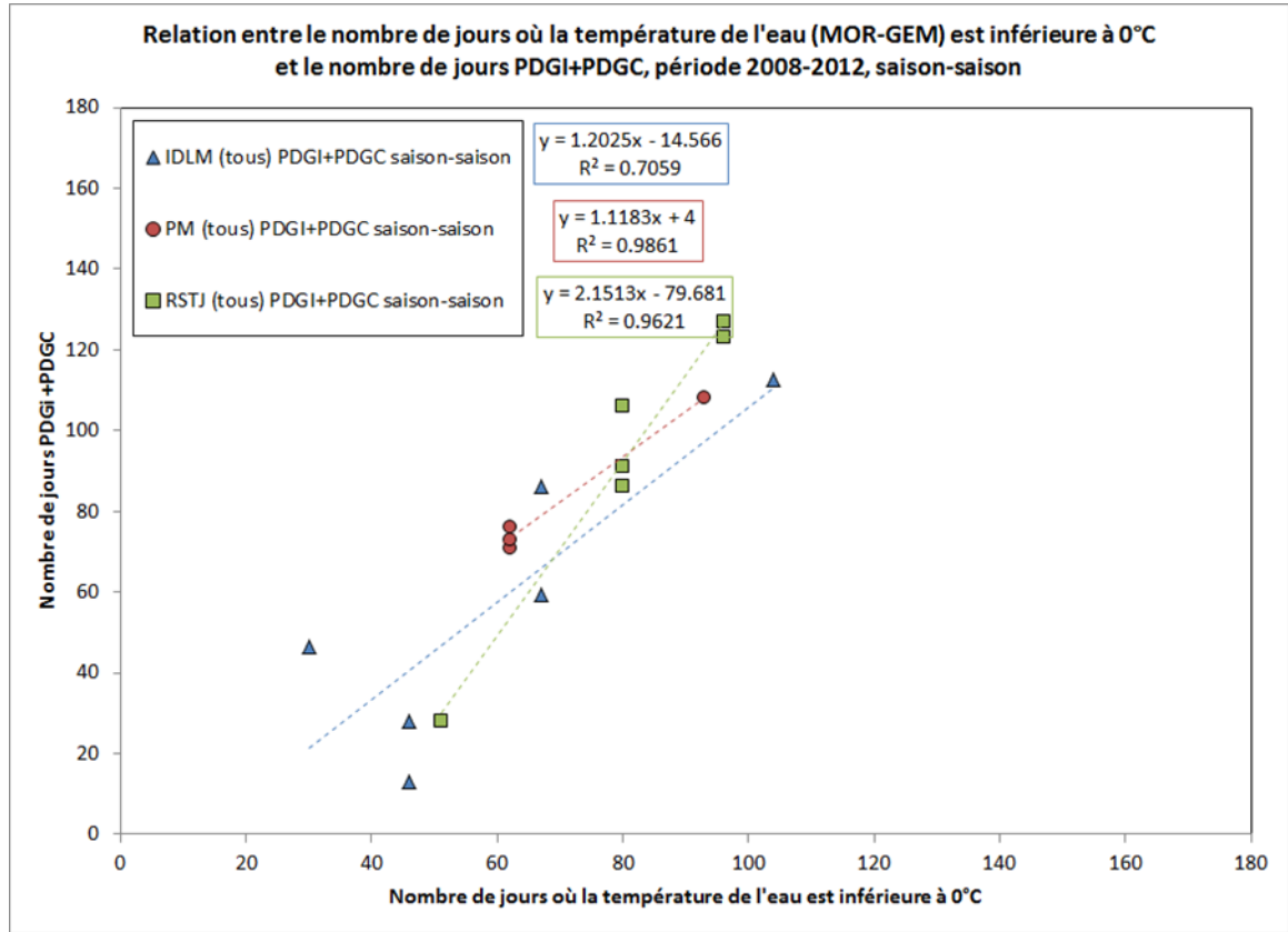
Figure 133 Relation entre le nombre de jours où la température de l'eau est inférieure à 0 °C et le nombre de jours PDGI+PDGC
