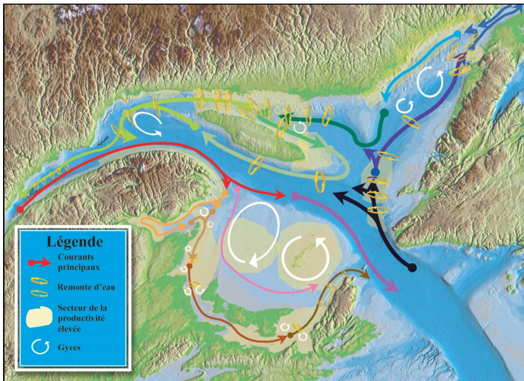
Figure 129 Représentation des courants et des remontées d'eau dans l'estuaire et dans le golfe du Saint-Laurent
