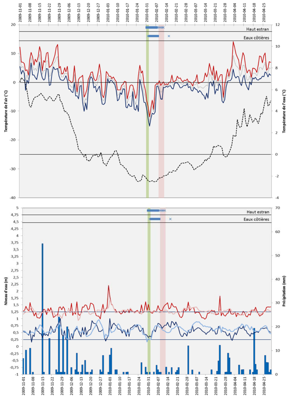
Figure 18 Saison glacielle 2009-2010, Pointe-aux-Loups, Îles-de-la-Madeleine
