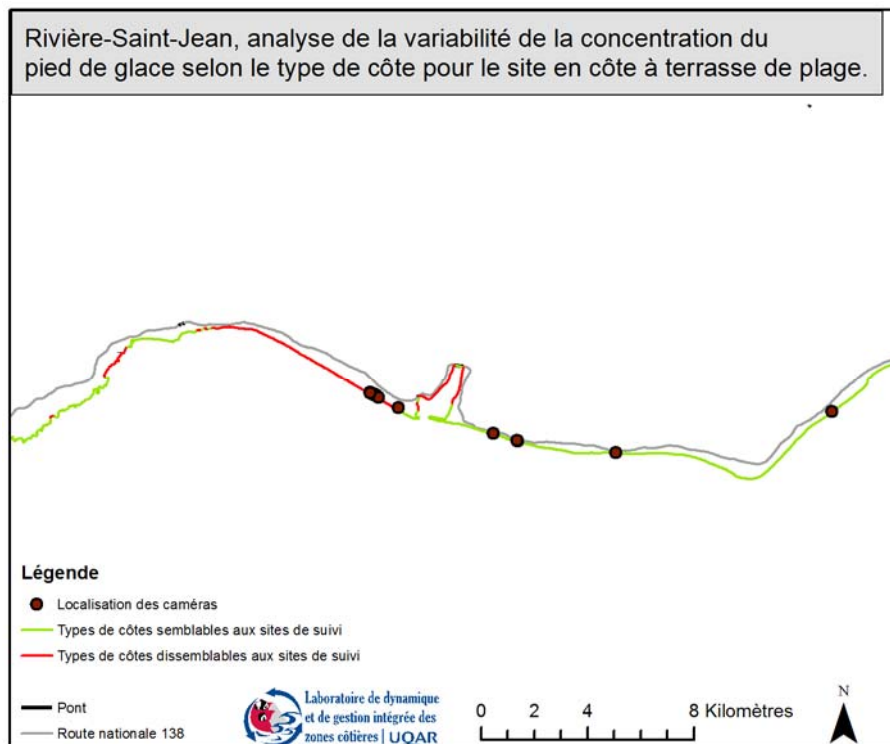
Figure 77 Cartographie de l'analyse de la variabilité spatiale du pied de glace de la région de l'embouchure de la rivière Saint-Jean pour le site situé en côte à terrasse de plage
