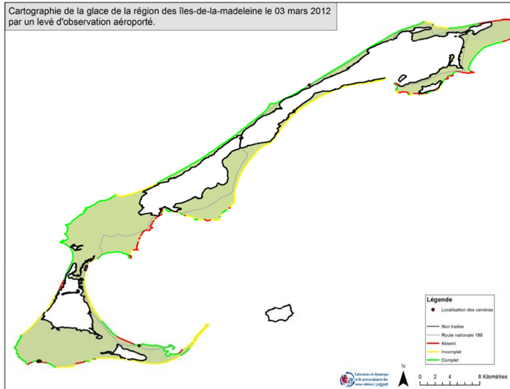
Figure 82 Cartographie du pied de glace estimé à partir des photographies aériennes acquises à basse altitude le 3 mars 2012
