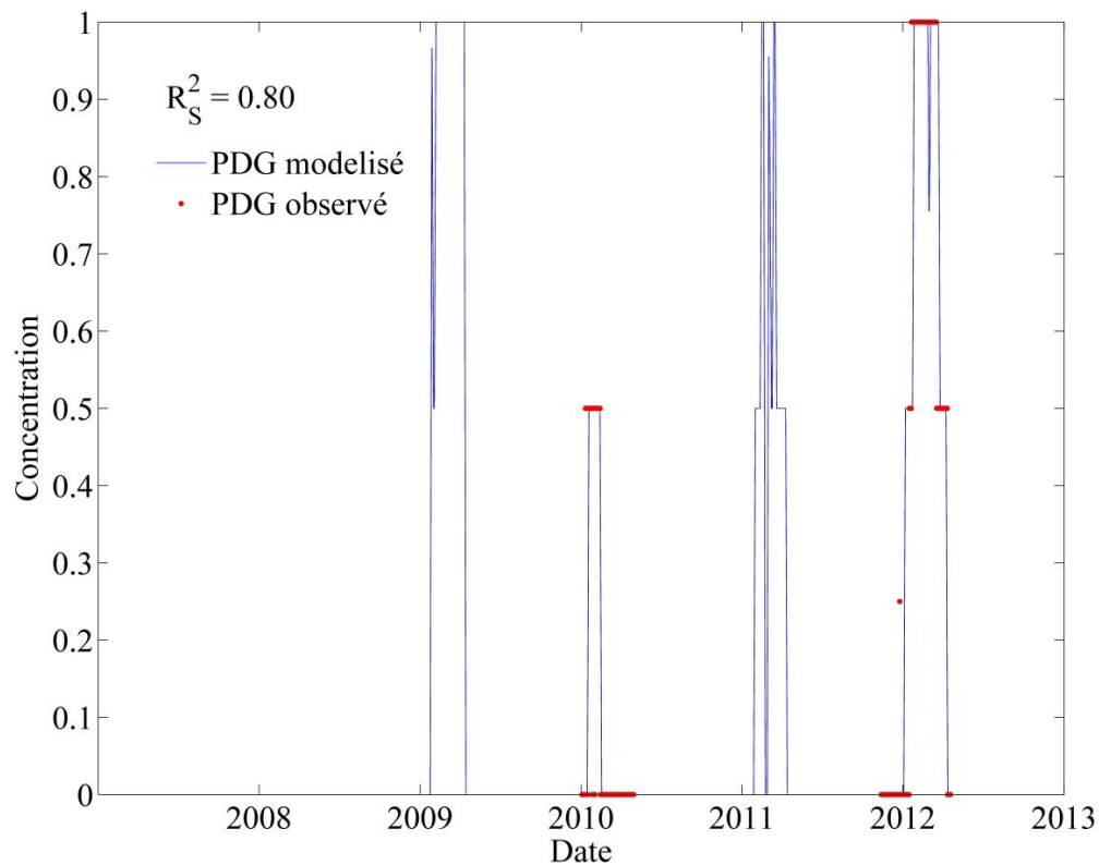
Figure 44 Série temporelle (2008-2013) du pied de glace à Rivière-Saint-Jean, site 1. Les observations semi-quantitatives (0=absence, 0,5=présence et 1=couvert complet) sont en rouge et le résultat de la relation empirique est en bleu. Comme plusieurs stations adjacentes sont moyennées, des valeurs intermédiaires pour les observations sont indiquées. Le coefficient de corrélation de Spearman ( R_s^2 ) est indiqué dans le coin supérieur gauche de la figure
