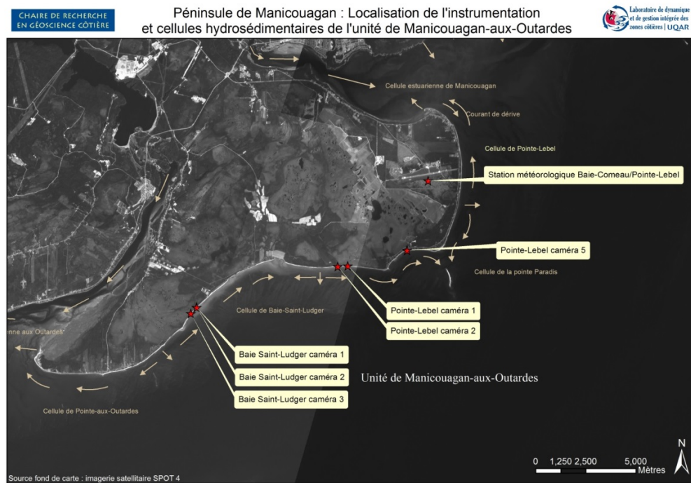
Figure 10 Localisation de l'instrumentation sur les sites de la péninsule de Manicouagan
