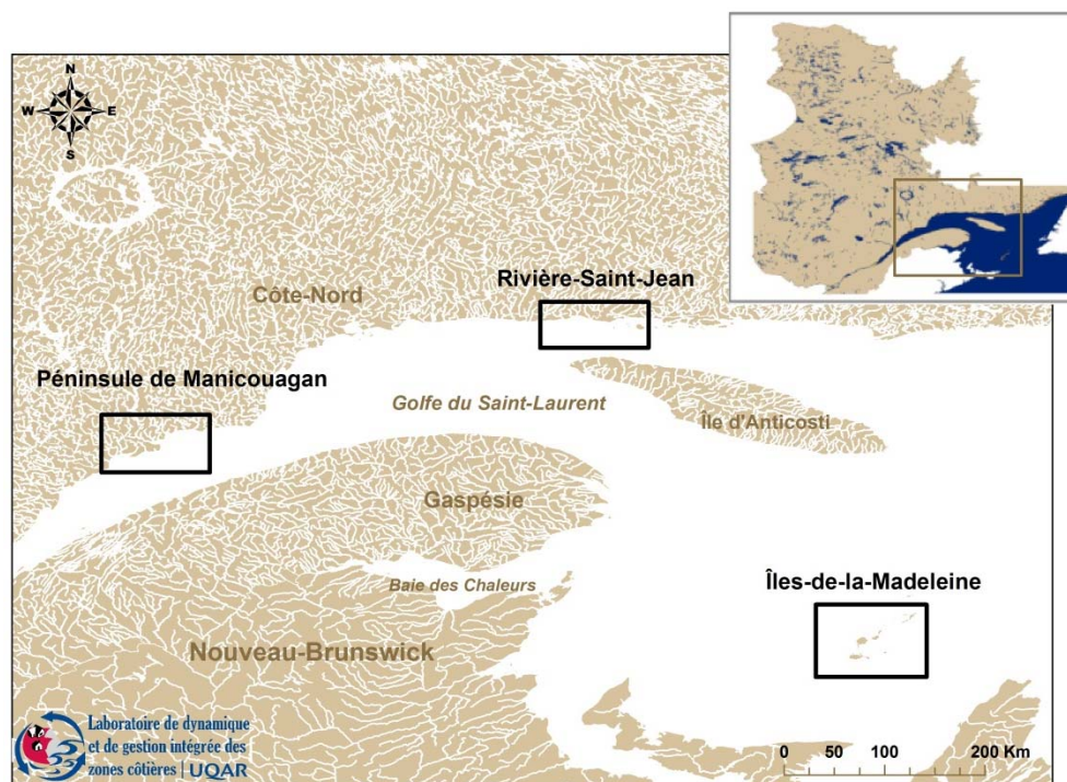
Figure 7 Localisation générale des sites d'étude : Îles-de-la-Madeleine, péninsule de Manicouagan et Rivière-Saint-Jean
