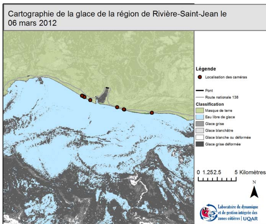
Figure 163 Cartographie de la glace littorale de la région de l'embouchure de la rivière Saint-Jean
