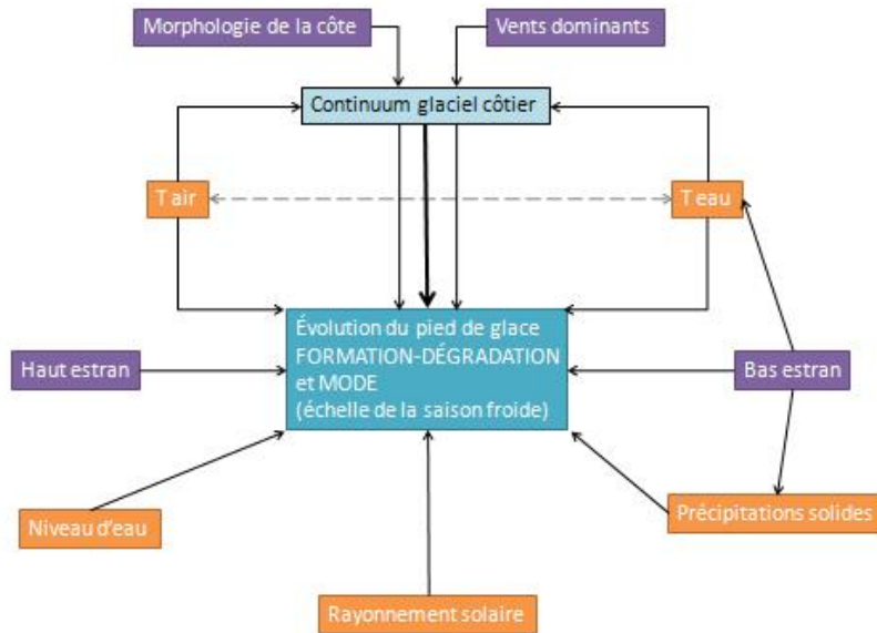
Figure 31 Modèle conceptuel des paramètres influençant l'évolution de l'englacement du haut estran
