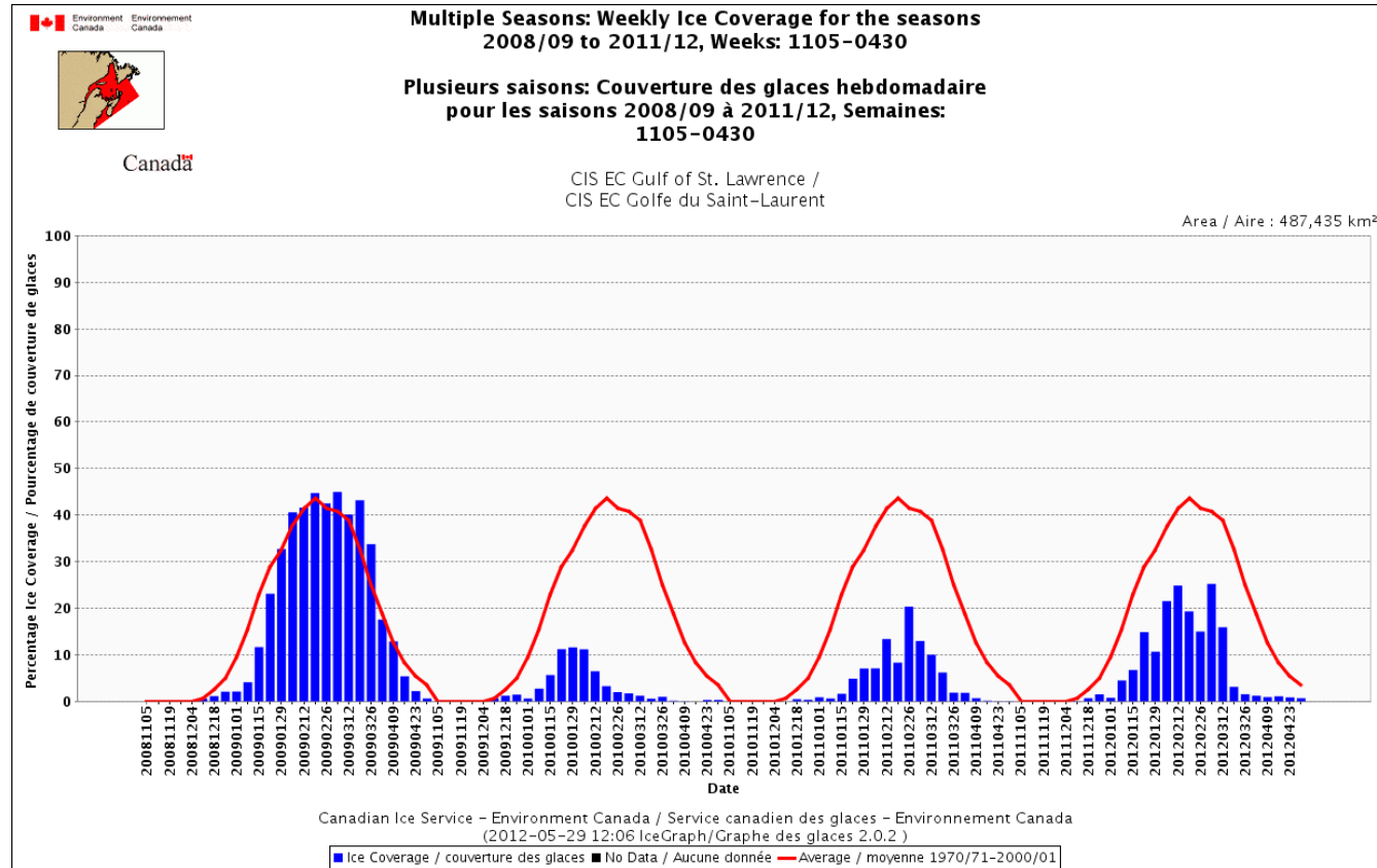
Figure 13 Évolution hebdomadaire du pourcentage d'englacement de l'estuaire et du golfe du Saint-Laurent et normale 1970-2000
