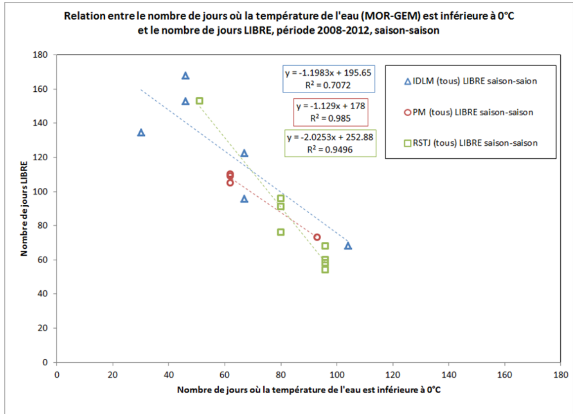
Figure 132 Relation entre le nombre de jours où la température de l'eau est inférieure à 0 °C et le nombre de jours LIBRE
