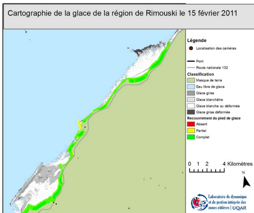
Figure 164 Cartographie de la glace littorale de la région de Rimouski
