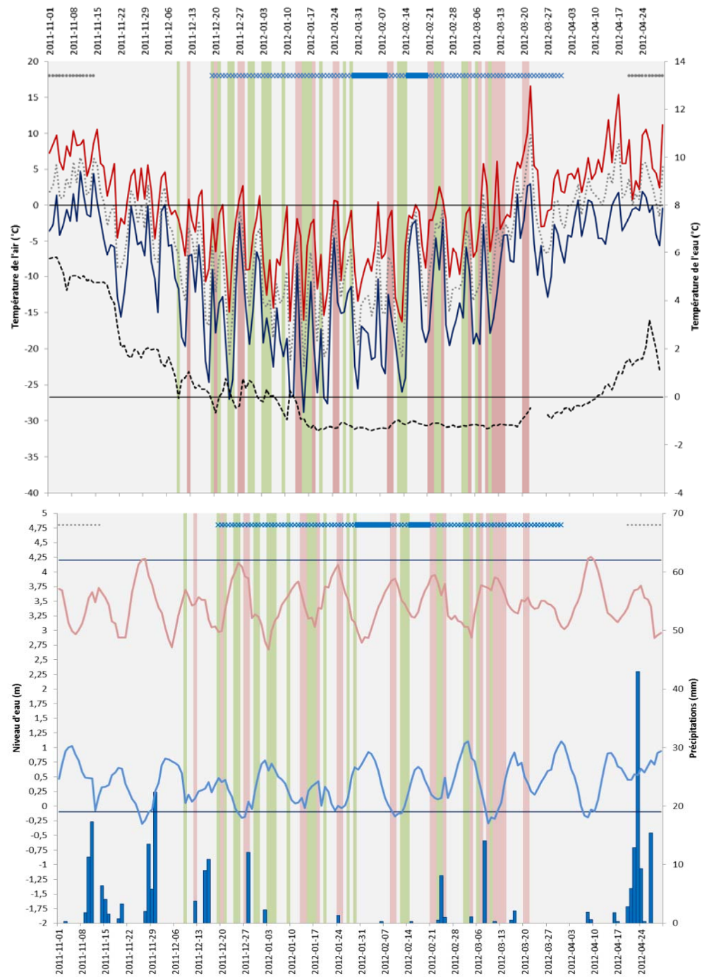
Figure 25 Saison glacielle 2011-2012, caméra 3, Pointe-Lebel, péninsule de Manicouagan, Côte-Nord
