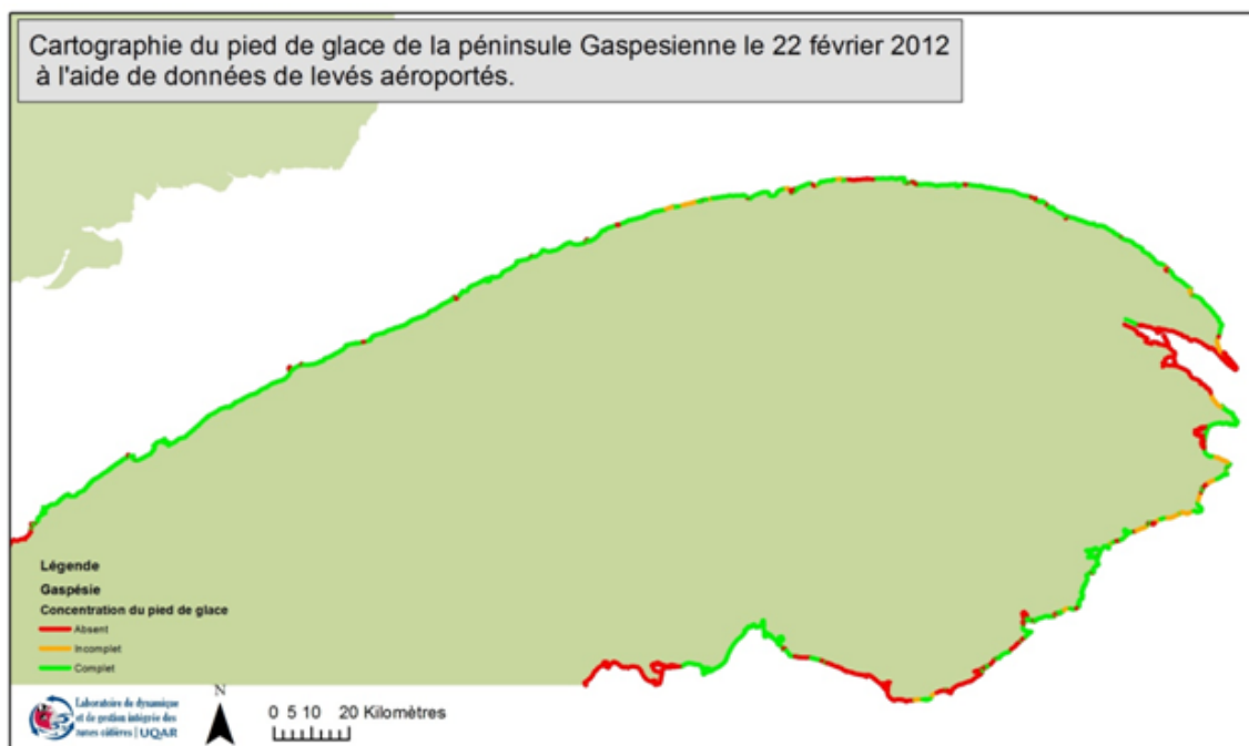
Figure 170 Cartographie de la présence de pied de glace sur les côtes de la péninsule gaspésienne à partir des données d'observation aéroportée du pied de glace
