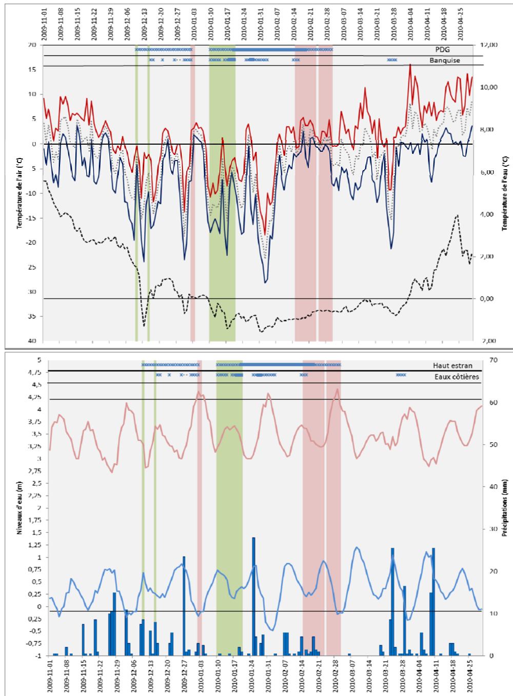
Figure 24 Saison glacielle 2009-2010, Baie-Saint-Ludger, péninsule de Manicouagan, Côte-Nord
