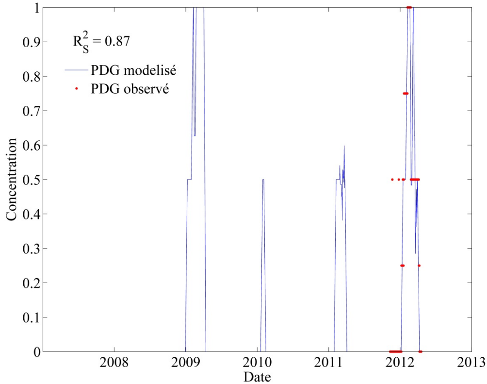
Figure 45 Série temporelle (2008-2013) du pied de glace à Rivière-Saint-Jean, site 2. Les observations semi-quantitatives (0=absence, 0,5=présence et 1=couvert complet) sont en rouge et le résultat de la relation empirique est en bleu. Comme plusieurs stations adjacentes sont moyennées, des valeurs intermédiaires pour les observations sont présentes. Le coefficient de corrélation de Spearman ( R_s^2 ) est indiqué dans le coin supérieur gauche de la figure
