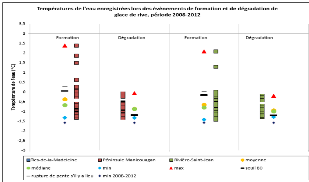
Figure 117 Température de l'eau observée à Sept-Îles lors des événements de formation et de dégradation sur les sites de la péninsule de Manicouagan et de Rivière-Saint-Jean
