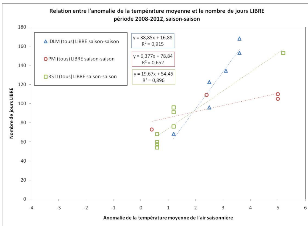
Figure 139 Relation entre les anomalies de températures de l'air et le nombre de jours LIBRE durant la saison, période 2008-2012
