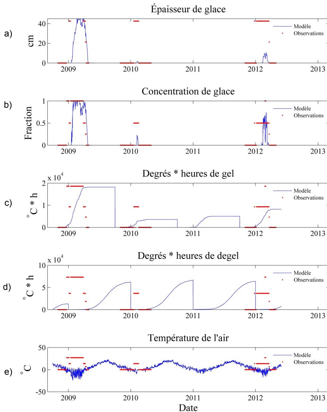
Figure 34 Exemples de variables du simulateur numérique pouvant être utilisées pour déterminer la relation empirique avec les observations : épaisseur de glace (a), concentration de glace (b), degrés-heures de gel (c), degrés-heures de dégel (d) et température de l'air à 2 m (e)
