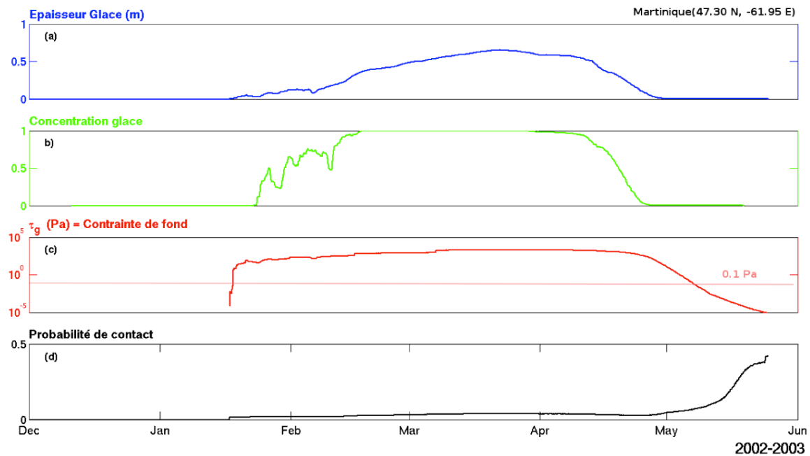
Figure 89 Séries temporelles de a) l'épaisseur, b) la concentration, c) contrainte au fond et d) la probabilité de contact au point de grille (47,03°N, 61,95°O), près de La Martinique, aux Îles-de-la-Madeleine pour l'hiver 2002-2003
