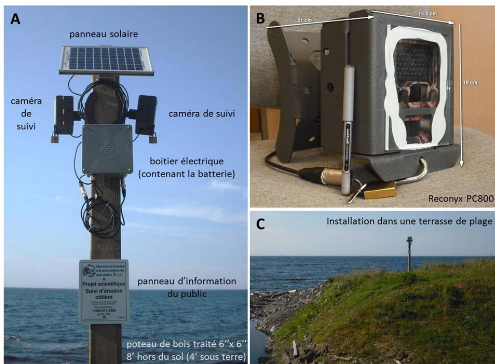
Figure 4 Caméra Reconyx sur le terrain
