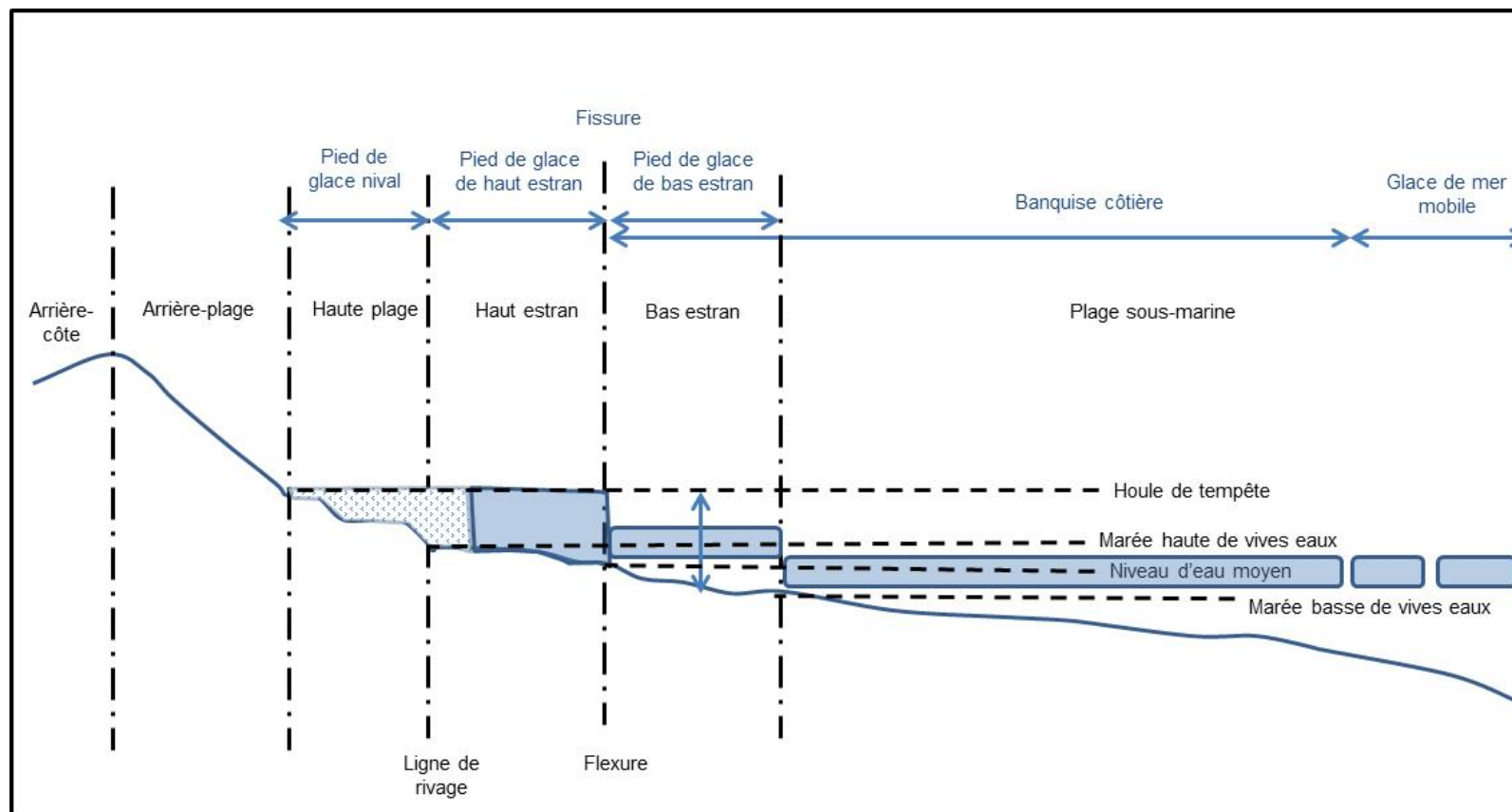
Figure 1 Représentation schématique du complexe glaciaire côtier sur une côte basse meuble
