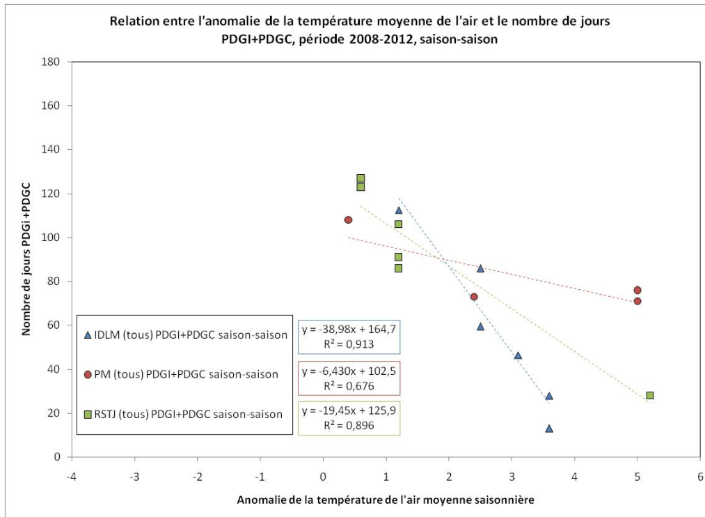
Figure 138 Relation entre les anomalies de températures de l'air et le nombre de jours PDGI+PDGC durant la saison, période 2008-2012
