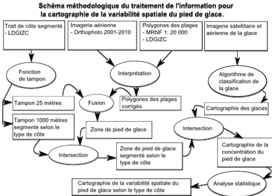
Figure 62 Schéma méthodologique de la cartographie de la variabilité spatiale du pied de glace
