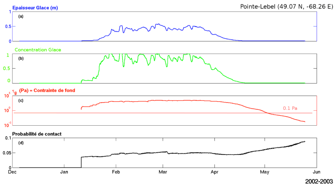
Figure 88 Séries temporelles de a) l'épaisseur, b) la concentration, c) contrainte au fond et d) la probabilité de contact au point de grille (49,07°N, 68,26°O), près de Pointe-Lebel, pour l'hiver 2002-2003
