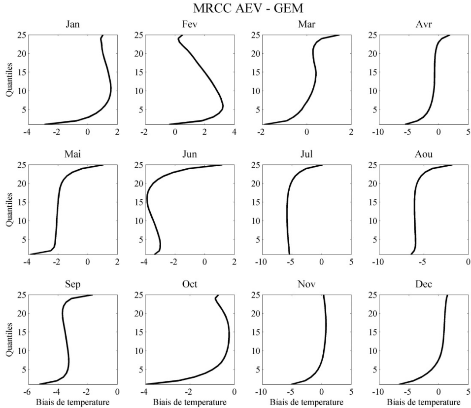
Figure 145 Biais par quantile pour la simulation forcée par MRCC-AEV
