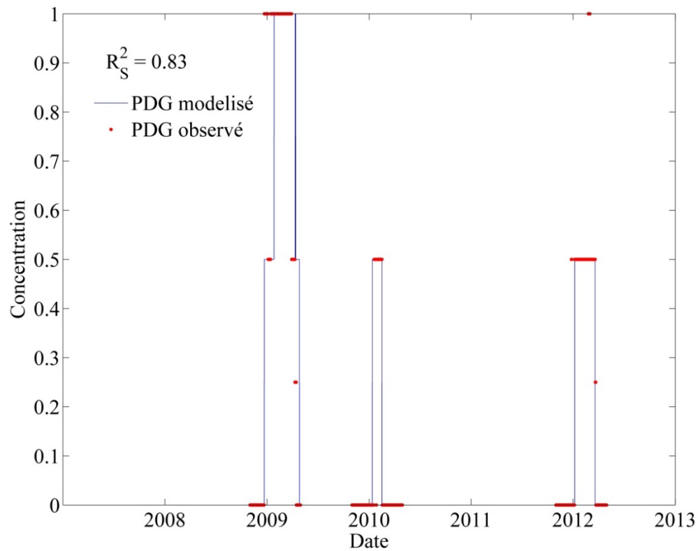
Figure 42 Série temporelle (2008-2013) du pied de glace à La Martinique, aux Îles-de-la-Madeleine. Les observations semi-quantitatives (0=absence, 0,5=présence et 1=couvert complet) sont en rouge et le résultat de la relation empirique est en bleu. Comme plusieurs stations adjacentes sont moyennées, des valeurs intermédiaires pour les observations sont présentes. Le coefficient de corrélation de Spearman ( R_s^2 ) est indiqué dans le coin supérieur gauche de la figure
