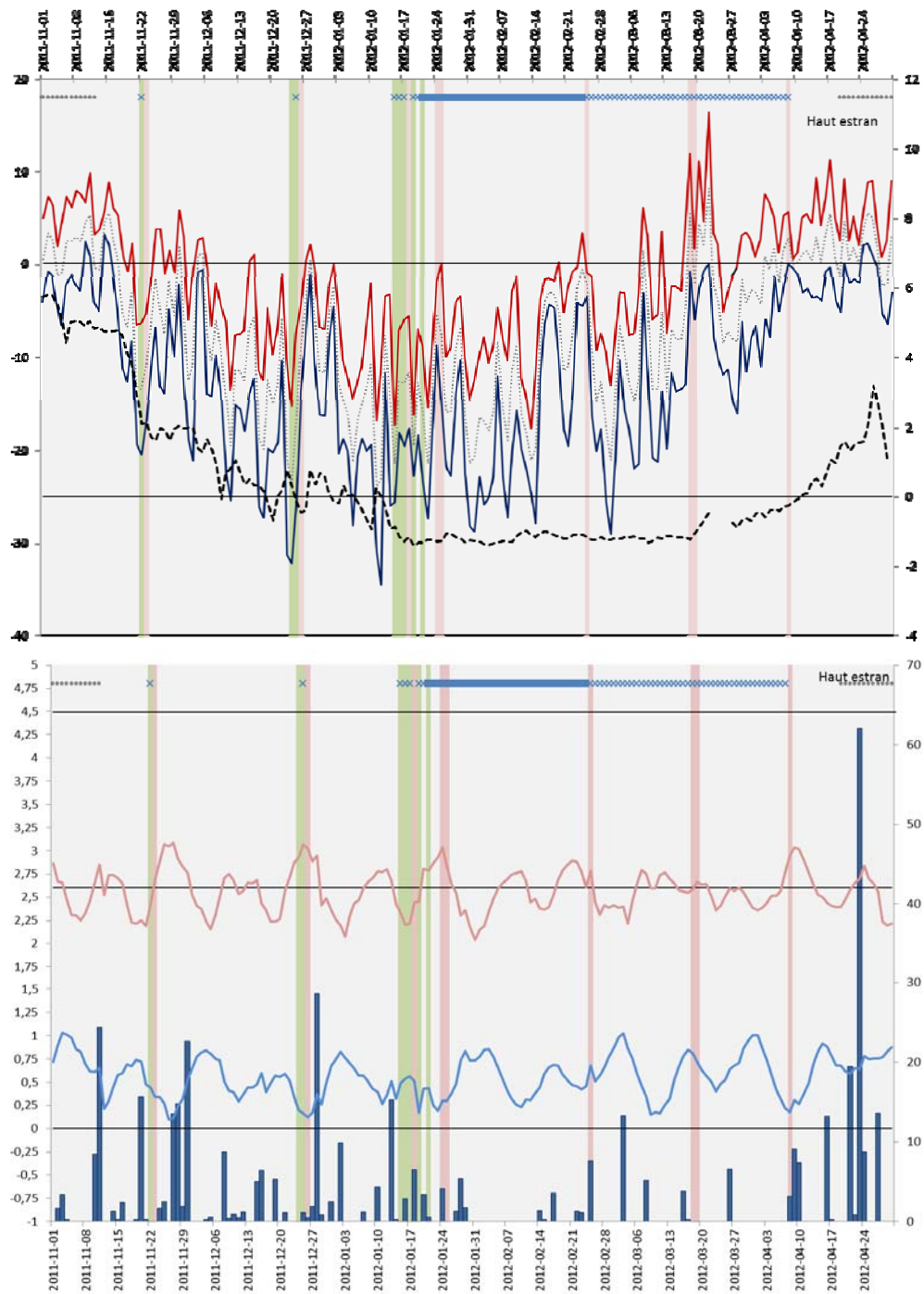
Figure 29 Saison glacielle 2011-2012, caméra OUEST, Côte-Nord
