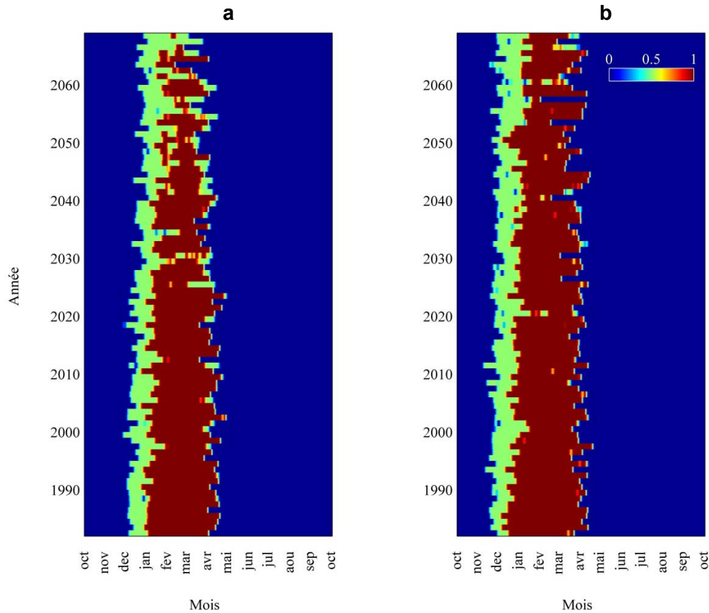
Figure 50 Séries temporelles du PDG à la péninsule de Manicouagan, site de Pointe-Lebel, pour la simulation MOR-AEV-bTq (a) et la simulation MOR-AHJ (b). Les années sont sur l'axe vertical (de 1981 à 2070), les mois, sur l'axe horizontal, et l'échelle de couleurs représente la fraction de la région couverte par le PDG
