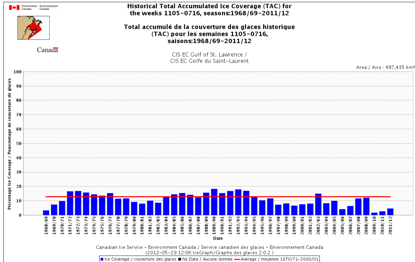
Figure 12 Total accumulé de la couverture des glaces de 1968 à 2011
