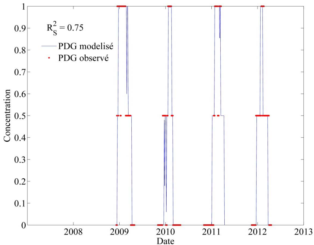
Figure 43 Série temporelle (2008-2013) du pied de glace à Pointe-Lebel, péninsule de Manicouagan. Les observations semi-quantitatives (0=absence, 0,5=présence et 1=couvert complet) sont en rouge et le résultat de la relation empirique est en bleu. Le coefficient de corrélation de Spearman ( R_s^2 ) est indiqué dans le coin supérieur gauche de la figure
