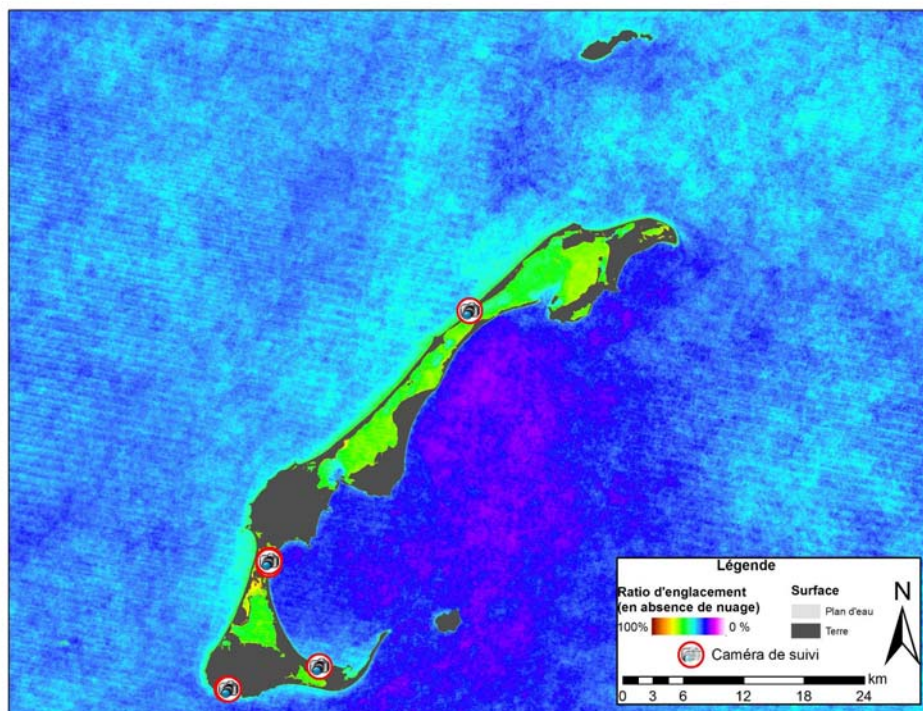
Figure 68 Ratio d'englacement pour les îles de la Madeleine, de 1996 à 2012
