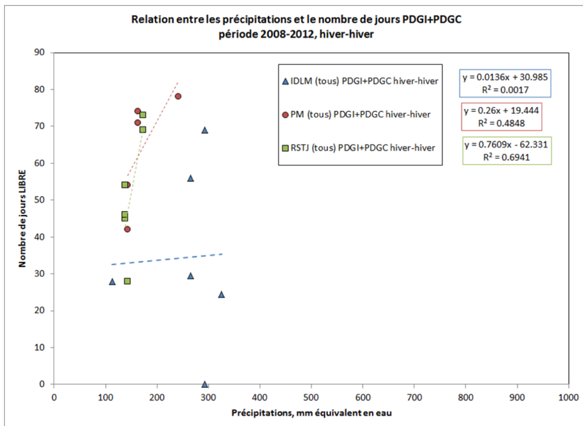
Figure 135 Relation entre les précipitations hivernales et le nombre de jours PDGI+PDGC durant l'hiver
