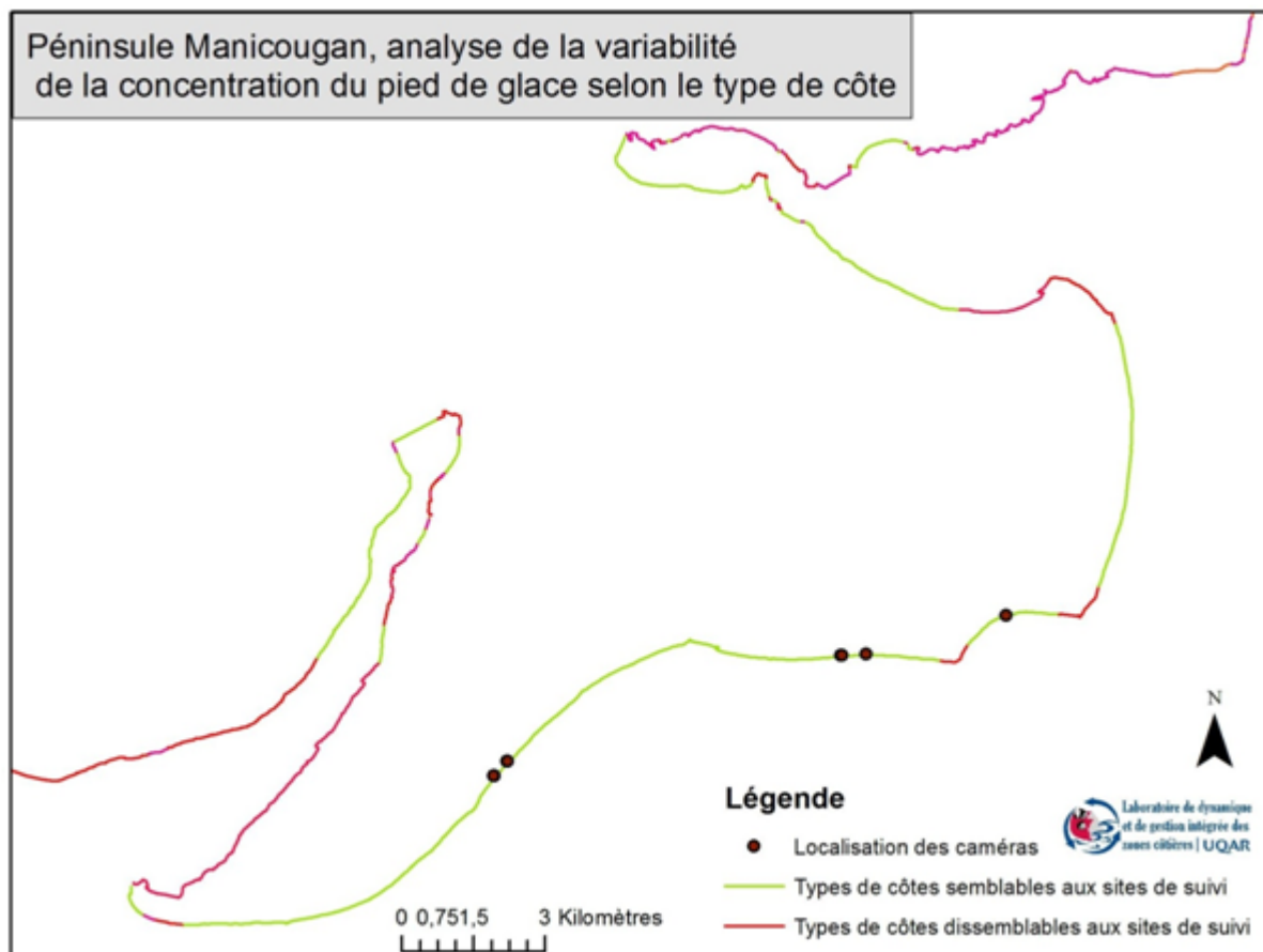
Figure 73 Cartographie de l'analyse de la variabilité spatiale du pied de glace de la région de la péninsule de Manicouagan
