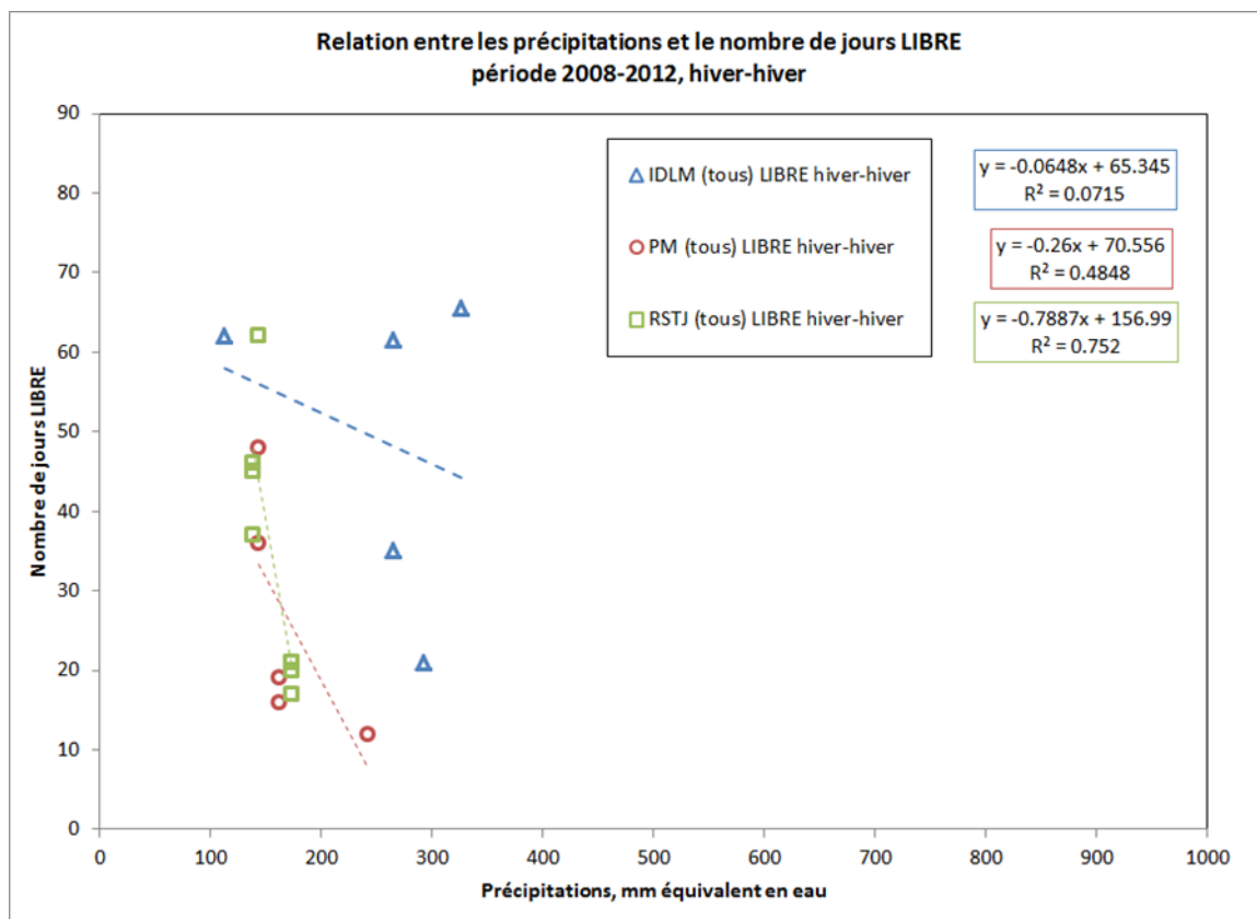
Figure 134 Relation entre les précipitations hivernales et le nombre de jours LIBRE durant l'hiver
