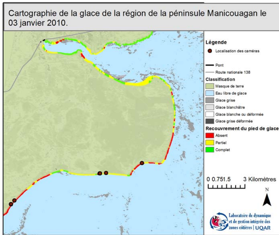
Figure 162 Cartographie de la glace littorale de la région de la péninsule de Manicouagan, le 3 janvier 2010
