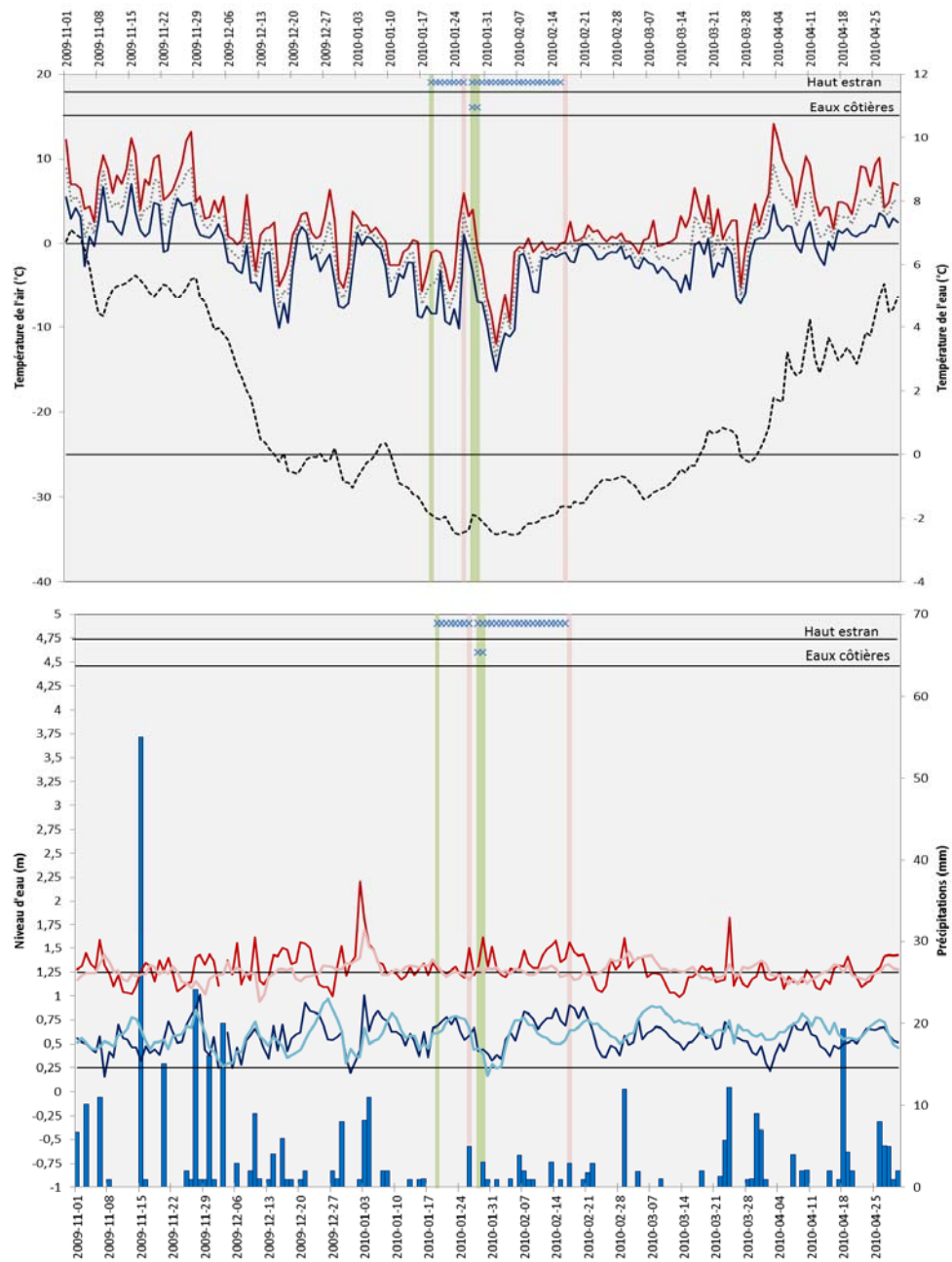
Figure 17 Saison glacielle 2009-2010, La Martinique, Îles-de-la-Madeleine
