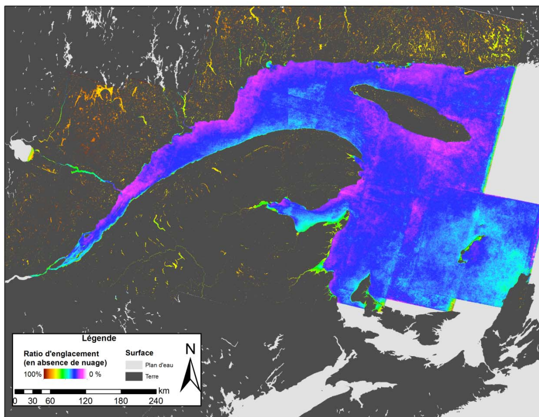
Figure 96 Fréquence d'englacement par temps clair du golfe et de l'estuaire du Saint-Laurent. Celle-ci est définie comme étant le ratio entre le nombre d'images sur lesquelles un pixel de 30 m×30 m est couvert de glace et le nombre total de pixels valides, c'est-à-dire sans nuage. Les zones à haut ratio d'englacement correspondent bien aux zones où la banquise interagit avec le fond (voir Figure 98)
