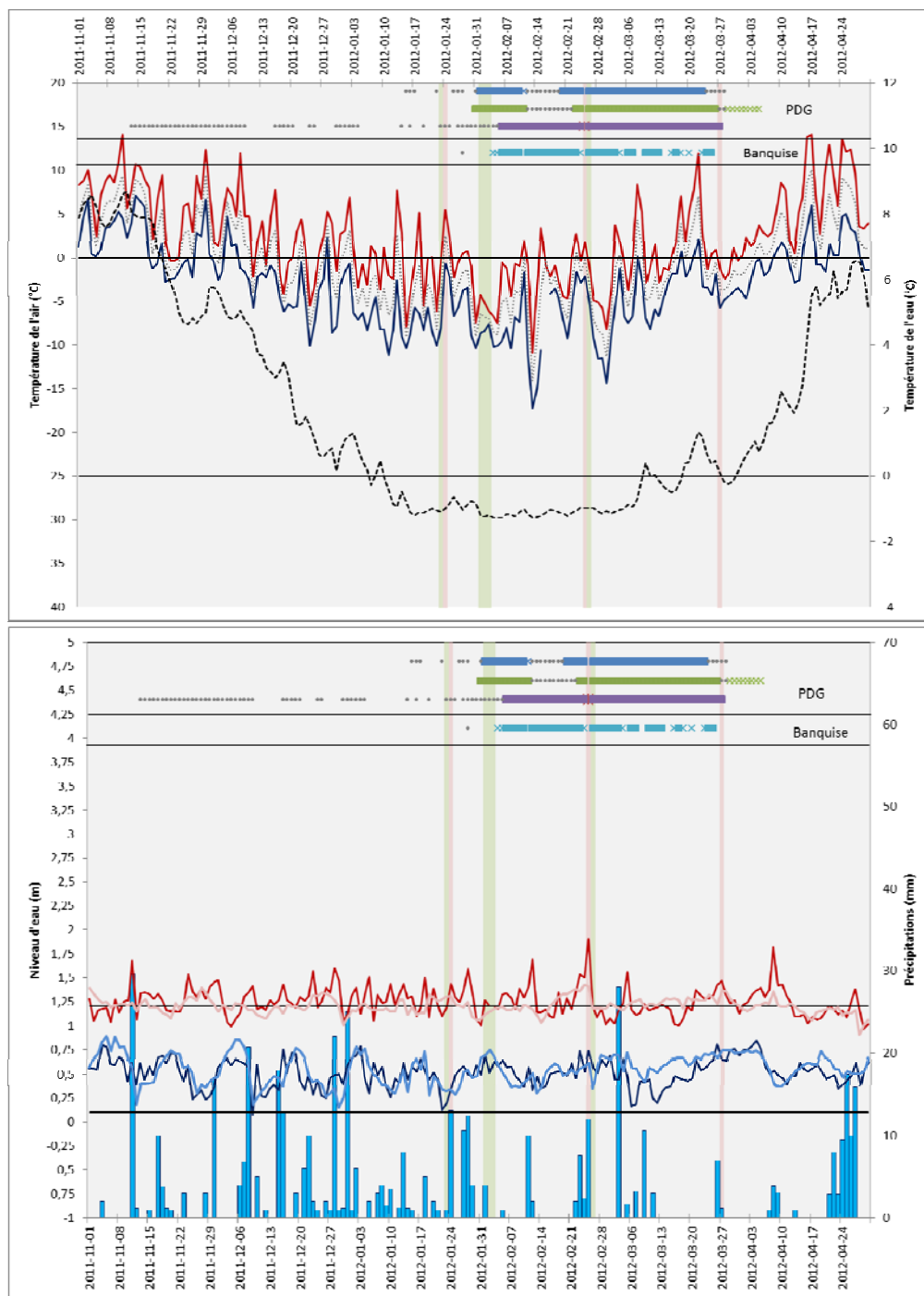
Figure 21 Saison glacielle 2011-2012, Pointe-aux-Loups, Îles-de-la-Madeleine
