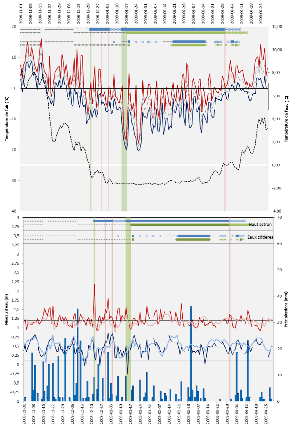
Figure 15 Saison glacielle 2008-2009, La Martinique, Îles-de-la-Madeleine
