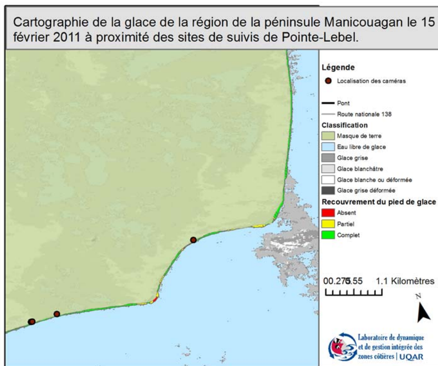
Figure 72 Cartographie de la glace littorale de la région de la péninsule de Manicouagan centrée sur le site de Pointe-Lebel
