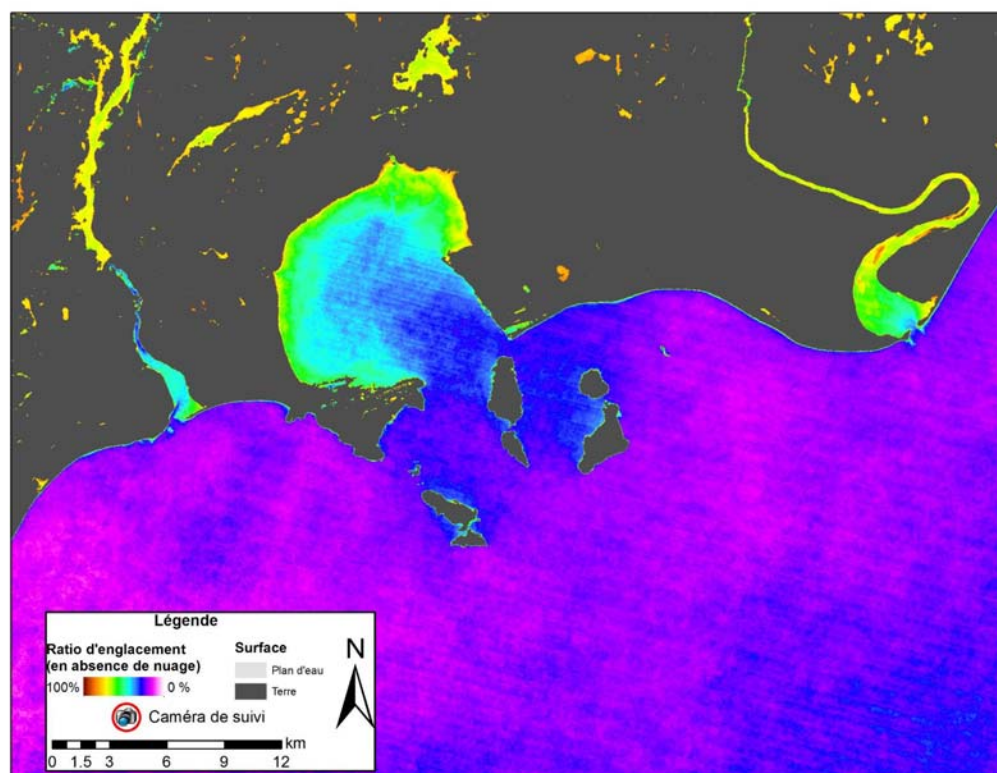
Figure 65 Ratio d'englacement dans le secteur de Sept-Îles. À droite, la rivière Moisie ; à gauche, la rivière Sainte-Marguerite
