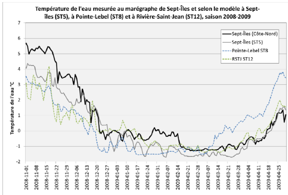
Figure 116 Température de l'eau enregistrée au marégraphe de Sept-Îles et selon le modèle MOR-GEM à Sept-Îles (ST5), Pointe-Lebel (péninsule de Manicouagan) (ST8) et Rivière-Saint-Jean (ST12)
