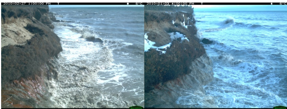
Figure 113 État de la nappe d'eau : ressacs visibles
