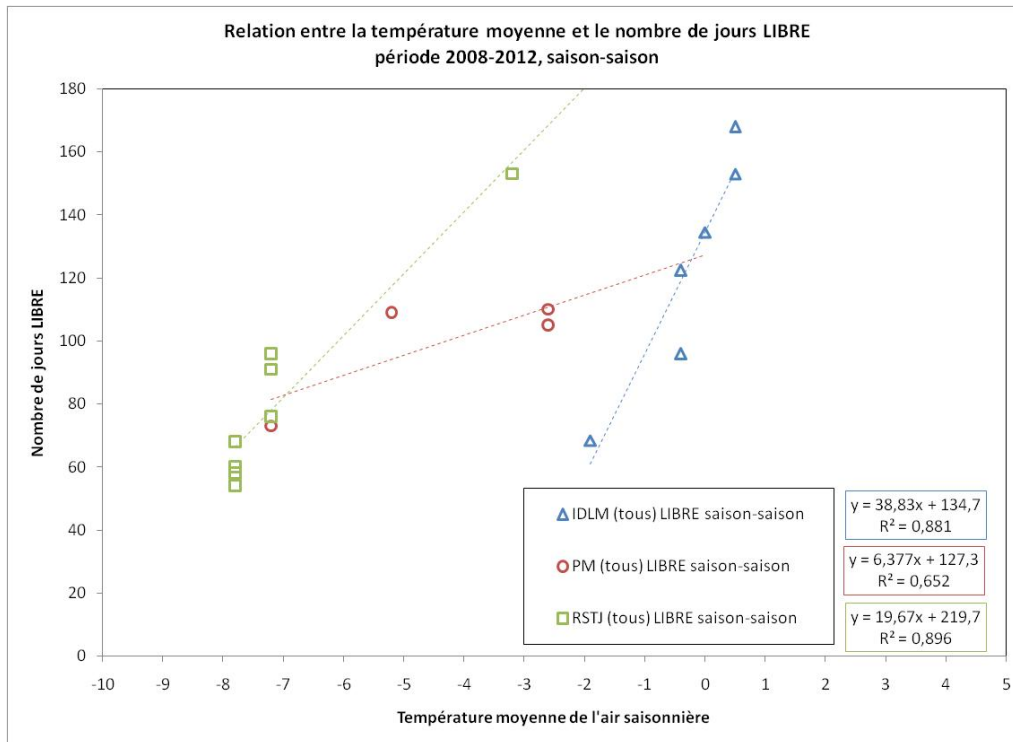
Figure 137 Relation entre les températures de l'air moyennes et le nombre de jours LIBRE durant la saison, période 2008-2012
