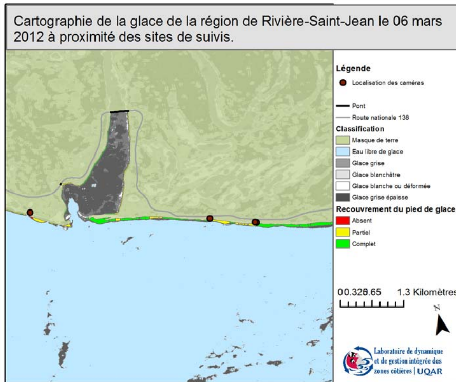
Figure 75 Agrandissement de la cartographie de la glace littorale de la région de l'embouchure de la rivière Saint-Jean, sur la Côte-Nord
