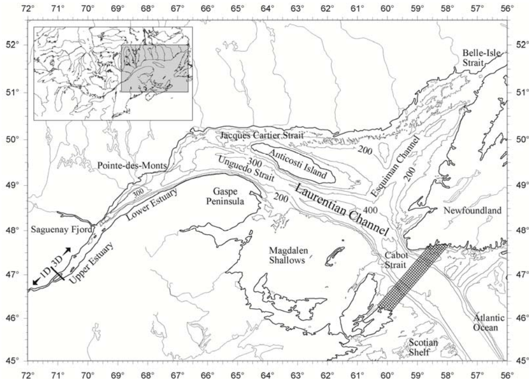
Figure 32 Domaine du simulateur MOR (tirée de Saucier et collab. 2003)
