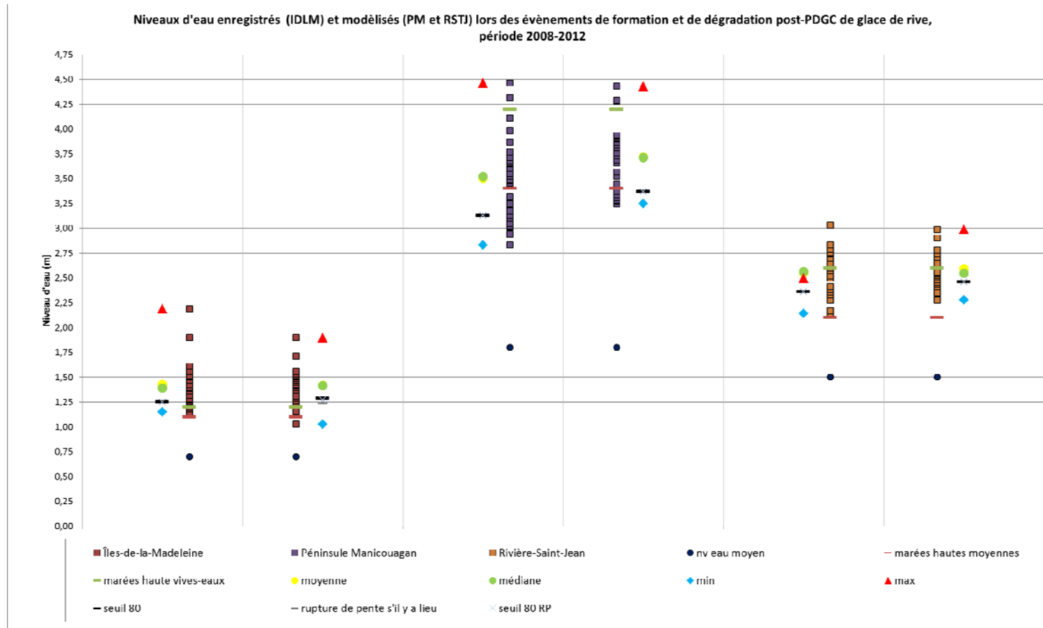
Figure 118 Répartition des niveaux d'eau observés (Cap-aux-Meules) et modélisés (PM et RSTJ) lors des événements de formation et de dégradation de glace de rive
