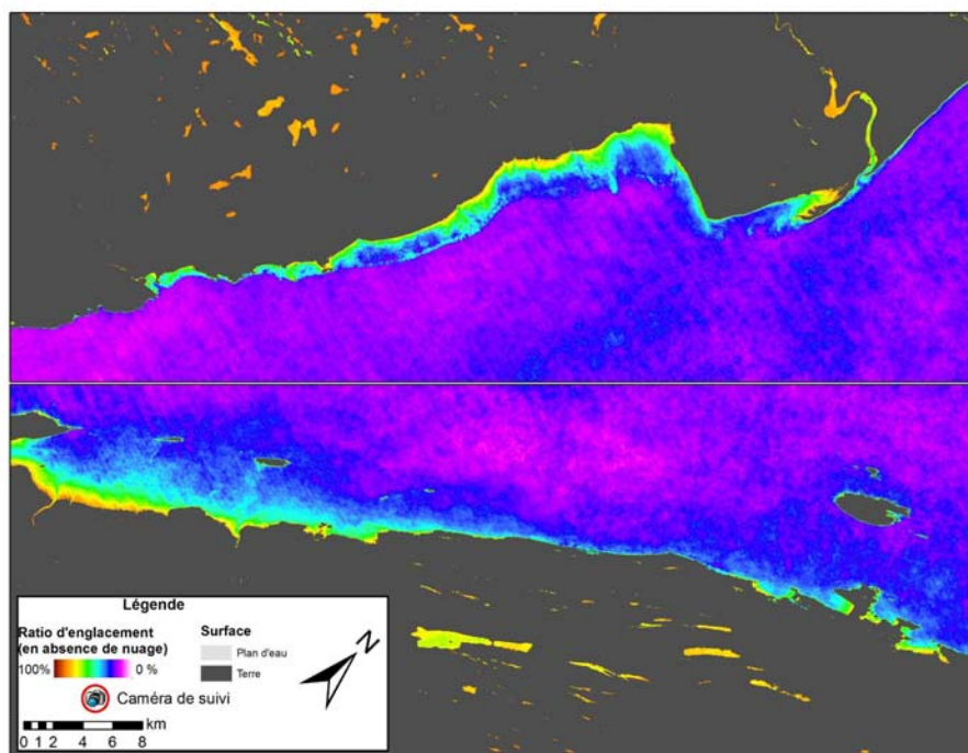
Figure 70 Ratio d'englacement pour la zone des Escoumins, à Portneuf-sur-mer (haut), et de l'Isle-Verte, au Bic (bas), de 1996 à 2012
