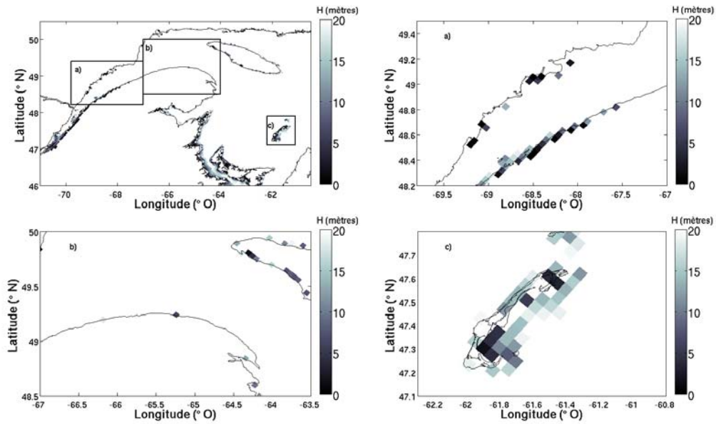
Figure 86 Bathymétrie moyenne du golfe du Saint-Laurent (en haut à gauche) avec accent mis sur les 20 premiers mètres, montrant ainsi les endroits où la glace est susceptible de s'ancrer au fond (agrandissement a, b et c représentant respectivement l'estuaire maritime, la côte nord de la Gaspésie et les îles de la Madeleine)
