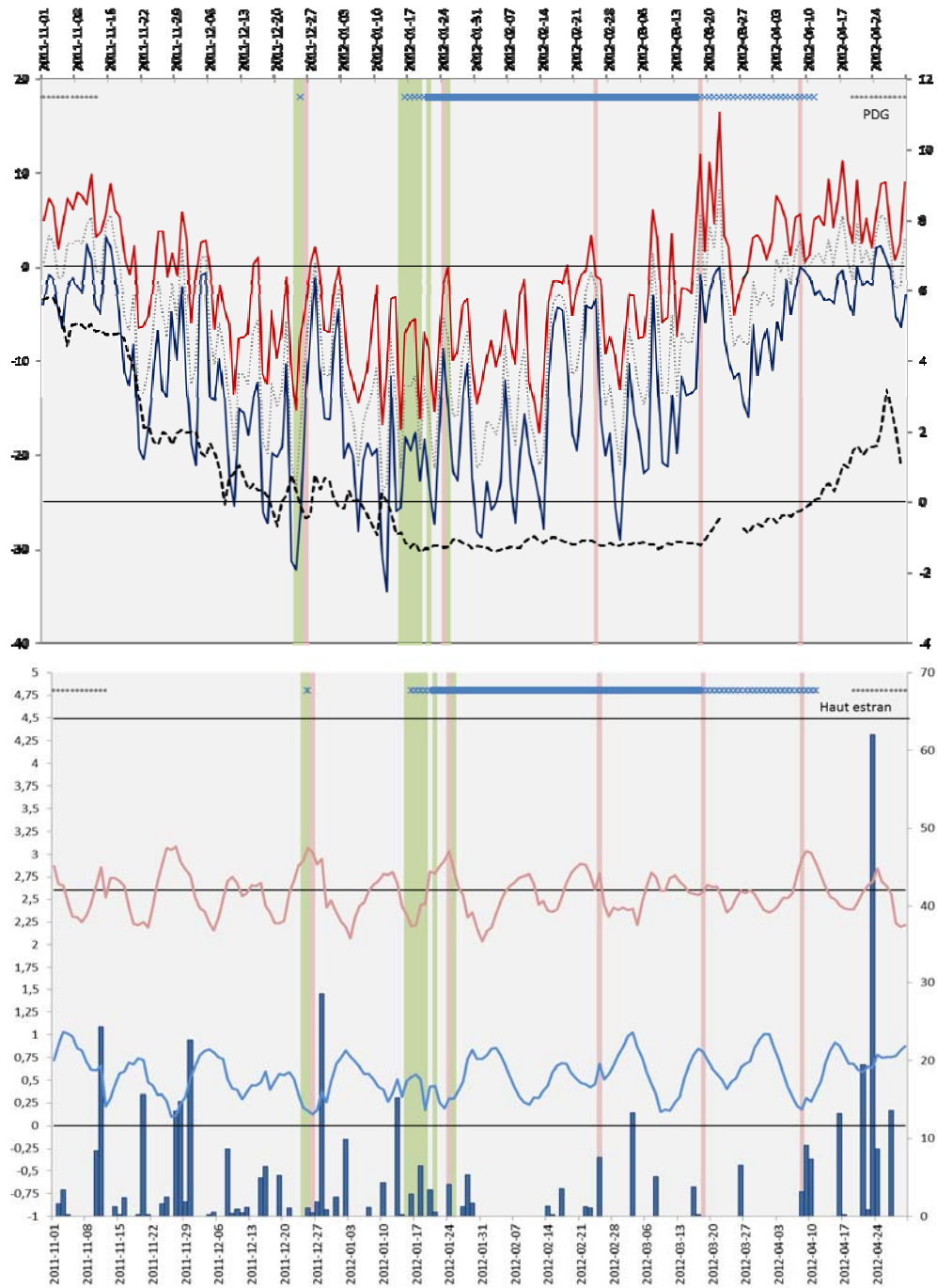
Figure 30 Saison glacielle 2011-2012, caméra HORIZONTAL, Rivière-Saint-Jean, Côte-Nord
