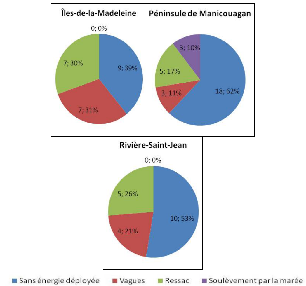
Figure 114 Répartition de l'état d'agitation de la mer lors de la dégradation du pied de glace observée pour chacun des sites d'étude durant la période 2008-2012
