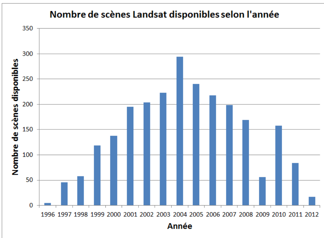
Figure 56 Répartition du nombre de scènes Landsat disponibles pour le traitement
