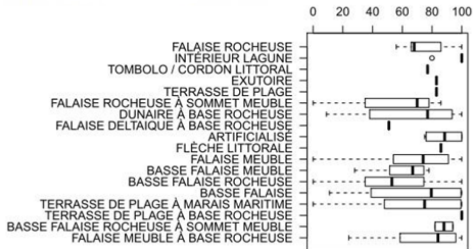
Figure 80 Diagramme à boîtes et moustaches de la concentration de glace estimée par RDO sur la zone pouvant accueillir un pied de glace, selon le type de côte, pour le secteur nord des îles de la Madeleine, le 13 février 2013
