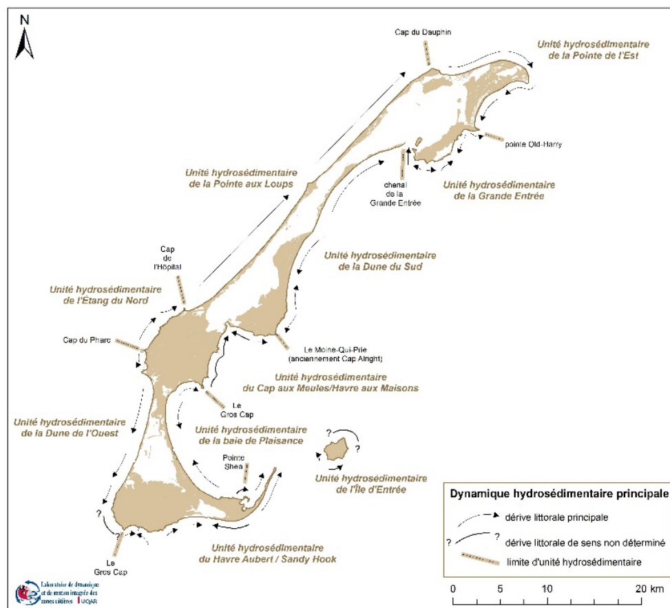
Figure 9 Unités hydrosédimentaires des Îles-de-la-Madeleine
