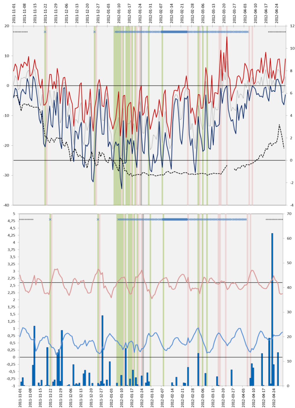
Figure 28 Saison glacielle 2011-2012, Rivière-Saint-Jean, caméra EST
