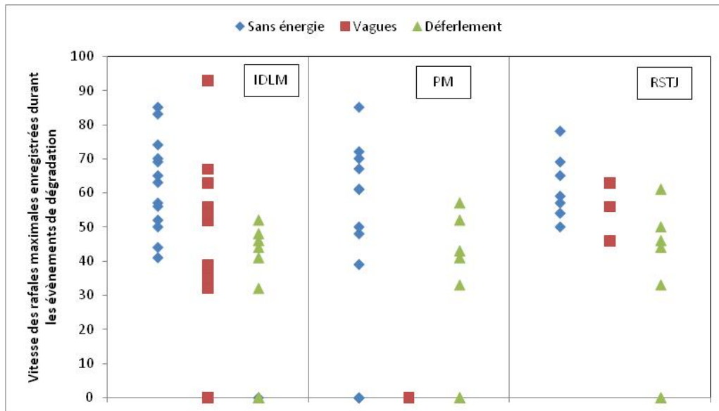
Figure 120 Vitesse des rafales maximales enregistrées lors des évènements de dégradation post-PDGC selon le niveau d'énergie déployée contre la glace pour chacun des sites d'étude
