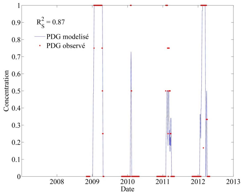
Figure 41 Série temporelle (2008-2013) du pied de glace à Pointe-aux-Loups, aux Îles-de-la-Madeleine. Les observations semi-quantitatives (0=absence, 0,5=présence et 1=couvert complet) sont en rouge et le résultat de la relation empirique est en bleu. Comme plusieurs stations adjacentes sont moyennées, des valeurs intermédiaires pour les observations sont présentes. Le coefficient de corrélation de Spearman ( R_s^2 ) est indiqué dans le coin supérieur gauche de la figure
