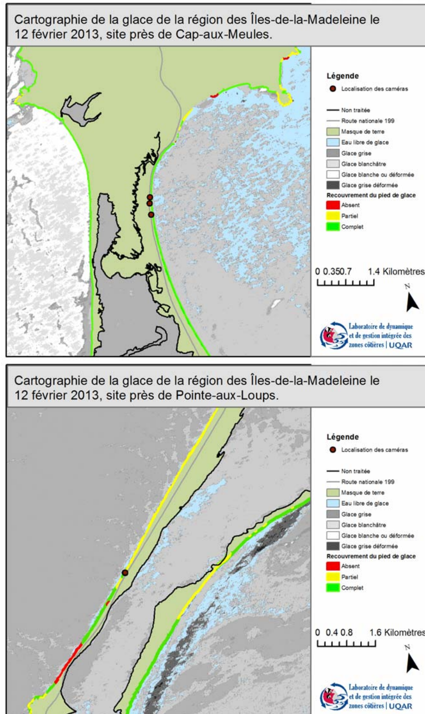
Figure 79 Agrandissement de la cartographie de la glace littorale des îles de la Madeleine pour les sites de Cap-aux-Meules (haut) et de Pointe-aux-Loups (bas)
