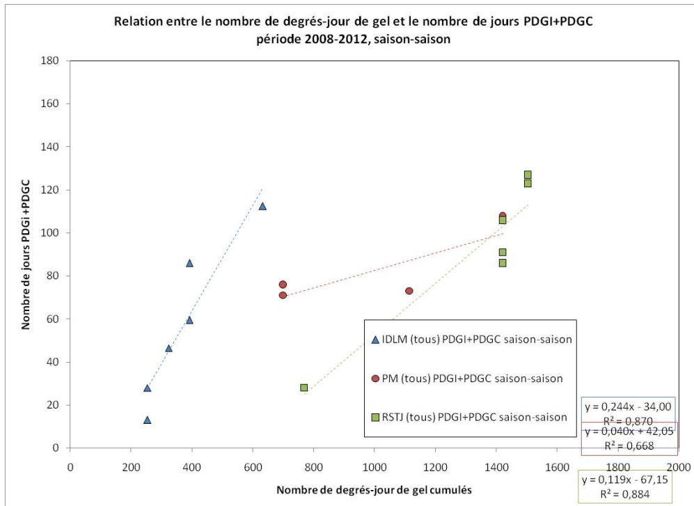
Figure 141 Relation entre le nombre de degrés-jours de gel et le nombre de jours PDGI+PDGC durant la saison, période 2008-2012
