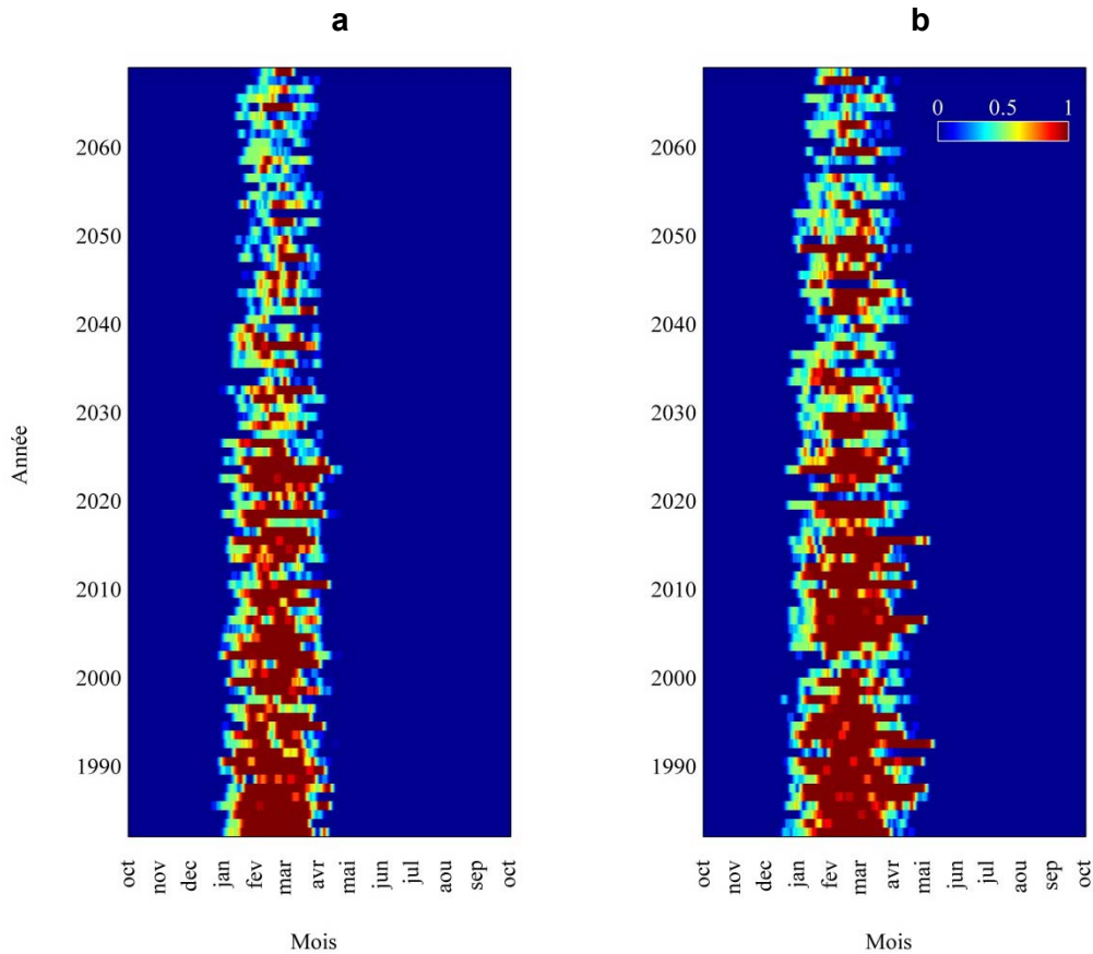
Figure 46 Séries temporelles du PDG aux Îles-de-la-Madeleine, site de Pointe-aux-Loups, pour la simulation MOR-AEV-bTq (a) et la simulation MOR-AHJ (b). Les années sont sur l'axe vertical (de 1981 à 2070), les mois sur l'axe horizontal et l'échelle de couleurs représente la fraction de la région couverte par le PDG
