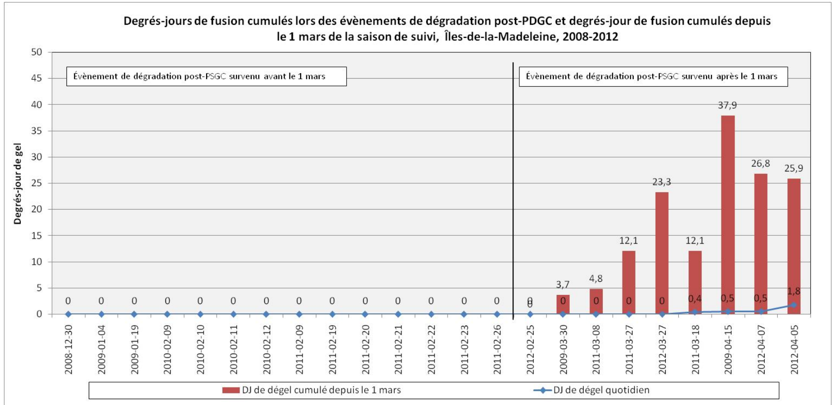
Figure 123 Nombre de degrés-jours de fonte cumulés quotidiennement et depuis le 1 er mars, lorsque applicable lors des événements de dégradation de glace de rive post-PDGC, Îles-de-la-Madeleine, 2008-2012
