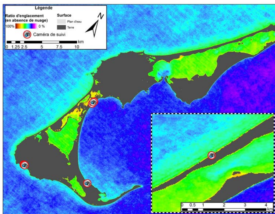
Figure 69 Ratio d'englacement pour le sud des îles de la Madeleine et le site de Pointe-aux-Loups, de 1996 à 2012
