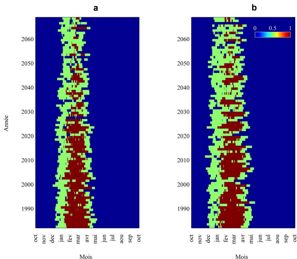
Figure 48 Séries temporelles du PDG aux Îles-de-la-Madeleine, site de La Martinique, pour la simulation MOR-AEV-bTq (a) et la simulation MOR-AHJ (b). Les années sont sur l'axe vertical (de 1981 à 2070), les mois, sur l'axe horizontal, et l'échelle de couleurs représente la fraction de la région couverte par le PDG
