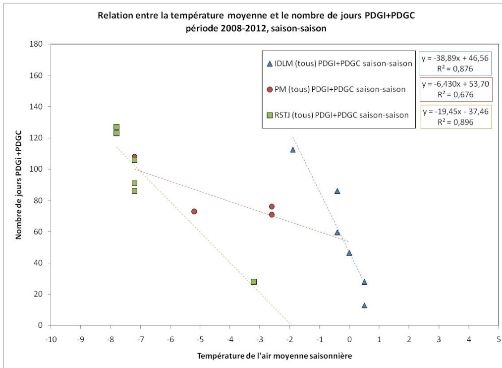
Figure 136 Relation entre les températures de l'air moyennes et le nombre de jours PDGI+PDGC durant la saison, période 2008-2012
