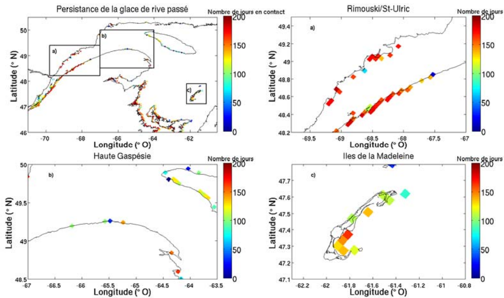
Figure 97 Carte de la persistance moyenne du pied de glace en nombre de jours pendant les quels la contrainte au fond a dépassé 0,1 Pa pour le golfe et l'estuaire (en haut, à gauche) pour le climat du passé récent (1982-2006) (agrandissement a, b et c représentant respectivement l'estuaire maritime, la côte nord de la Gaspésie et les îles de la Madeleine)
