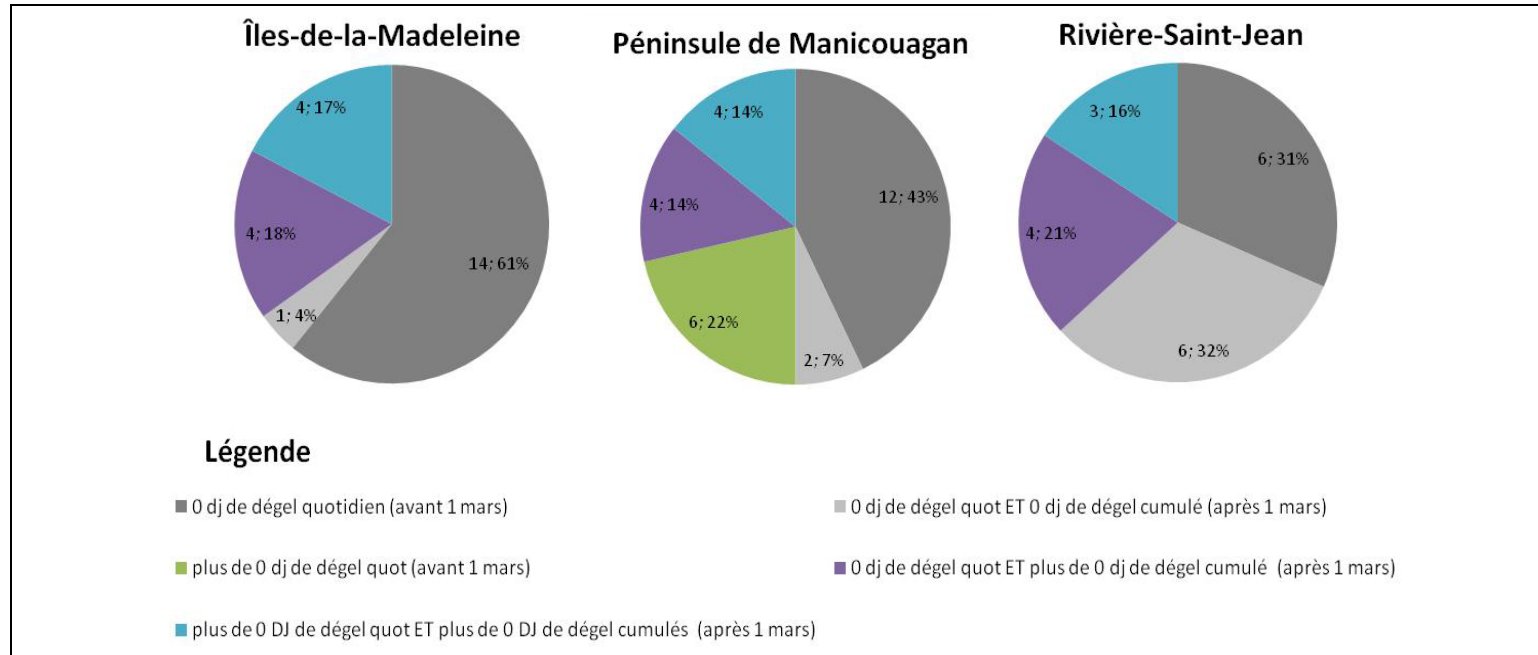
Figure 122 Degrés-jours de fonte enregistrés lors des évènements de dégradation post-PDGC
