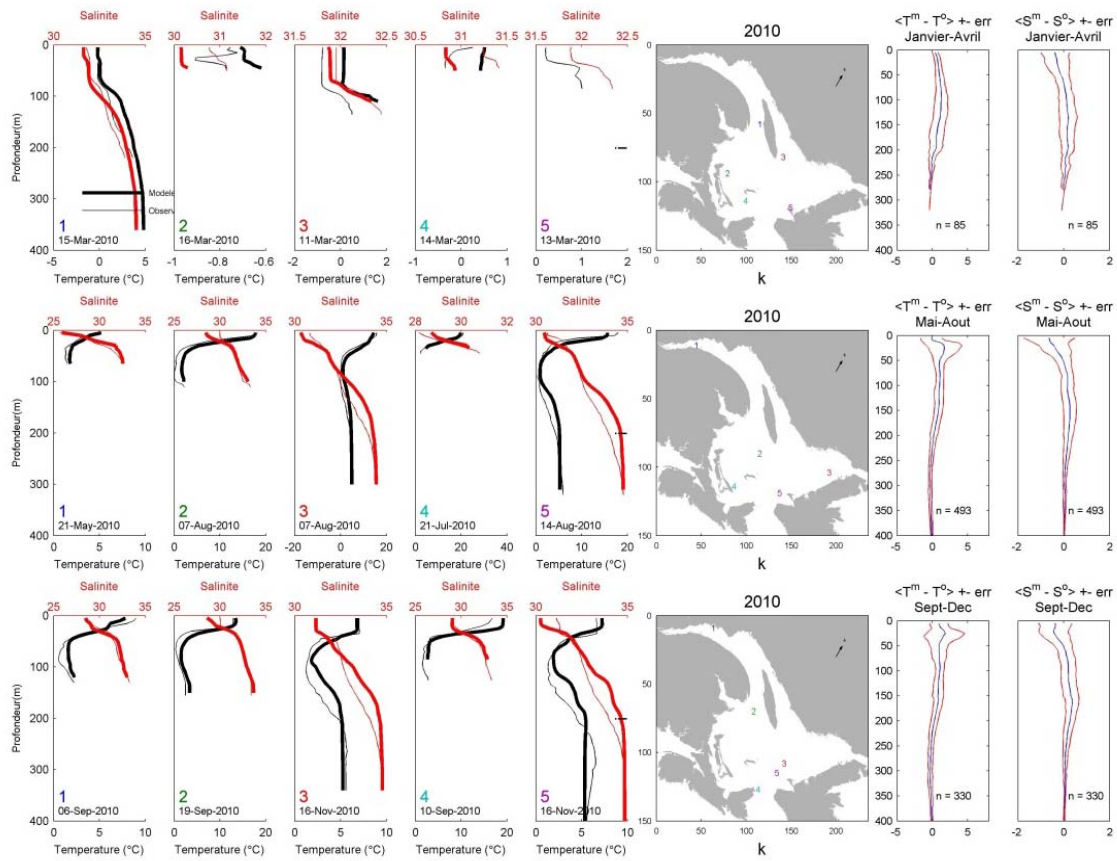
Figure 151 Comparaison de profils de température (en noir) et de salinité (en rouge). Les positions des stations sélectionnées de façon aléatoire sont présentées dans la sixième colonne. La moyenne (en bleu) et la déviation standard de l'erreur (en rouge) sur la température et la salinité sont dans les septième et huitième colonnes, respectivement
