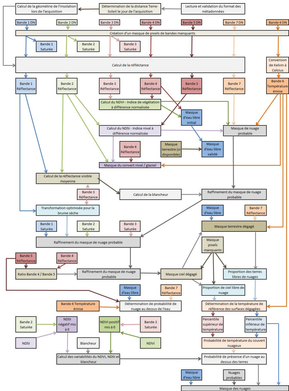
Figure 153 Procédure adaptée de classification automatisée de l'imagerie Landsat
