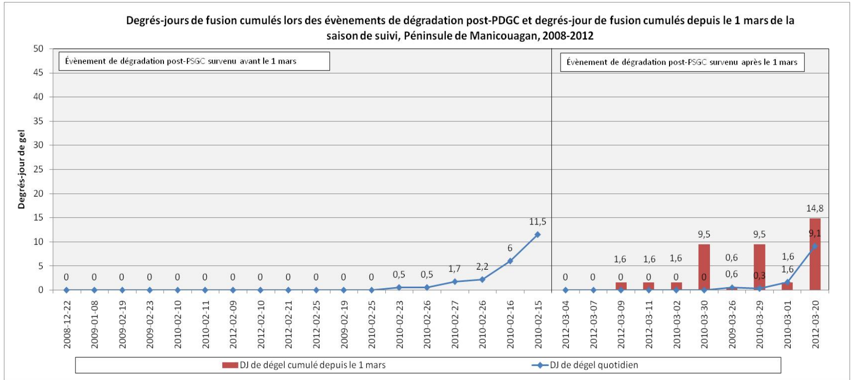
Figure 125 Nombre de degrés-jours de fonte cumulés quotidiennement et depuis le 1 er mars, lorsque applicable lors des événements de dégradation de glace de rive post-PDCG, péninsule de Manicouagan, 2008-2012
