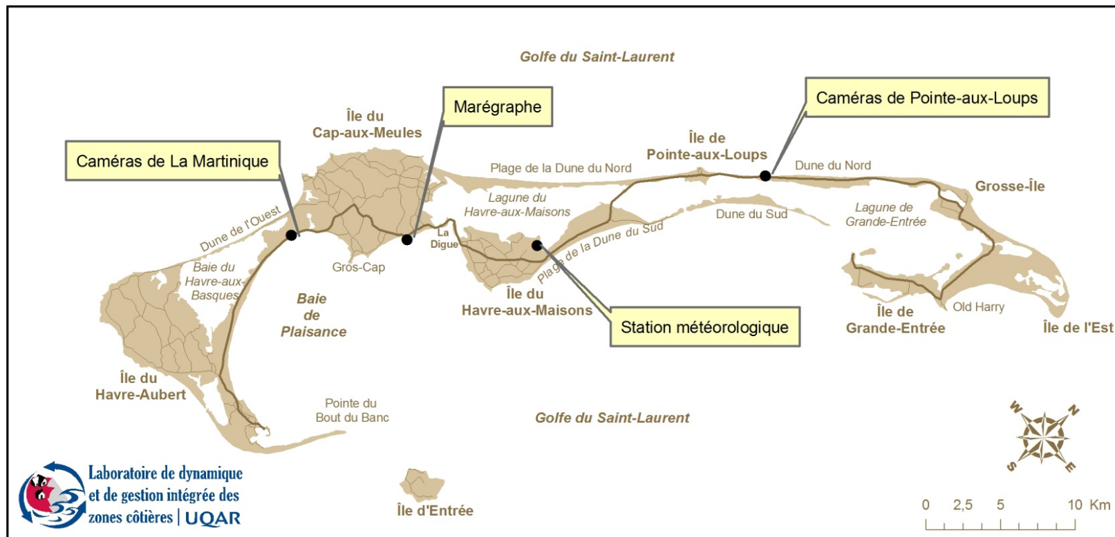
Figure 8 Localisation de l'instrumentation aux Îles-de-la-Madeleine
