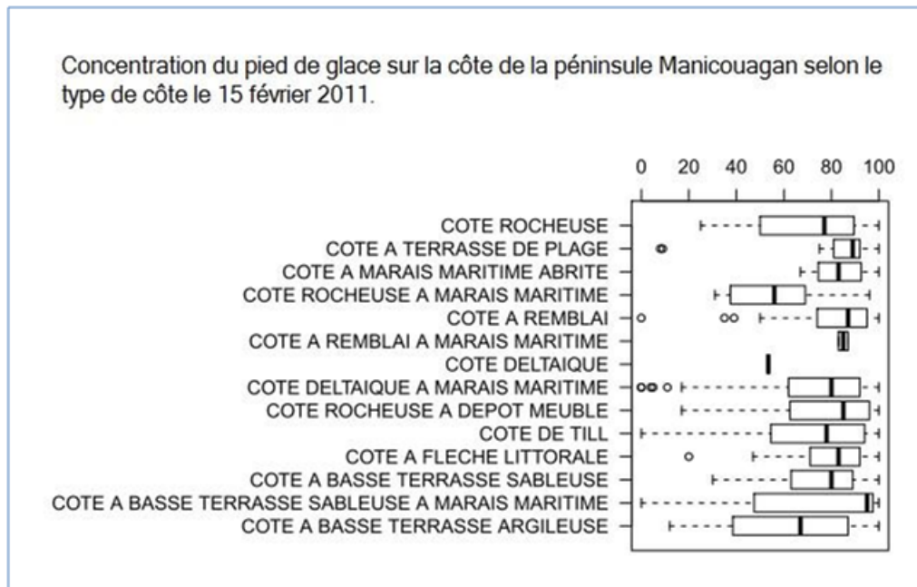
Figure 71 Diagramme à boîtes et moustaches de la concentration de glace mesurée sur la zone pouvant accueillir un pied de glace, selon le type de côte, pour la région de la péninsule de Manicouagan et ses environs
