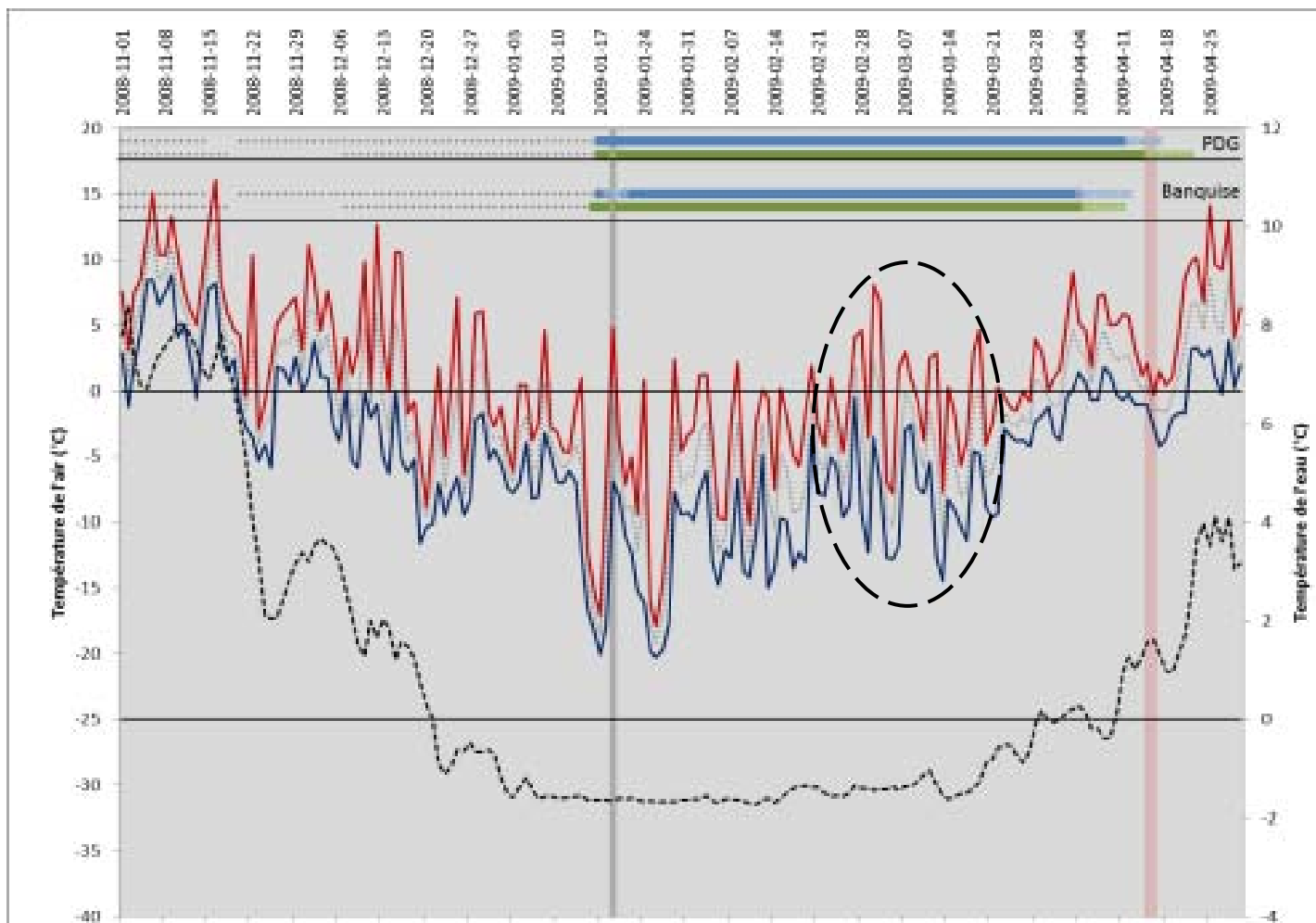
Figure 130 Températures de l'air et de l'eau et évolution de l'état d'englacement du haut estran et des eaux côtières à Pointe-aux-Loups, Îles-de-la-Madeleine, 2008-2009 : Exemple d'un redoux n'ayant pu affecter le pied de glace de haut estran en raison de l'englacement des eaux côtières
