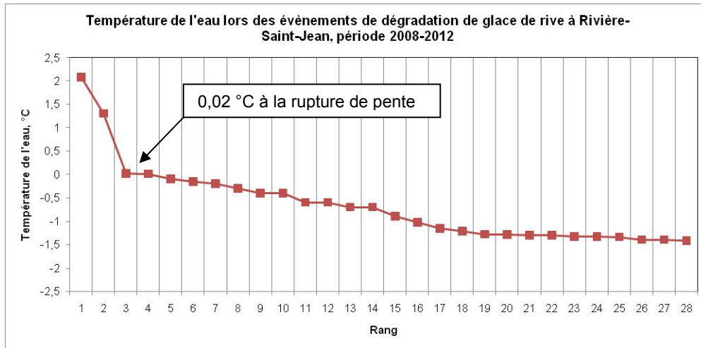
Figure 6 Représentation des températures de l'eau lors des évènements de dégradation de glace de rive à Rivière-Saint-Jean et identification de la rupture de pente
