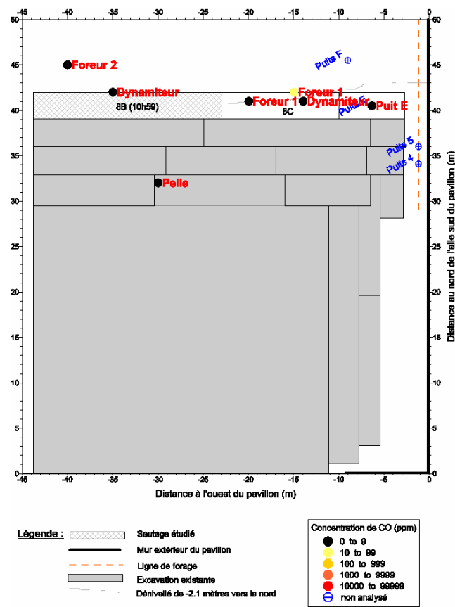
Figure 25 : Exposition d'un foreur au CO lors du forage à la suite du sautage 8B
