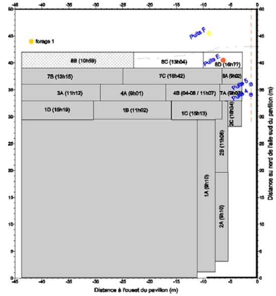
Teneur en CO dans le sol 1 @ 2 heures suivant le sautage 8B
