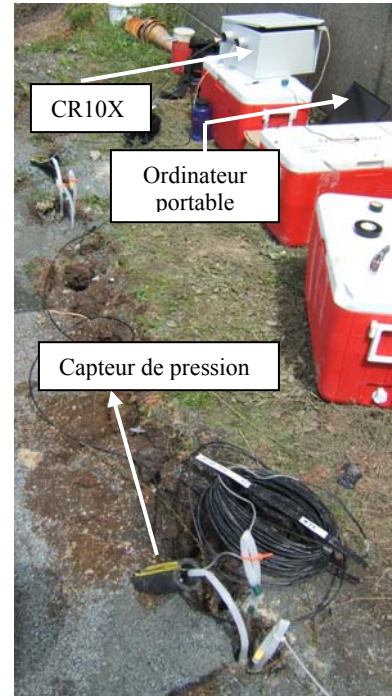
Figure 5 : Instrumentation pour la prise de pressions dans les puits pendant les sautages
