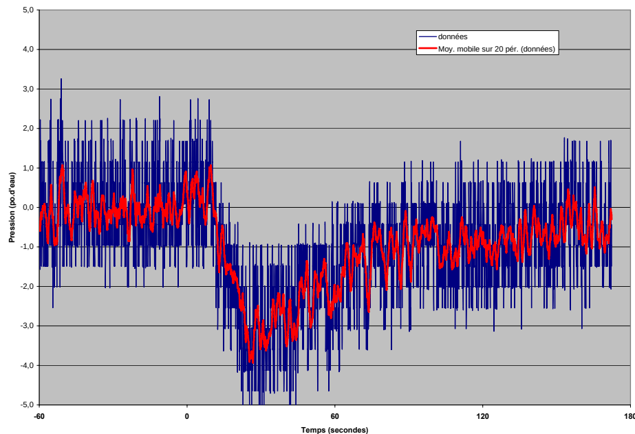
Figure 11a : Variation des pressions enregistrées au puits A-p à la suite du sautage 1B indiquant la création de vides et l'aspiration subséquente des gaz émis
