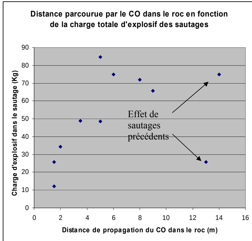
Figure 20 : Distance de propagation du CO dans le roc en fonction de la charge totale d'explosif des sautages ( R^2 = 0.63 )
