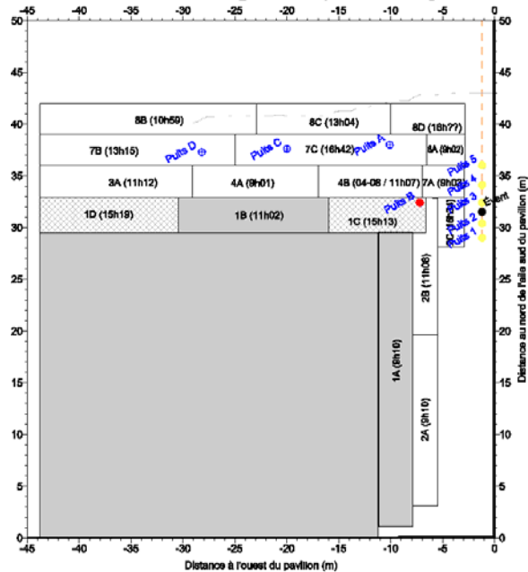
Teneur en CO dans le sol 40 @ 70 min. après les sautages 1C & 1D
