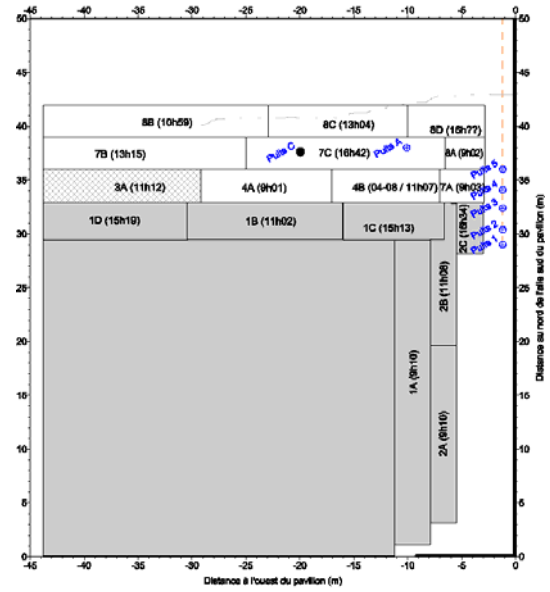
Teneur en CO dans le sol 48 min. après le sautage 3A
