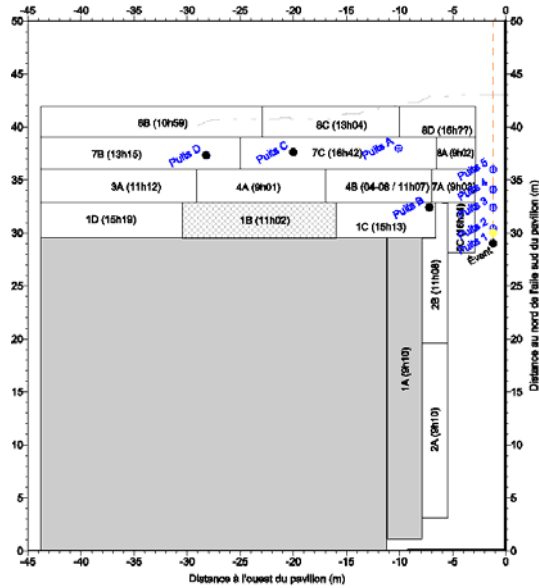
Teneur en CO dans le sol dans les 30 min. suivant le sautage 1B
