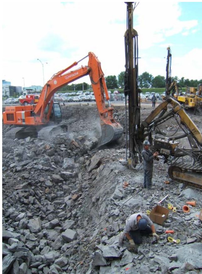
Figure 23 : Localisation typique des travailleurs lors des opérations de chantier (Après le sautage 8B)
