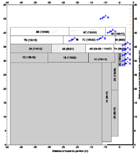
Teneur en CO dans le sol 50 @ 80 min. après le sautage 4A
