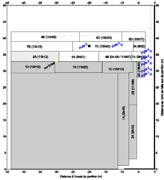
Teneur en CO dans le sol dans les 8 min. suivant le sautage 3A
