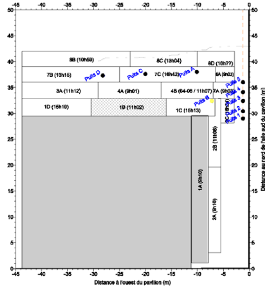
Teneur en CO dans le sol de 2h40 @ 3h20 après le sautage 1B
