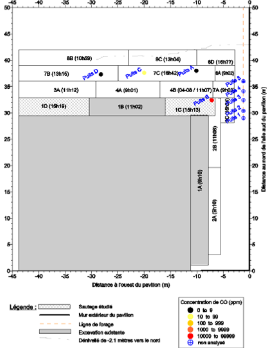
Teneur en CO dans le sol 70 @ 100 min. après les sautages 1C & 1D
