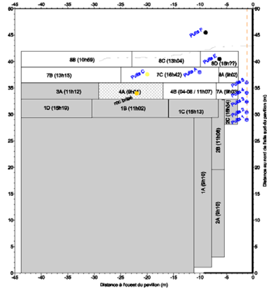
Teneur en CO dans le sol 20 @ 50 min. après le sautage 4A
