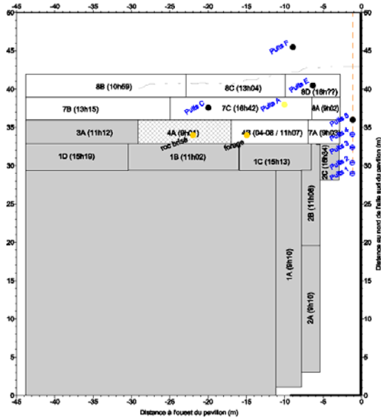
Teneur en CO dans le sol dans les 20min. suivant le sautage 4A
