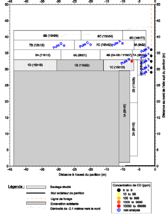
Teneur en CO dans le sol 100 @ 130 min. après les sautages 1C & 1D
