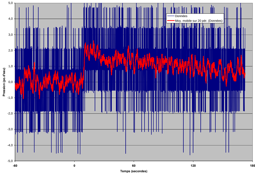
Figure 11b Variation des pressions enregistrées au puits D-p à la suite du sautage 1B indiquant une injection de gaz dans la famille de joints #1
