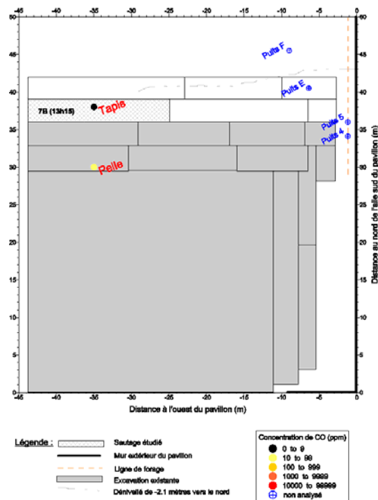
Figure 27 : Localisation de la pelle lors des travaux d'excavation du sautage 7B
