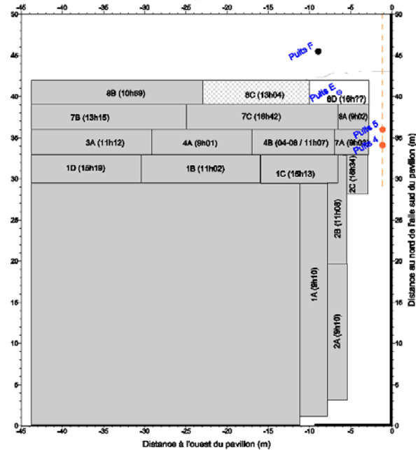
Teneur en CO dans le sol 3 @ 4 heures après le sautage 8C
