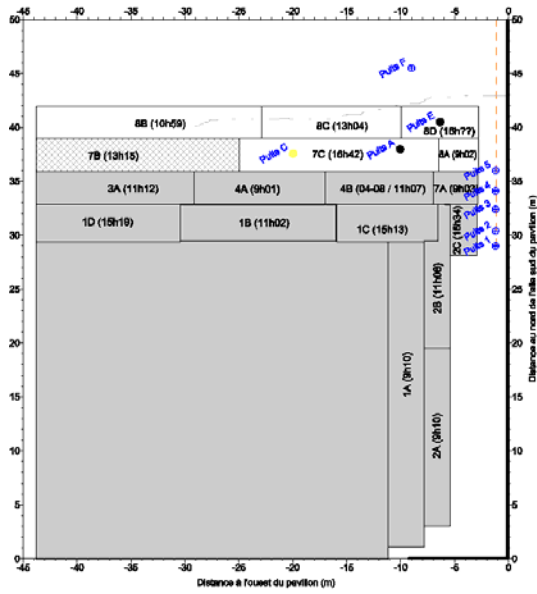
Teneur en CO dans le sol dans les 30 min. suivant le sautage 7B
