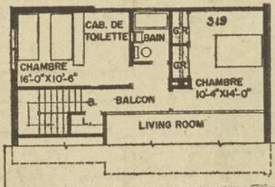
PLAN DU SECOND ÉTAGE
