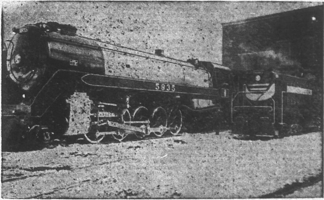
La 5935, locomotive du type "Selkirk", pour transport mixte dans les Rocheuses, dont M. N.-R. Crump, vice-président du Pacifique Canadien, a reçu livraison, hier, au nom de la compagnie, aux usines de la Montreal Locomotive Works, à Montréal-Est. Cette puissante machine sera vraisemblablement la dernière locomotive à vapeur construite pour le C.P.R. A l'avenir, le matériel de traction de cette compagnie sera constitué exclusivement de locomotives diésels. A droite, on voit précisément une diésel pour manoeuvres d'aiguillage dans les cours de triage, construite également à la Montreal Locomotive Works et dont le C.P.R. a aussi reçu livraison hier. (Nouvelle en page 6)
