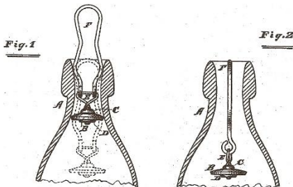
Dessins démontrant le dispositif de fermeture. Fig n° 1. Dispositif fermé Fig n° 2. Dispositif ouvert
