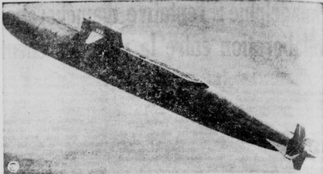
• DESTRUCTEUR DE SOUS-MARINS — Dessin d'artiste du "Tullibee", le premier sous-marin conçu spécialement pour faire la lutte à ses semblables. C'est un bâtiment mù par l'énergie nucléaire, dont la mission consistera à rechercher et à détruire des sous-marins ennemis sous la surface des mers. Le "Tullibee" ne mesure que 260 pieds et il est présentement construit aux chantiers de General Dynamics de Groton, au Connecticut. Son déplacement sera de 2.175 tonnes, ce qui en fera le plus petit sous-marin atomique jamais construit. (N.E.A.)
