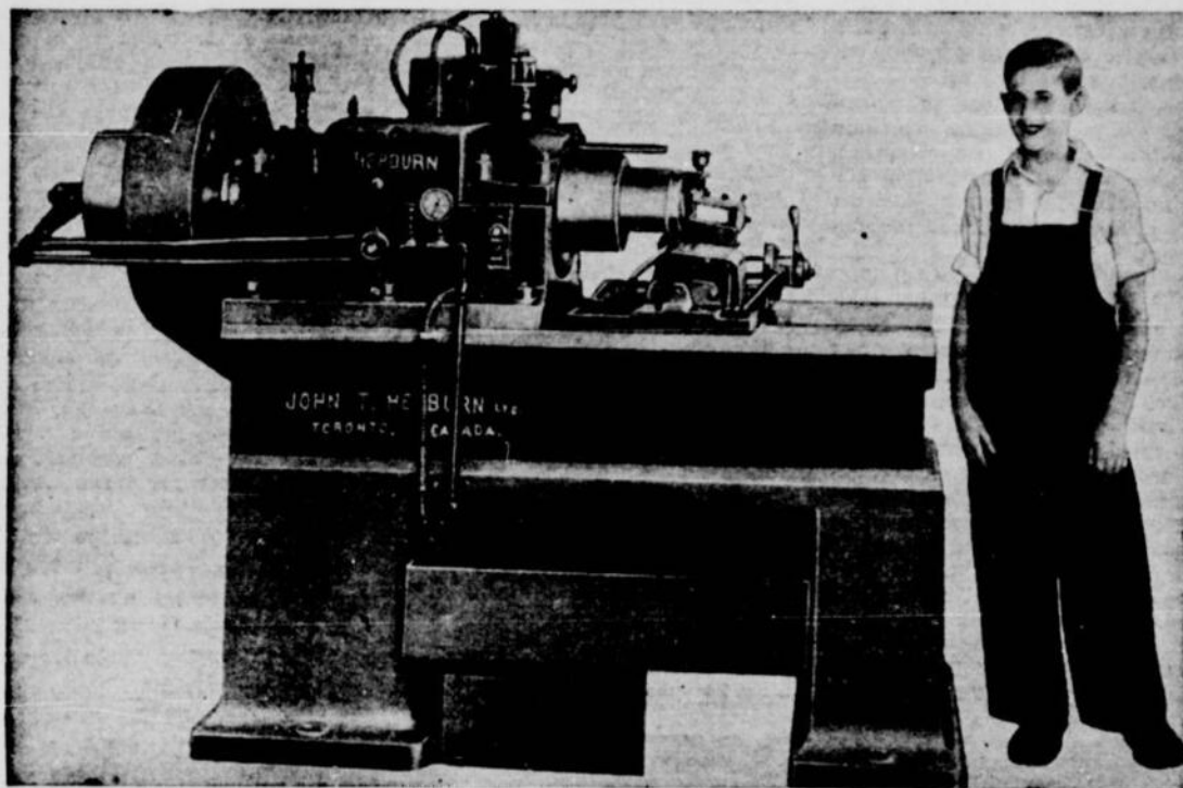
Les machines de M. Hepburn sont si simples qu'un garçon ou une jeune fille peuvent les manoeuvrer. Voici l'une des anciennes machines-outils et James-Forgan Hepburn, fils de John-T. Hepburn, âgé de 16 ans.
