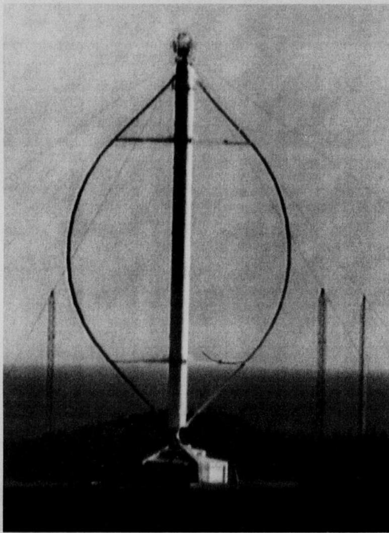
L'éolienne de Cap-Chat mesure 110 mètres de hauteur (un immeuble de 30 étages). Elle produit 4 mégawatts par heure d'électricité et peut alimenter plus de 400 familles.
