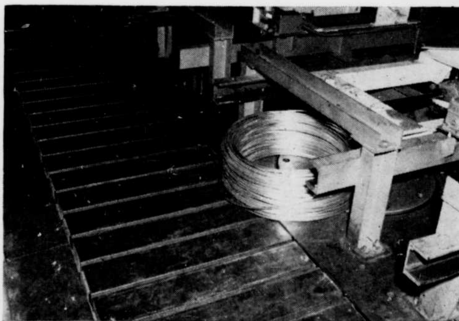
Enroulement terminé. La tige est poussée hors de la roue à chevilles (Pin-reels), et placée sur un transporteur.
