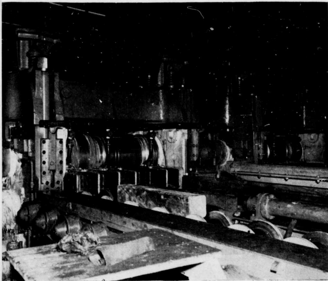
Le près d'une pièce d'aluminium subissant la première opération du dégrossisseur (Roughing-mill).
