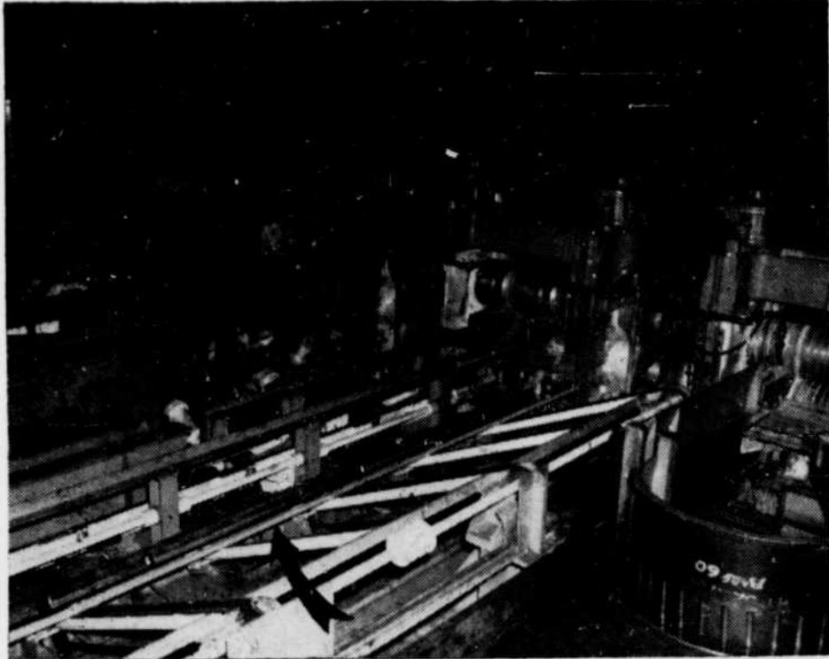
Autre phase d'opération. La tige d'aluminium est transportée à la dernière passe du dégrossisseur. La flèche indique la tige.
