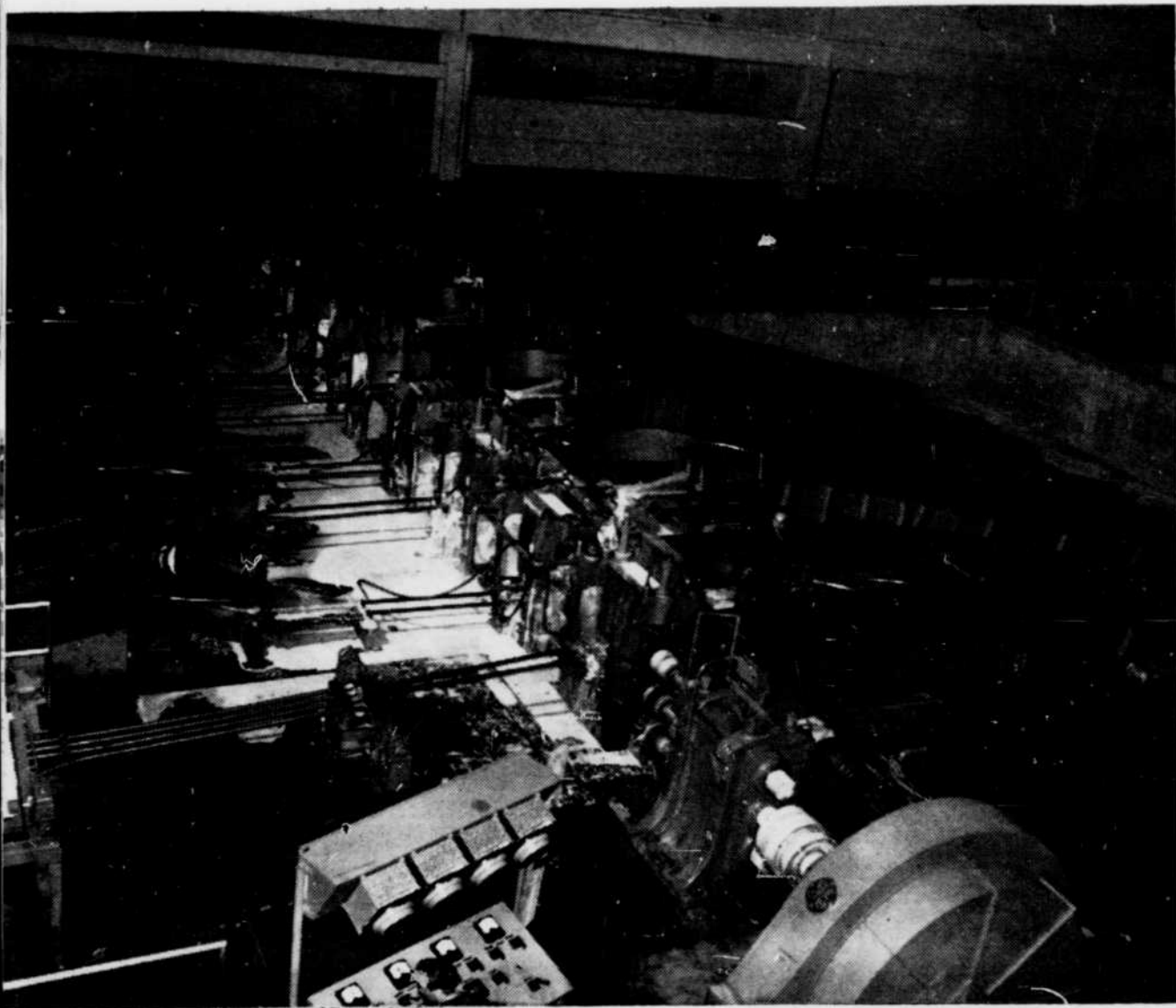
Vue d'ensemble du laminoir de finissage (Finishing-mill). On remarquera la tige complètement bou-
