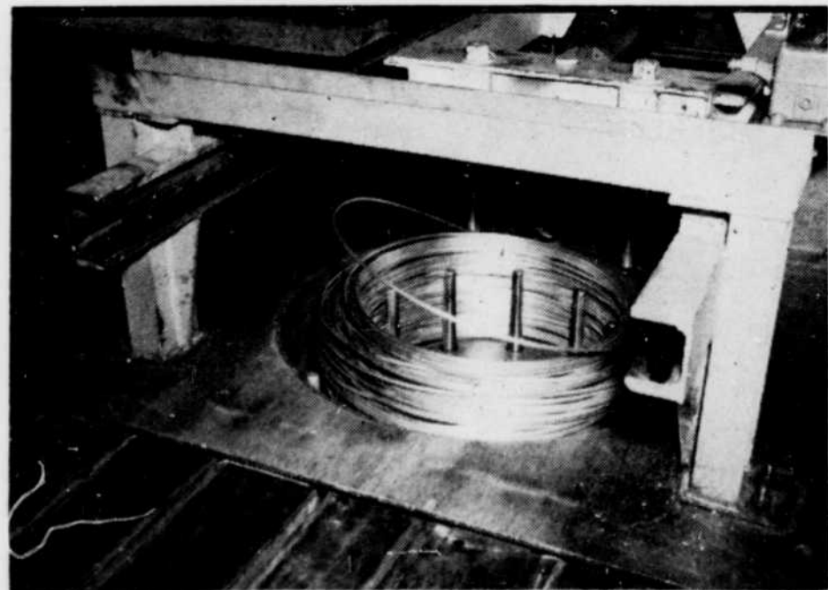
La tige complétée s'enroulant automatiquement sur une roue à chevilles.
