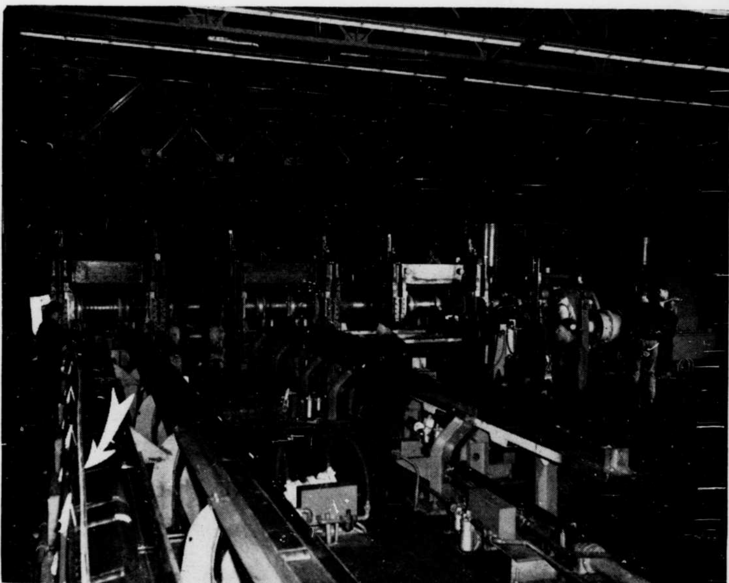
Vue d'ensemble du dégrossisseur (Roughing-mill). On remarquera sur la rampe de gauche la tige d'aluminium se rendant au laminoir de finissage. La flèche indique la tige.
