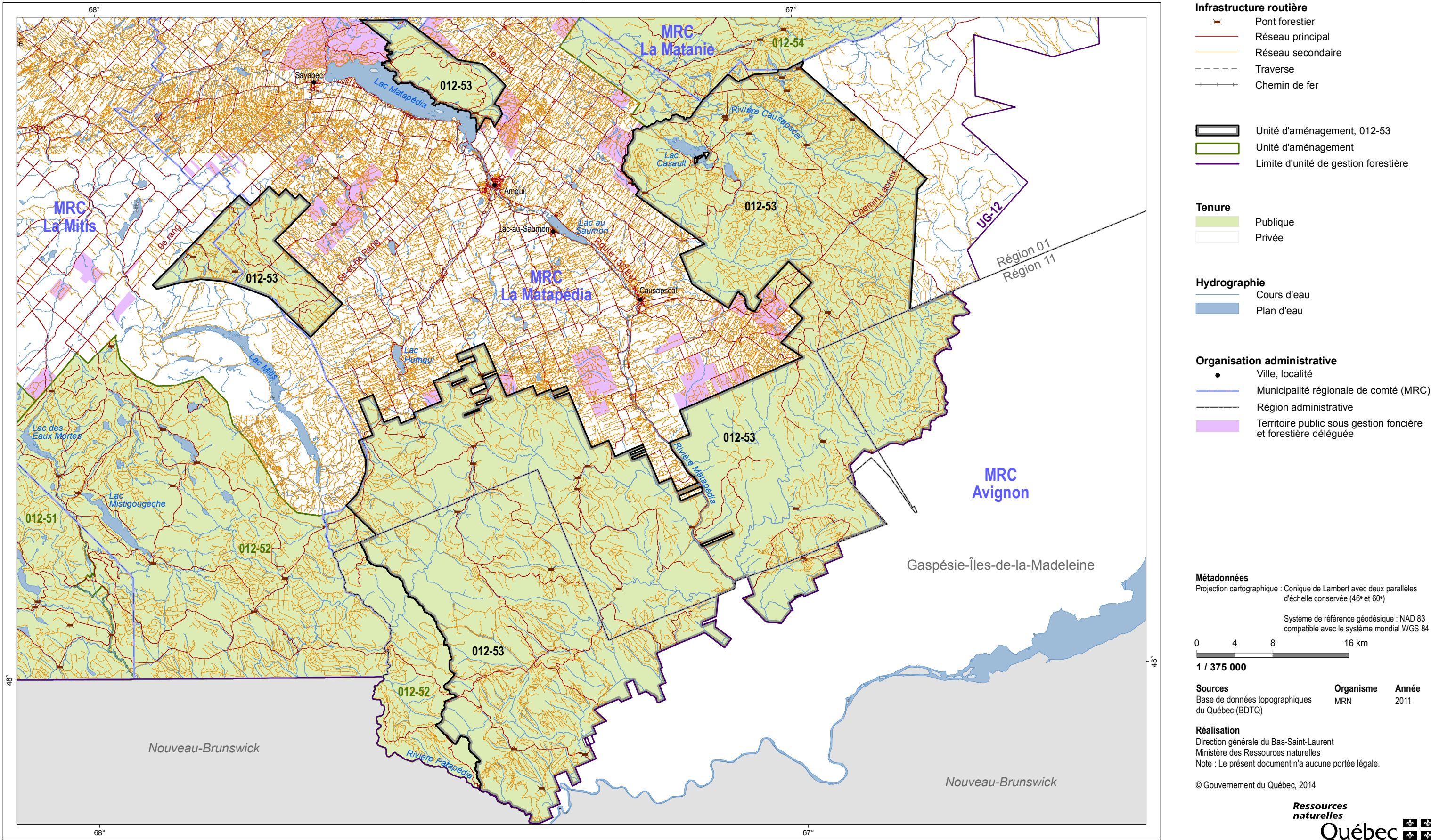
Figure 3 : Infrastructure routière existante Unité d'aménagement 012-53
