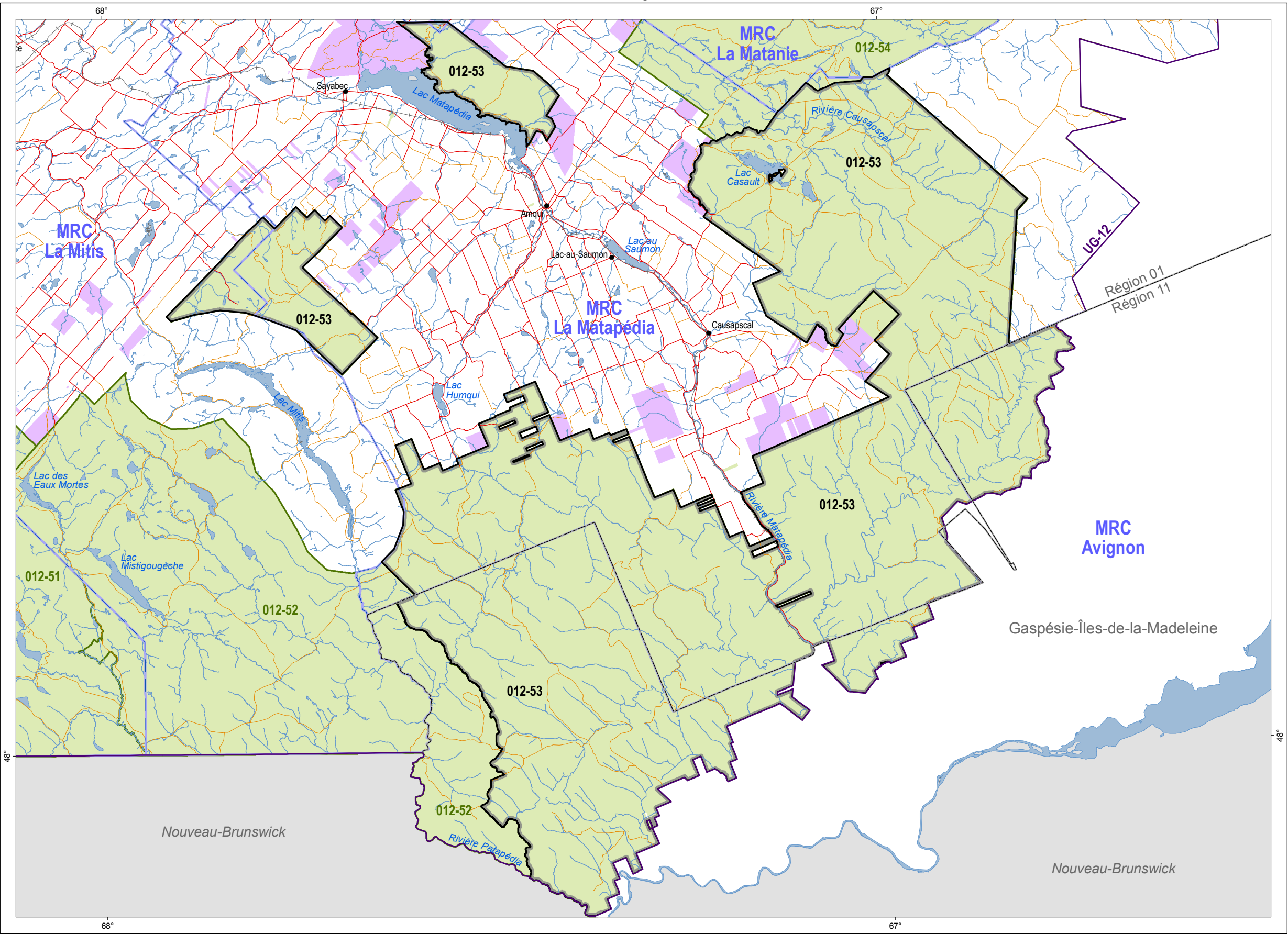
Figure 14 : Épidémie de l'arpenteuse de la pruche Unité d'aménagement 012-53
