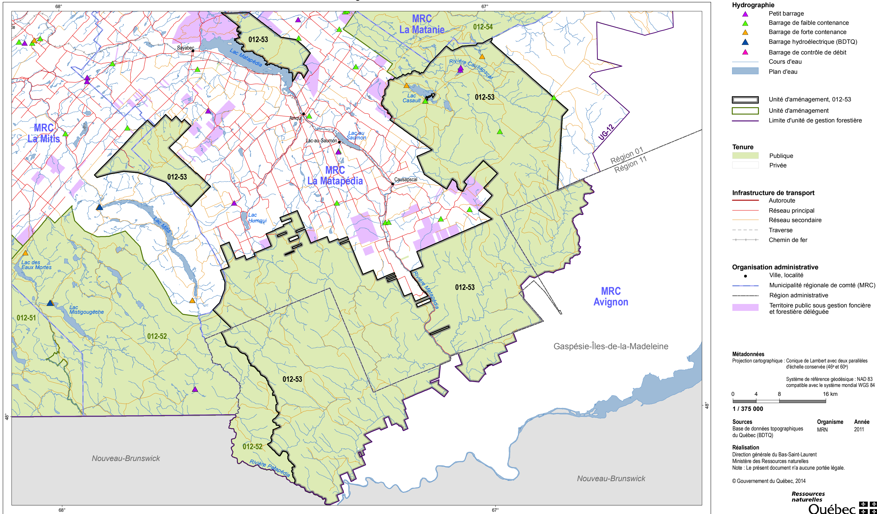
Figure 2 : Réseau hydrographique et aménagement hydrique Unité d'aménagement 012-53
