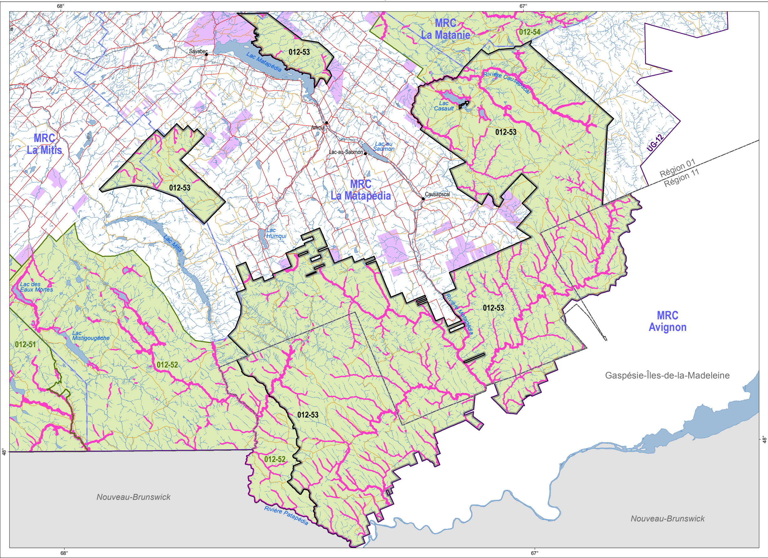
Figure 26 : Bande riveraine sans intervention Unité d'aménagement 012-53
