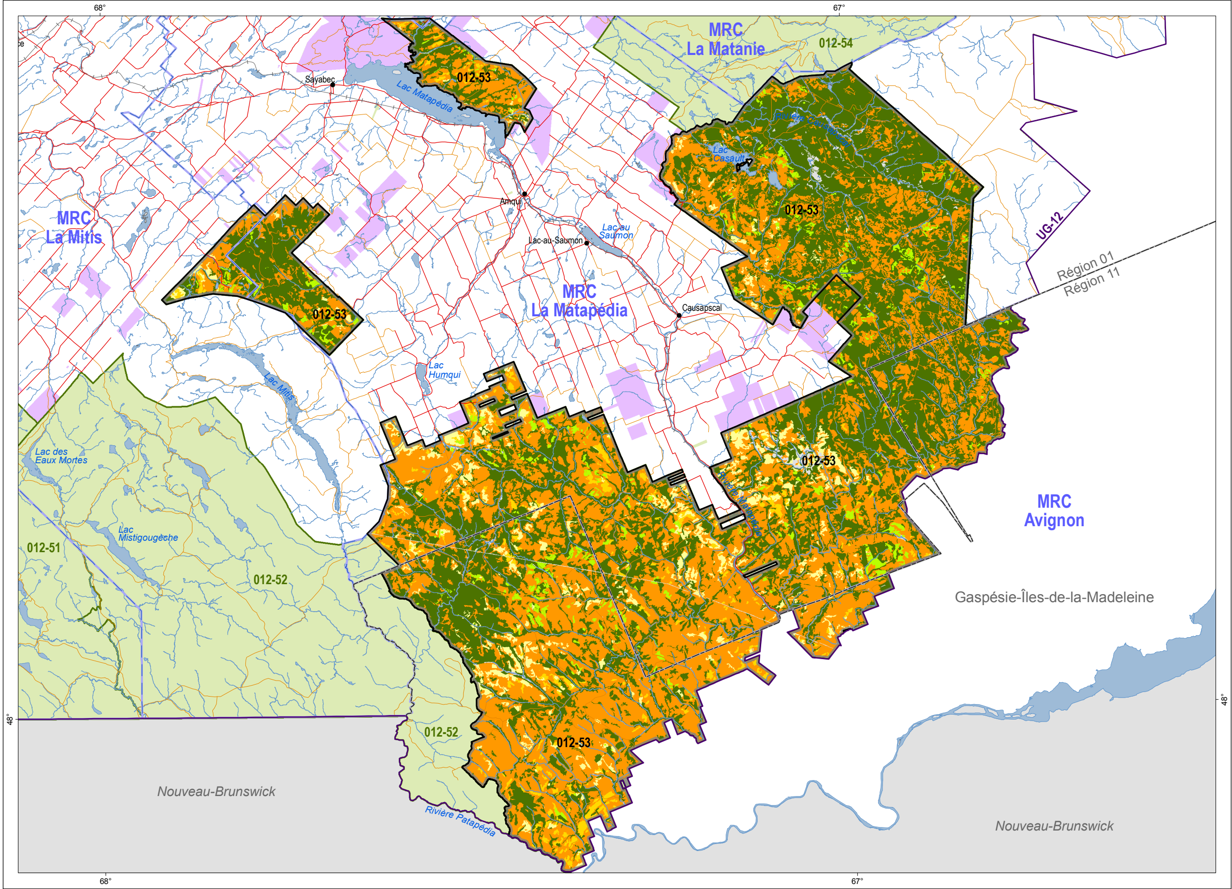
Figure 11 : Type de couvert forestier Unité d'aménagement 012-53
