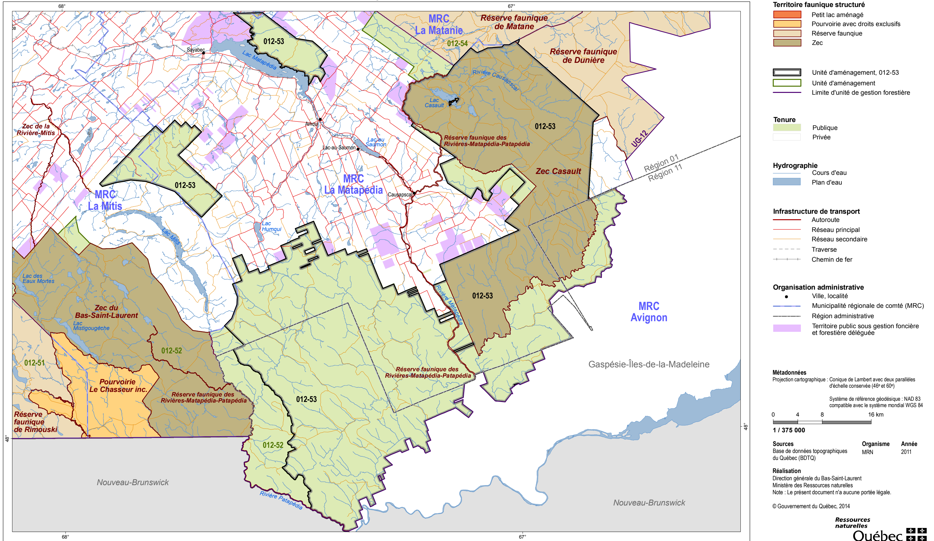
Figure 18 : Territoire faunique structuré Unité d'aménagement 012-53
