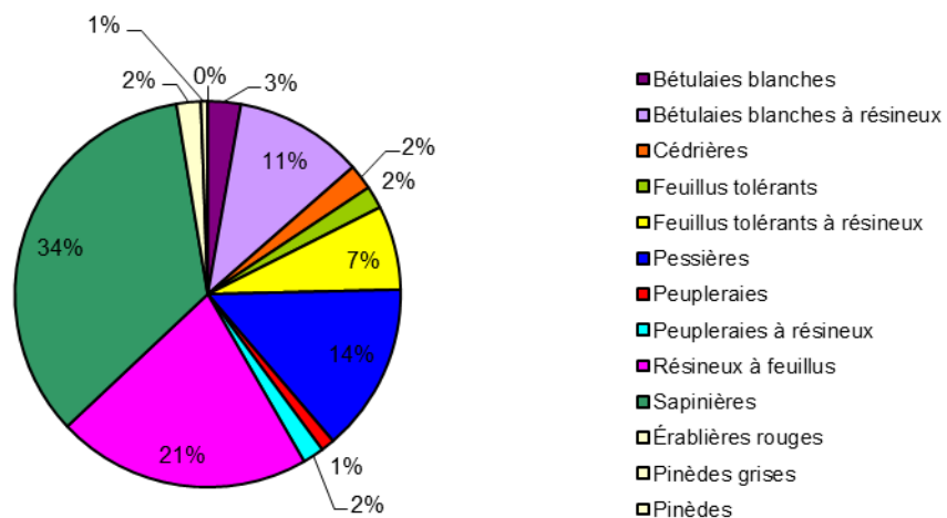
Figure 13 : Proportions des grands types de forêts
