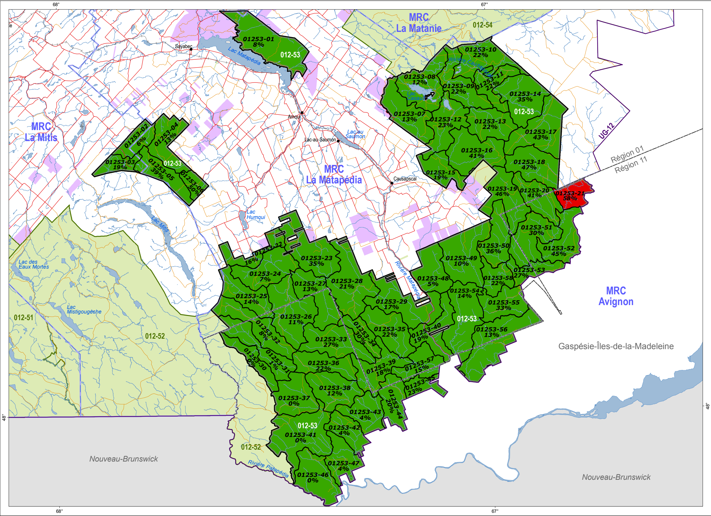
Figure 31 : Proportion de la forêt de moins de 20 ans (habitat de l'orignal)
