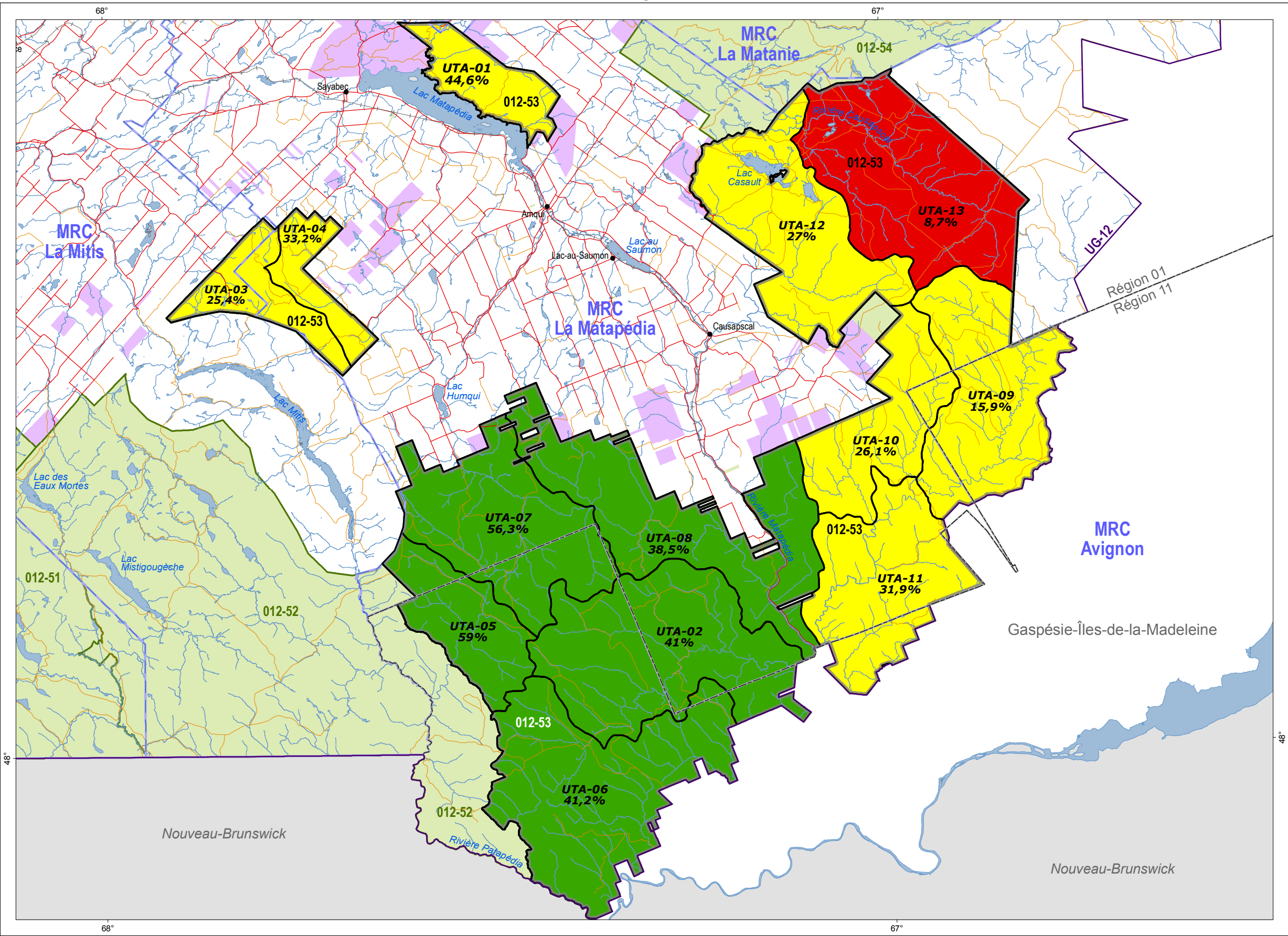
Figure 27 : Altération de la forêt d'intérieure Unité d'aménagement 012-53
