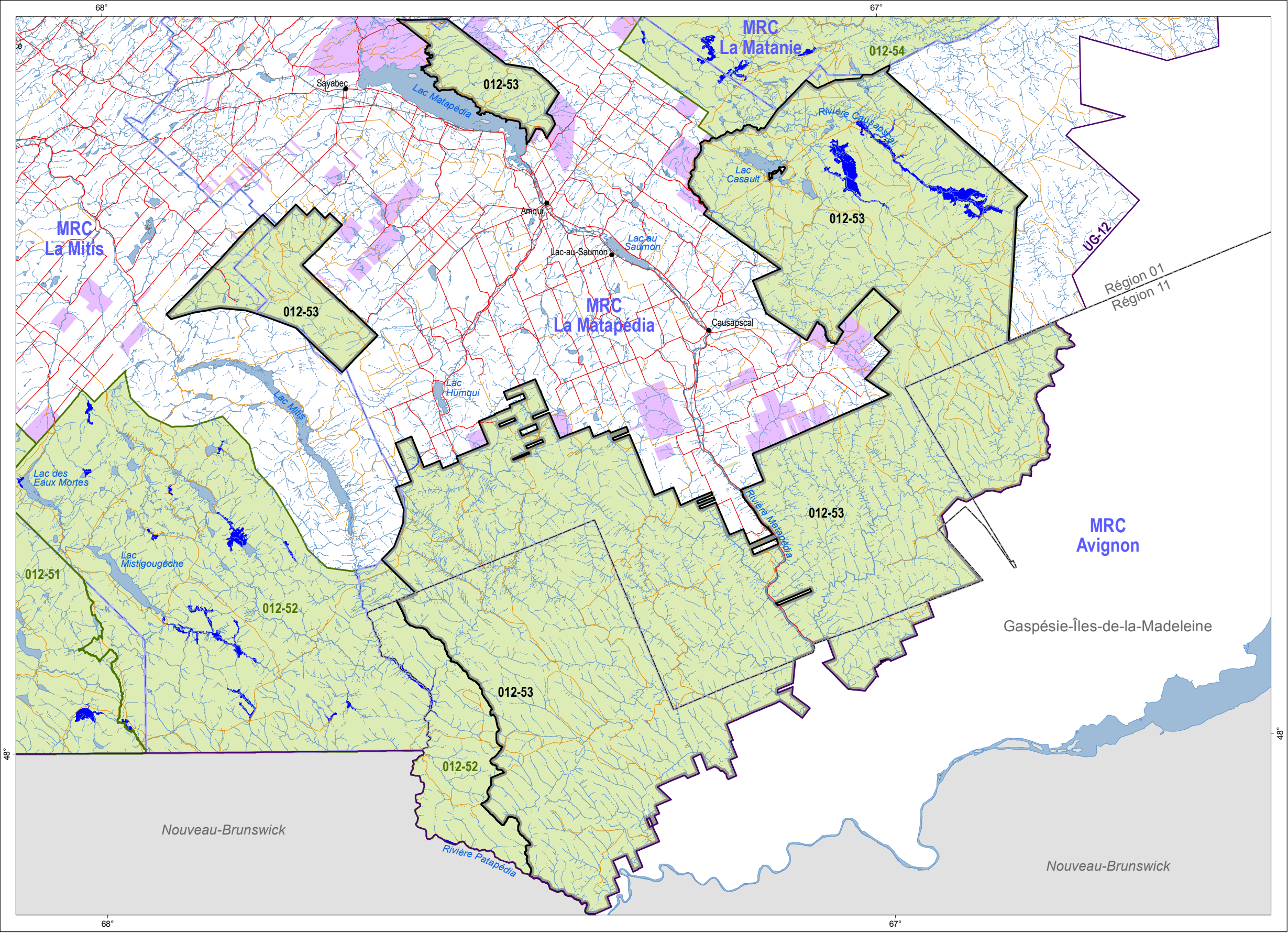
Figure 25 : Milieu humide d'intérêt Unité d'aménagement 012-53
