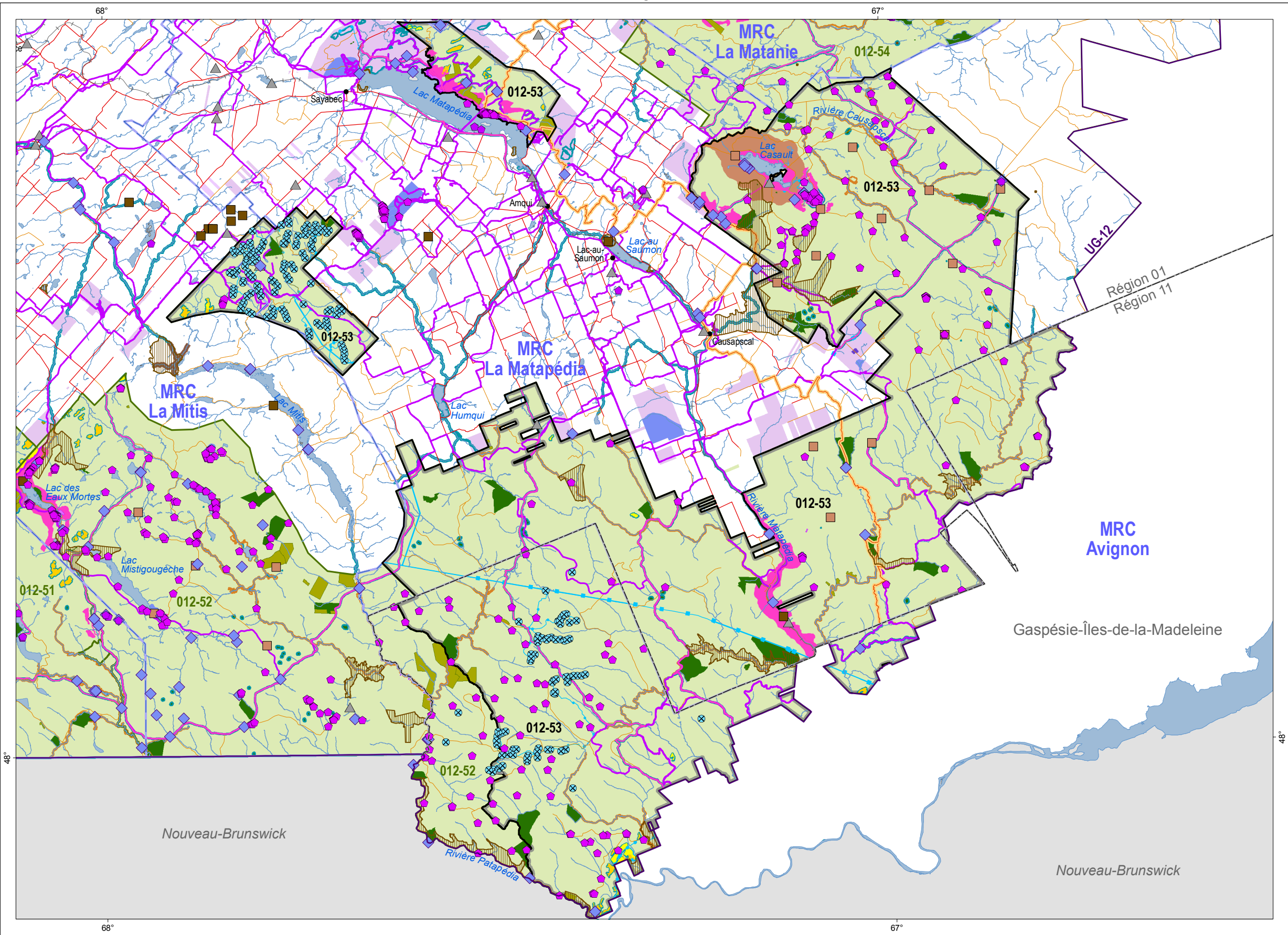
Figure 5 : Usage forestier et zone d'application avec modalité d'intervention (ZAMI) Unité d'aménagement 012-53
