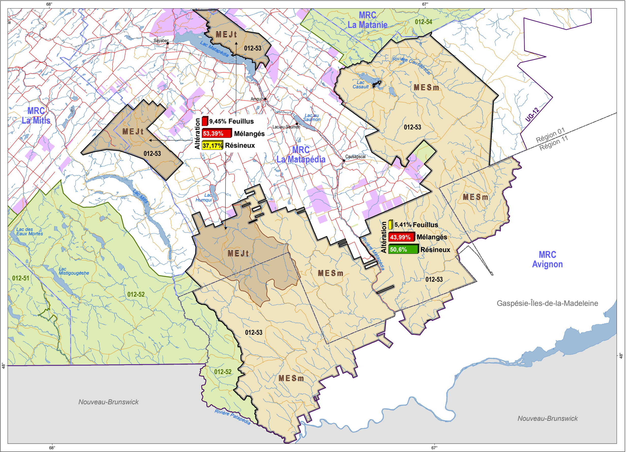
Figure 24 : Altération selon le type de couvert forestier Unité d'aménagement 012-53
