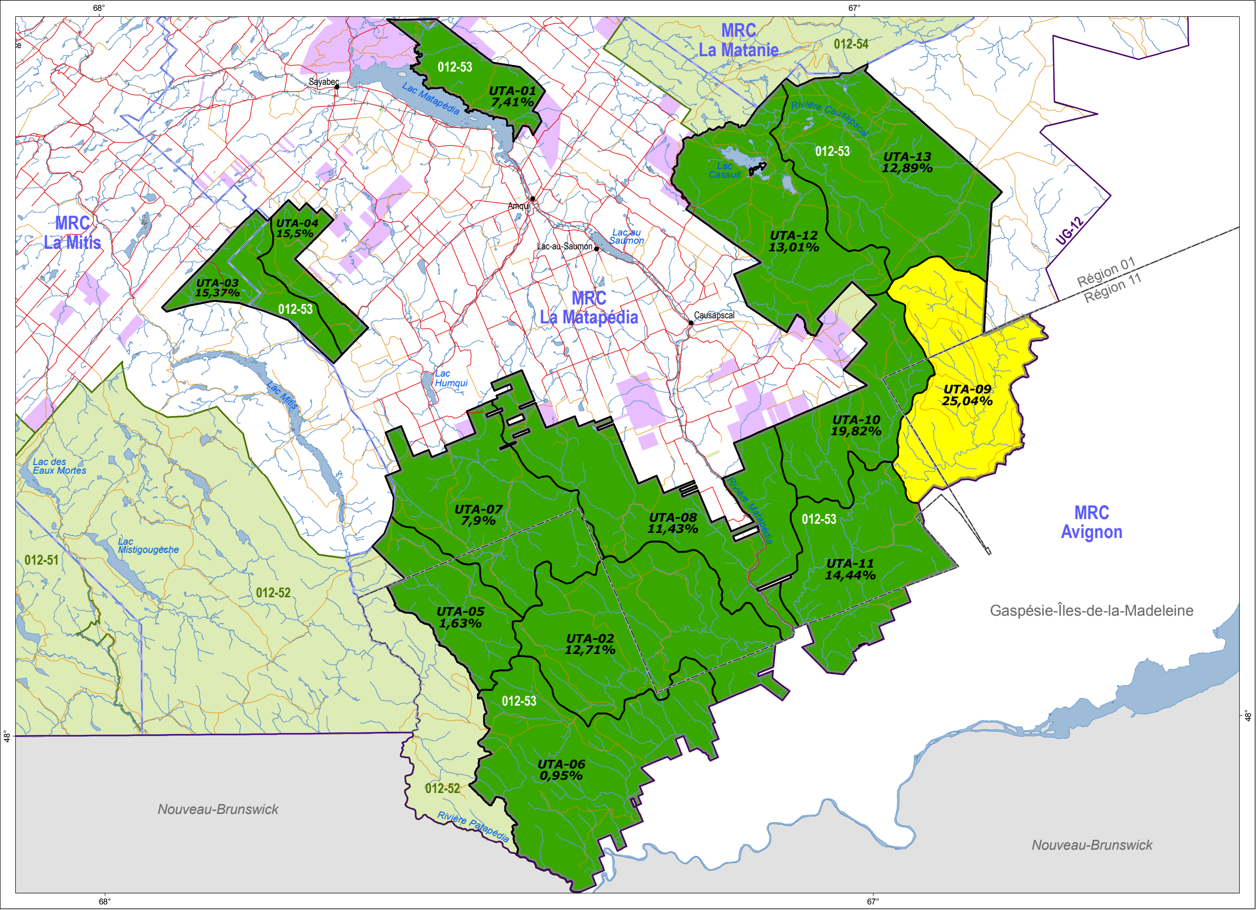
Figure 21 : Altération de la structure d'âge (jeune forêt) Unité d'aménagement 012-53
