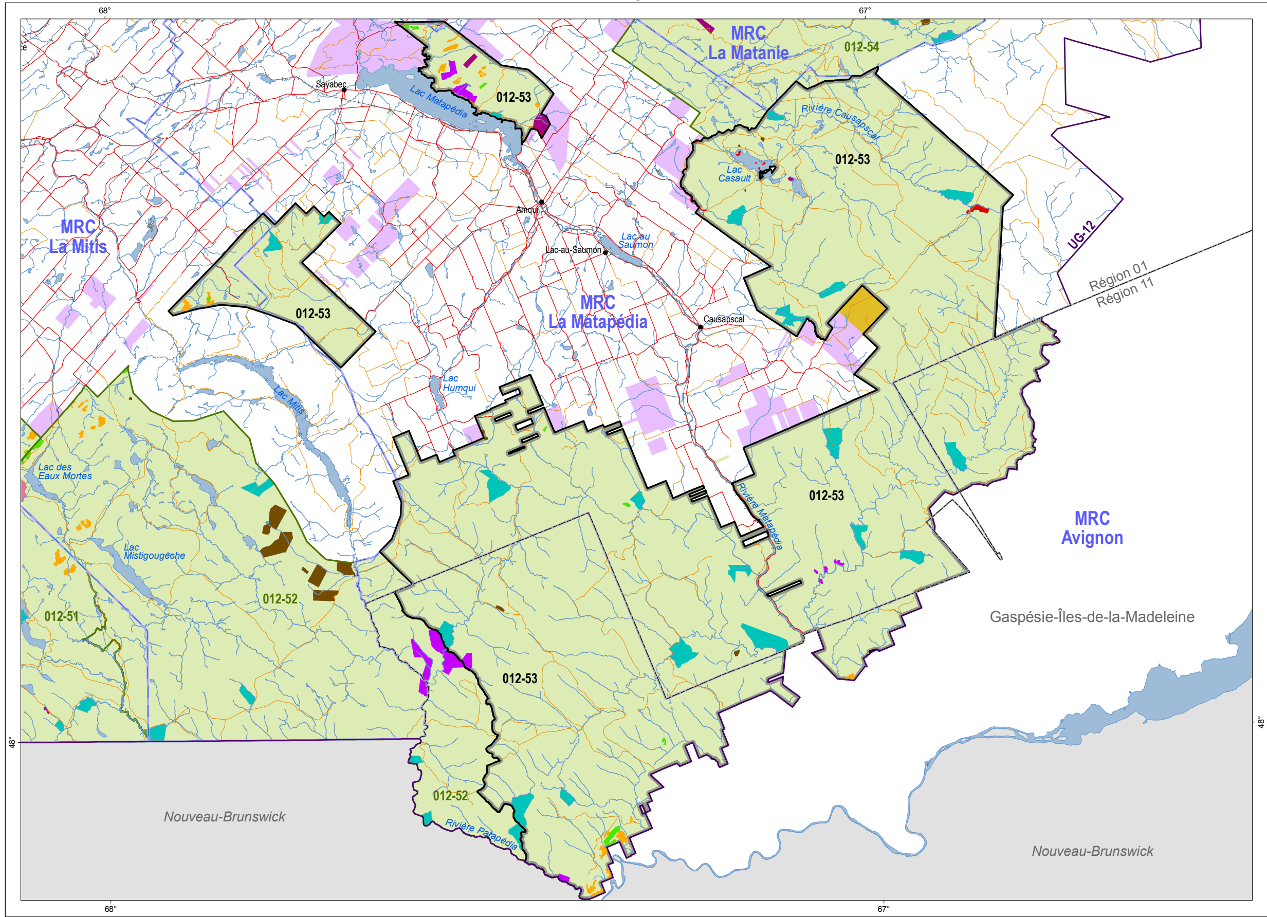
Figure 4 : Mode de gestion Unité d'aménagement 012-53
