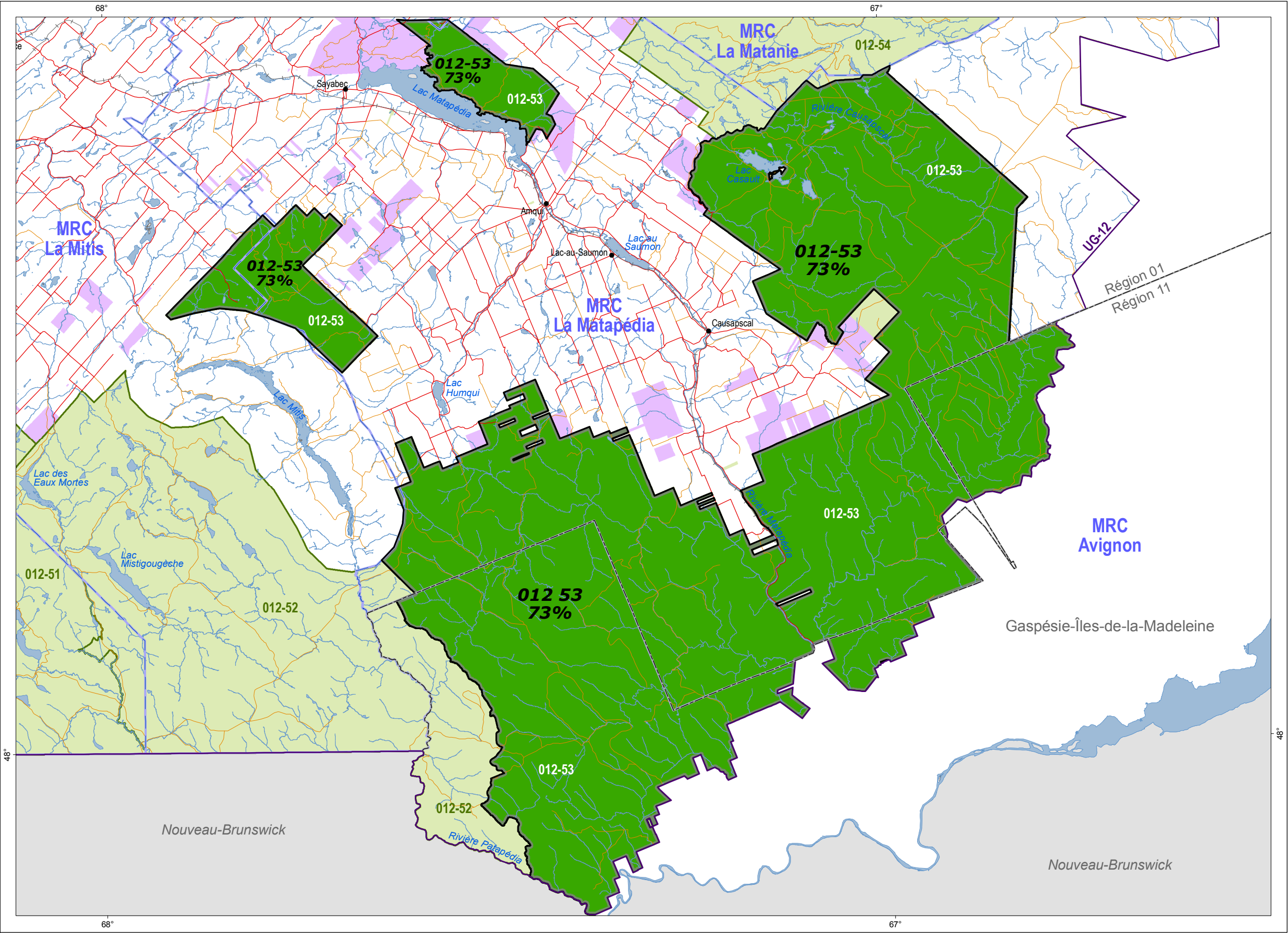
Figure 28 : Proportion de la forêt de 7 mètres et plus Unité d'aménagement 012-53
