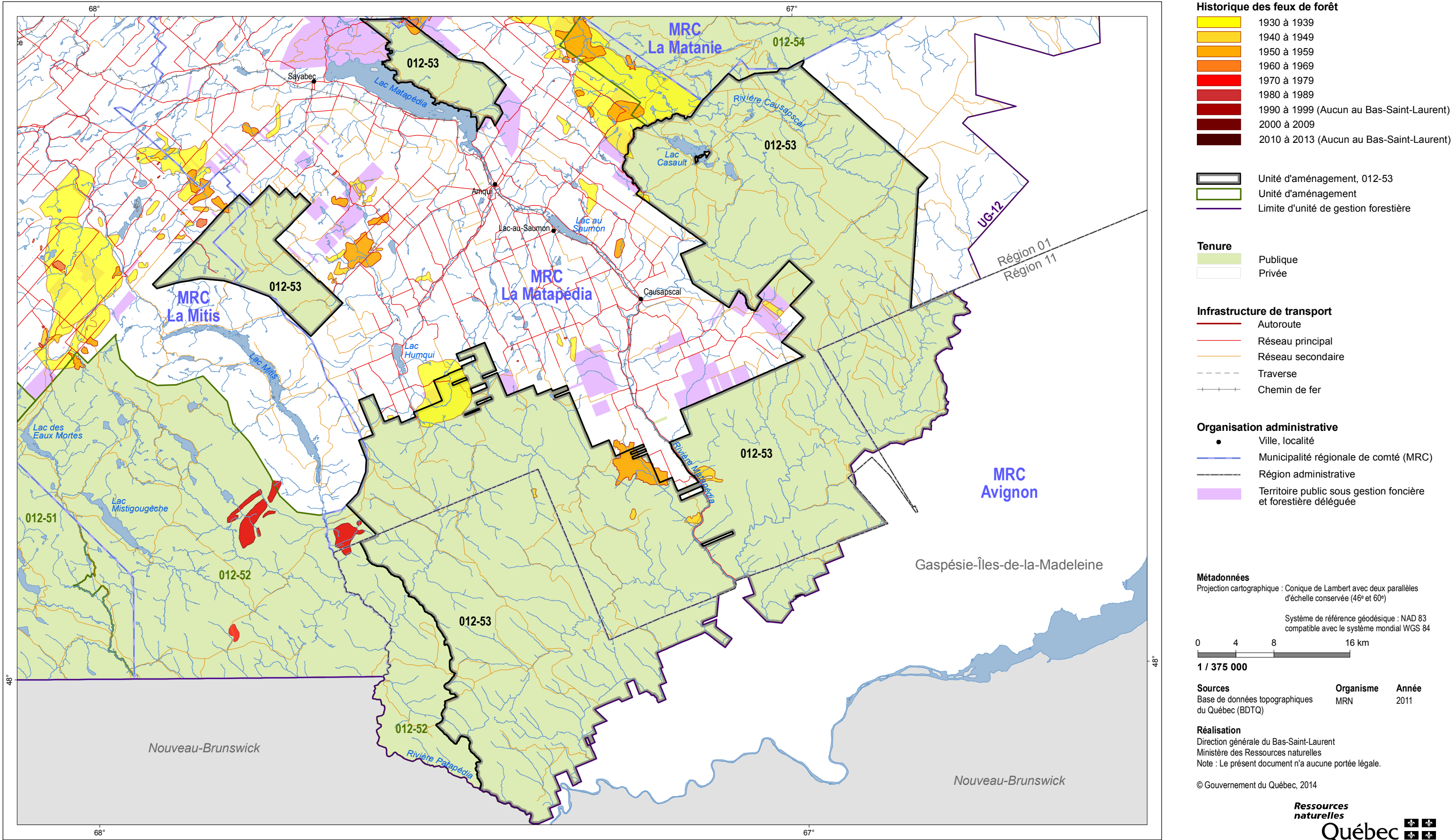
Figure 16 : Historique des feux de forêt entre 1920 et 2013 Unité d'aménagement 012-53
