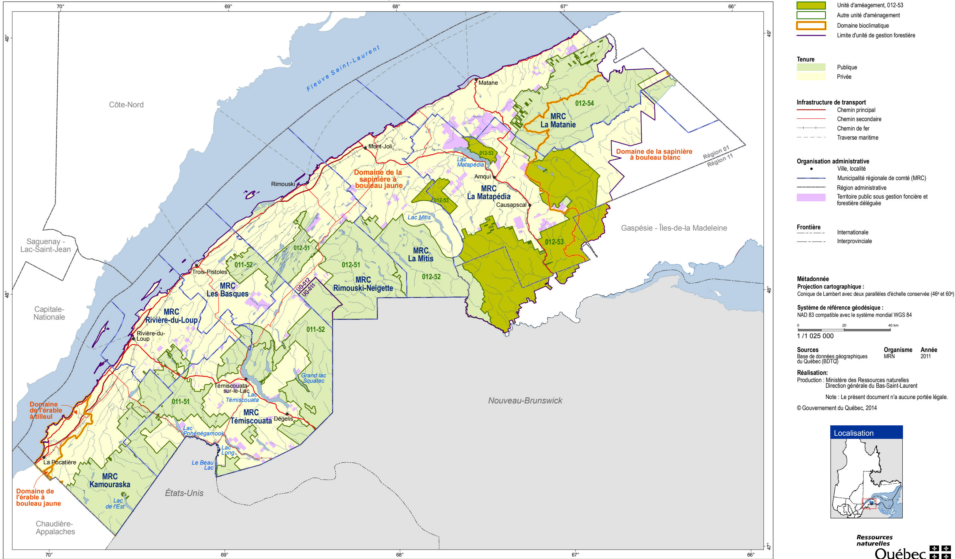
Figure 1 : Localisation de l'unité d'aménagement Unité d'aménagement 012-53
