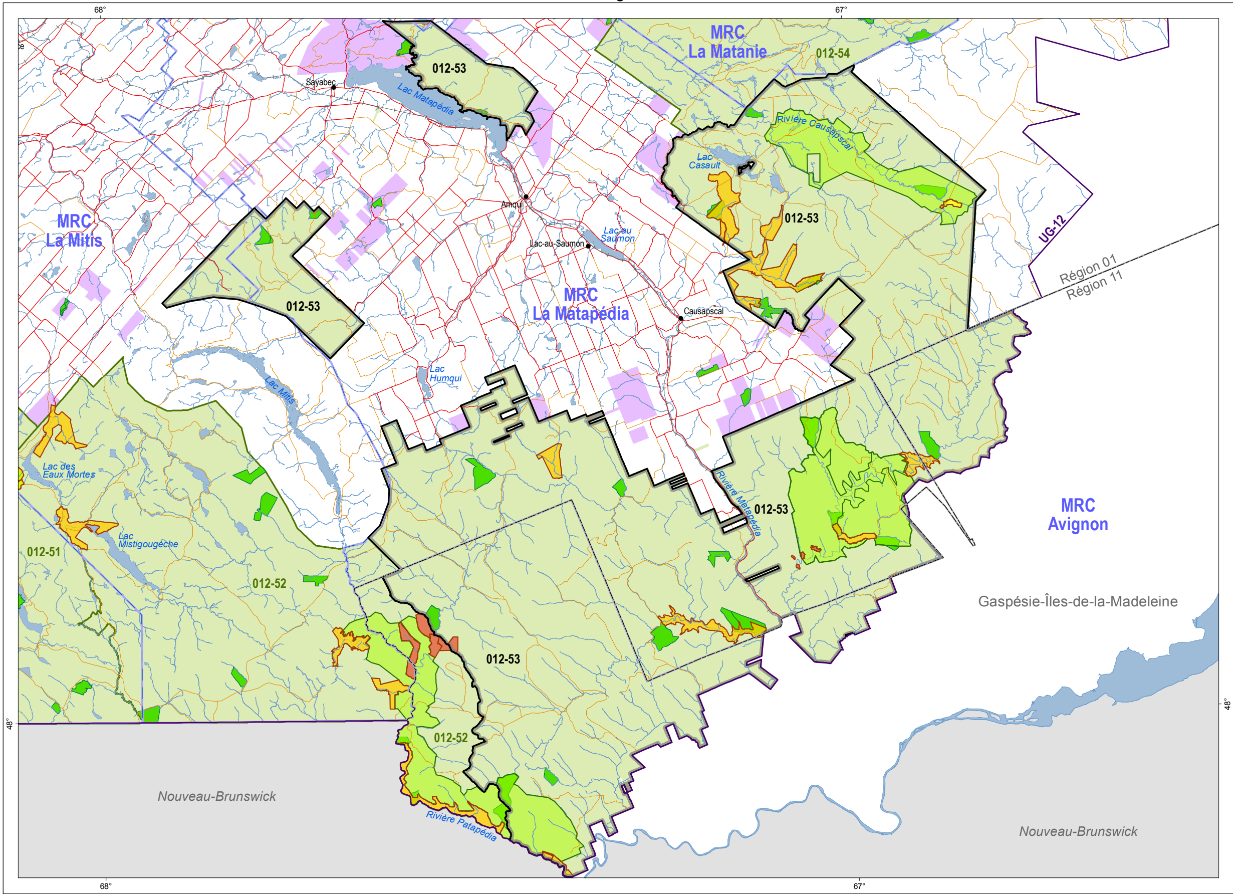
Figure 6 : Aire protégée Unité d'aménagement 012-53
