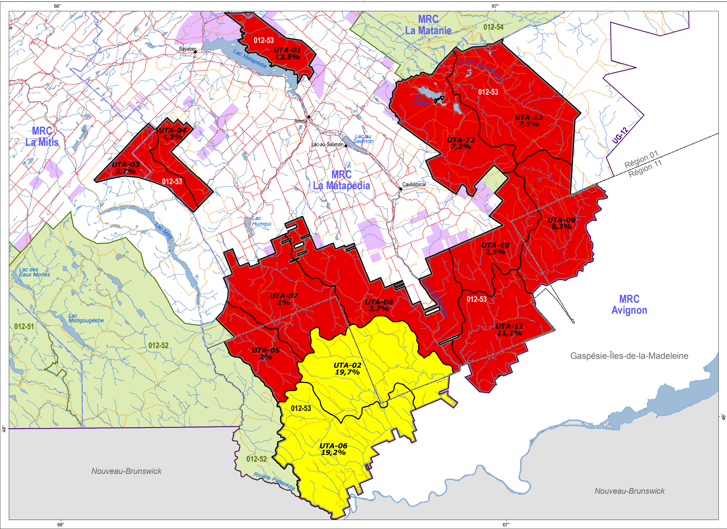
Figure 22 : Altération de la structure interne des peuplements (vieille forêt irrégulière) Unité d'aménagement 012-53
