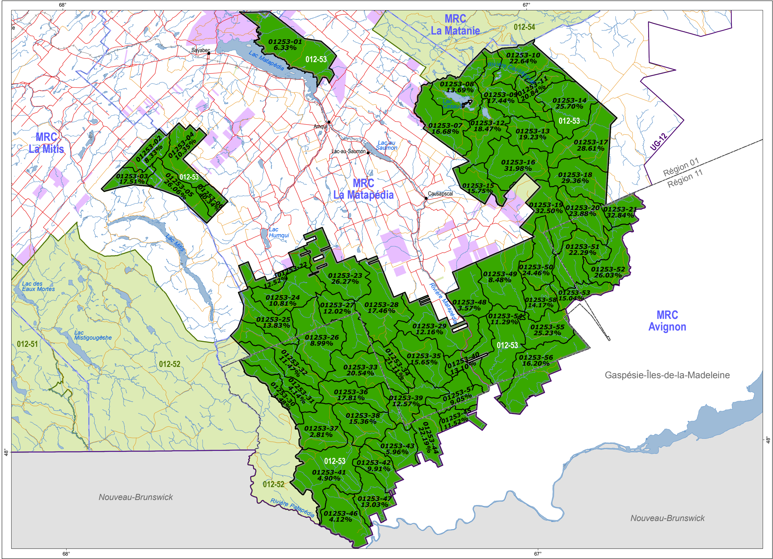
Figure 30 : Aire équivalente de coupe Unité d'aménagement 012-53
