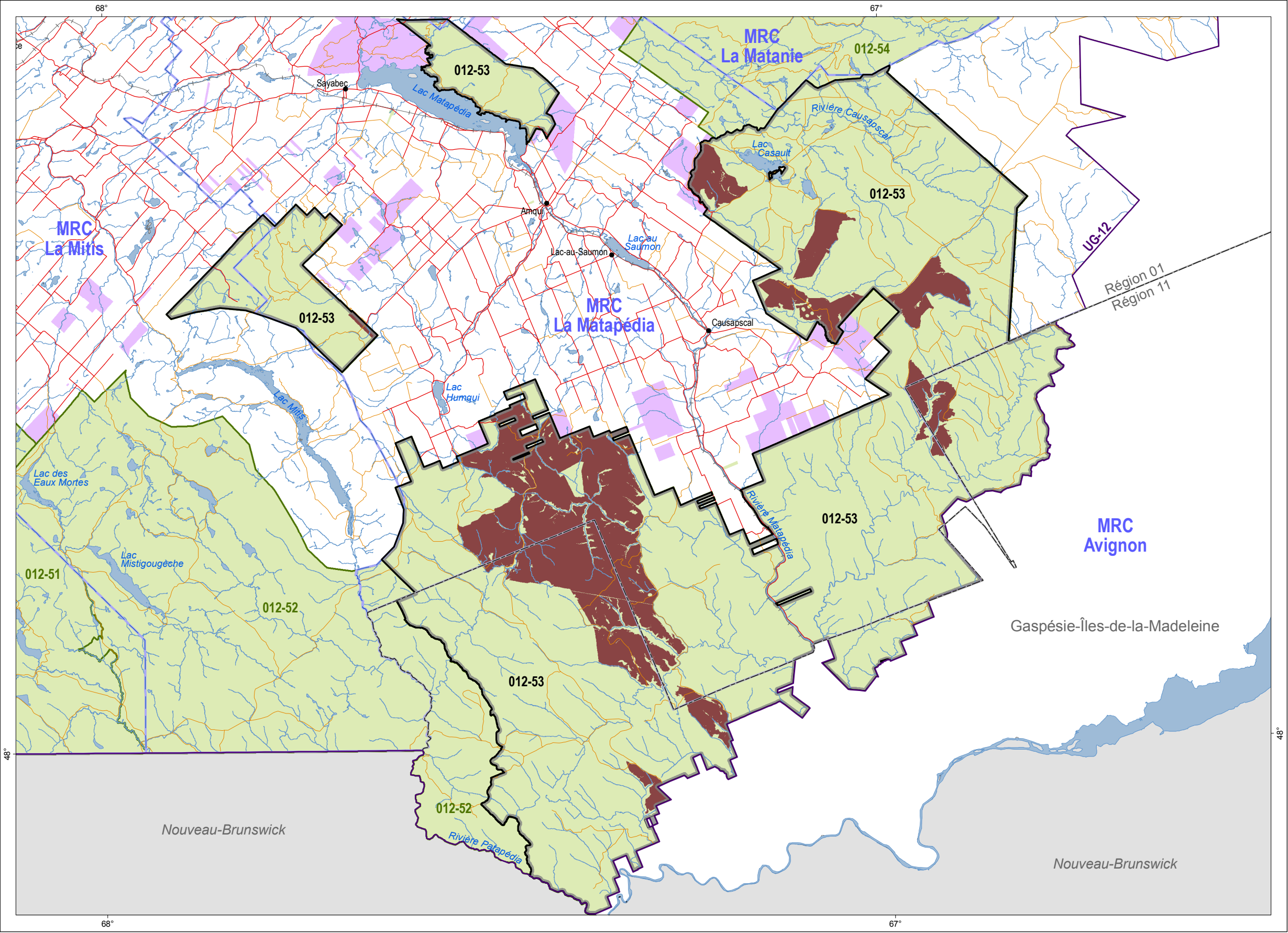
Figure 32 : Aire d'intensification de la production ligneuse Unité d'aménagement 012-53
