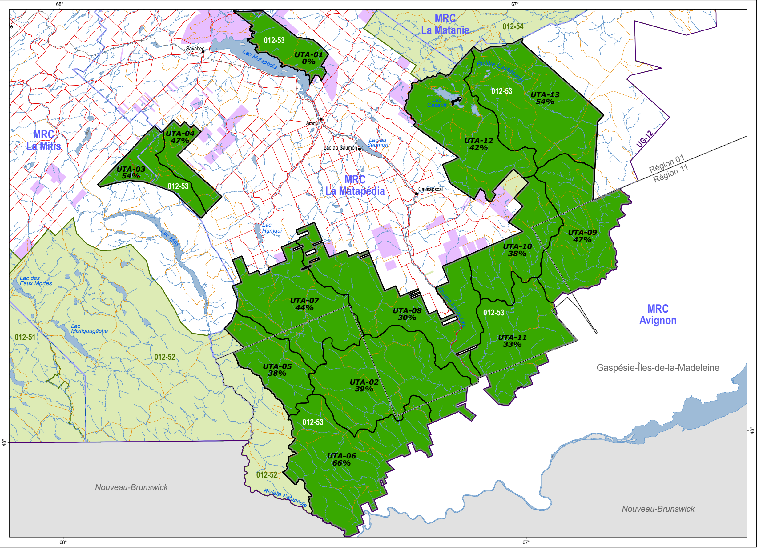
Figure 23 : Altération de la structure interne des peuplements (jeune forêt éduquée) Unité d'aménagement 012-53
