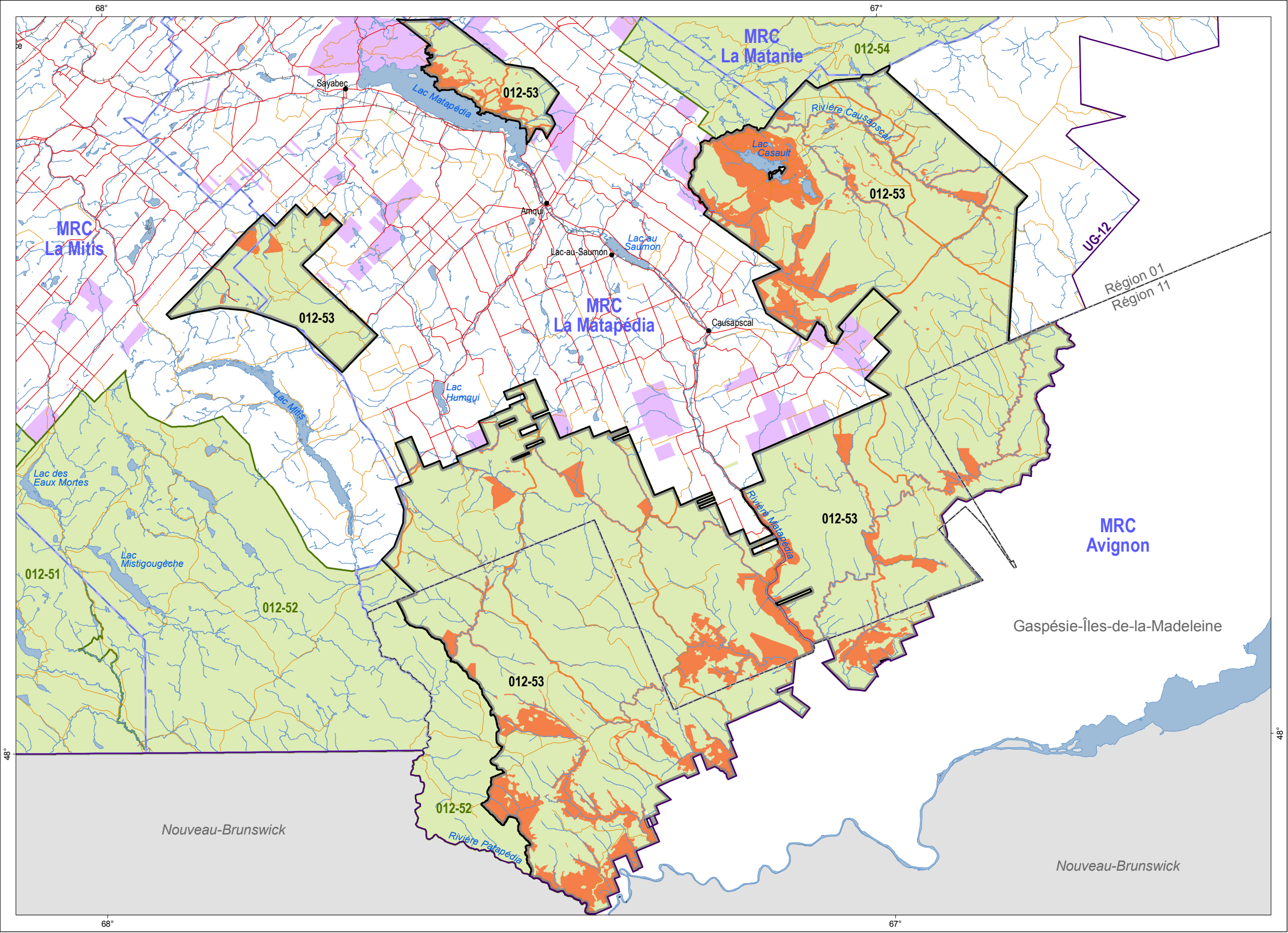
Figure 7 : Forêt à haute valeur de conservation (FHVC) Unité d'aménagement 012-53
