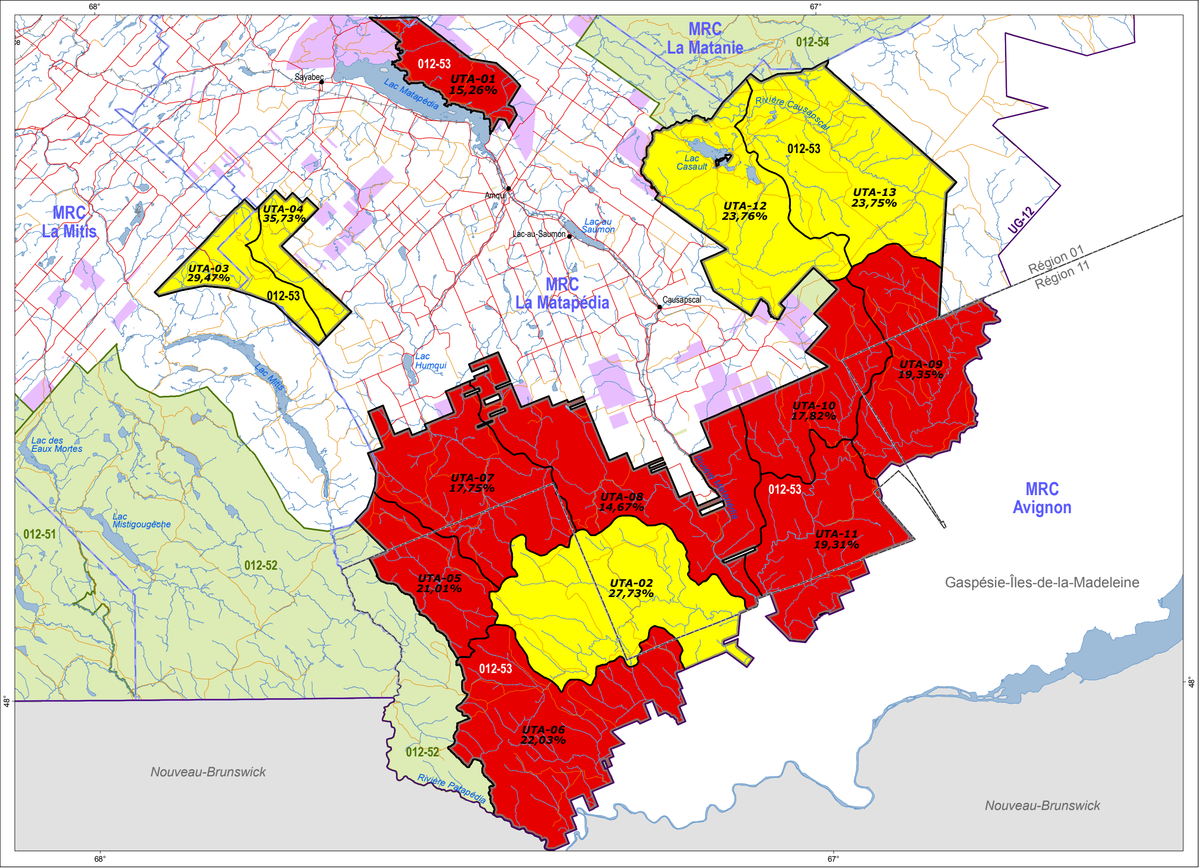
Figure 20 : Altération de la structure d'âge (vieille forêt) Unité d'aménagement 012-53
