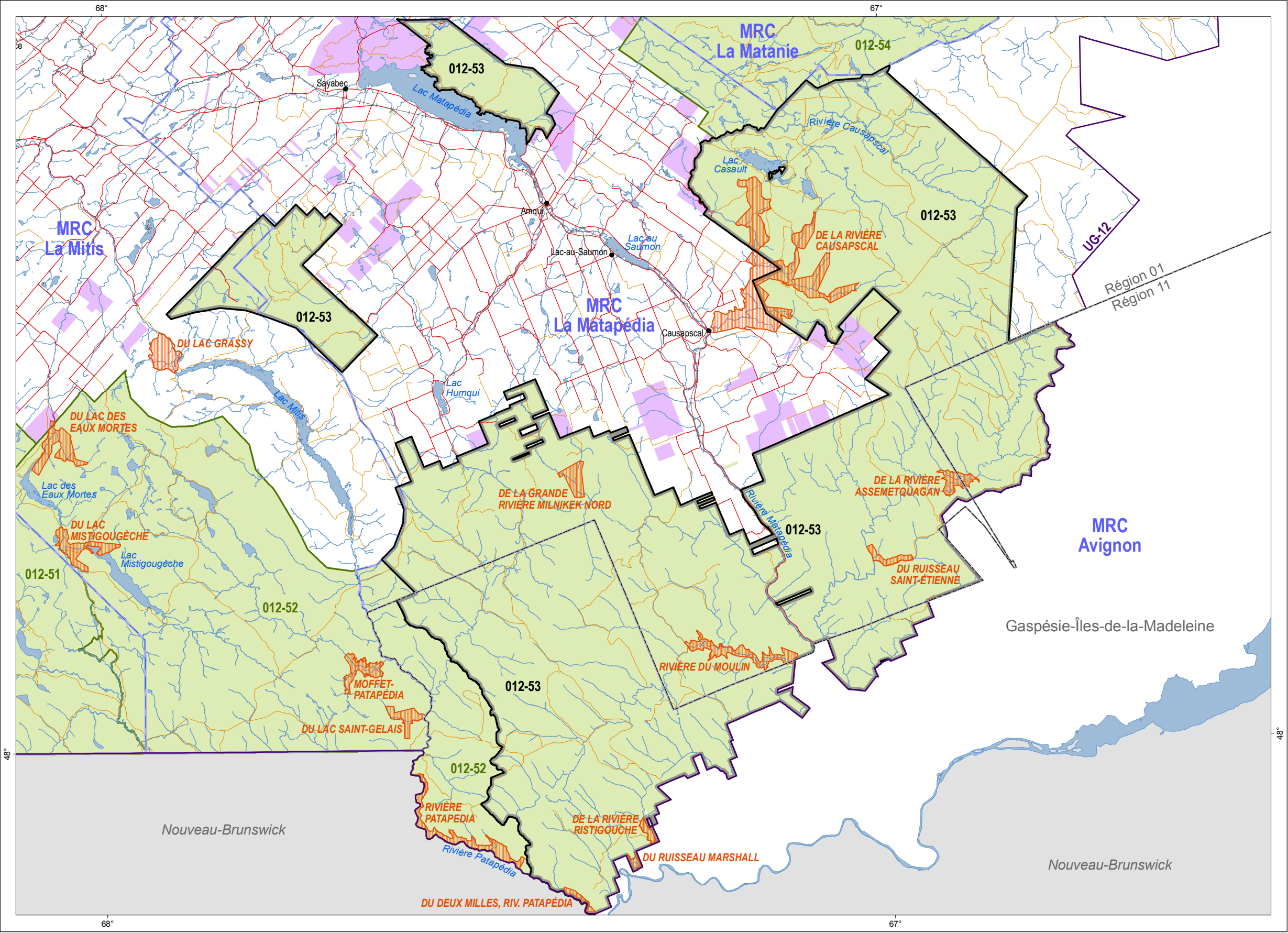
Figure 19 : Aire de confinement du cerf de Virginie Unité d'aménagement 012-53
