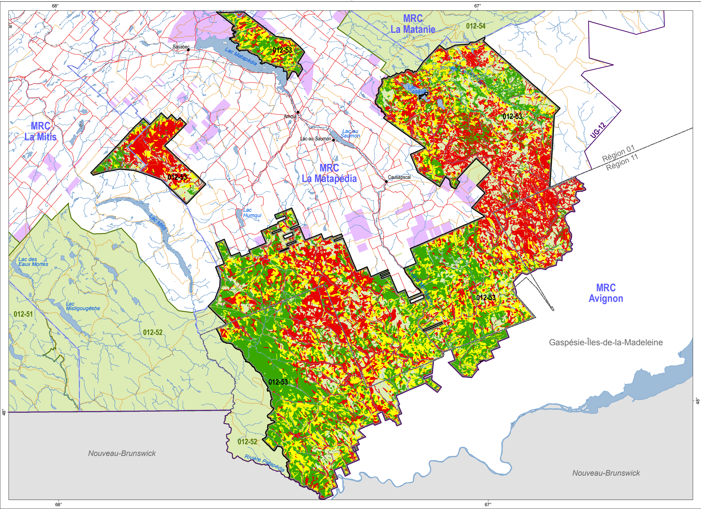
Figure 15 : Vulnérabilité à la tordeuse des bourgeons de l'épinette Unité d'aménagement 012-53
