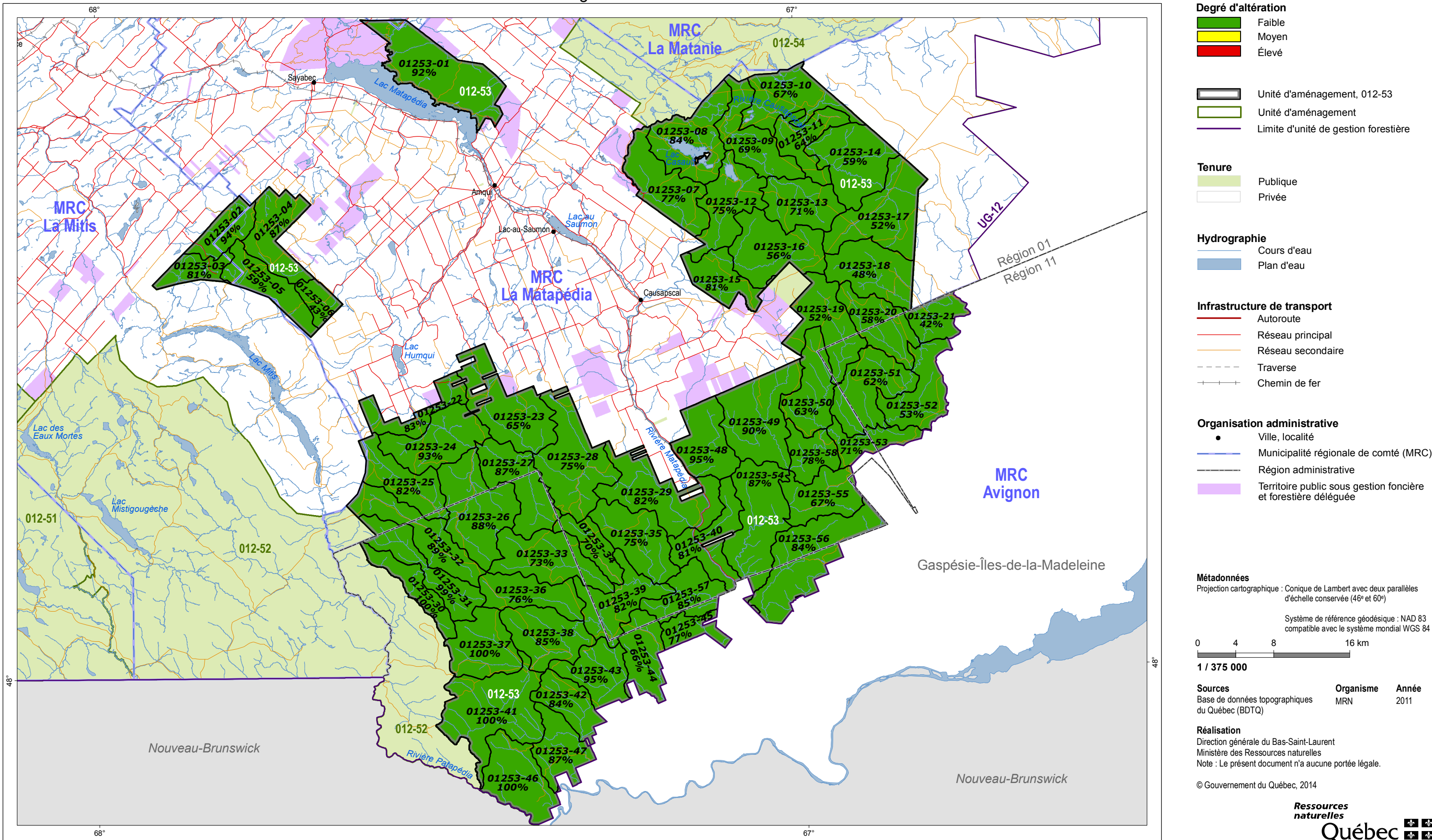
Figure 29 : Proportion de la forêt de 6 mètres et plus (habitat de la martre) Unité d'aménagement 012-53
