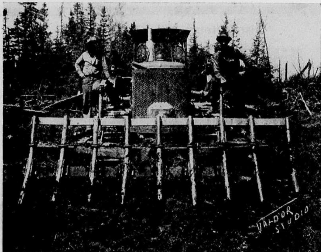
Voici une "grippe" à essouchement telle qu'inventée par M. l'abbé Georges Béland et M. Paul-Emile Ayotte de Val Senneville. Cette machine rénovera complètement le métier harassant du défricheur en simplifiant le travail et gardant au sol toutes ses propriétés cultivables.
