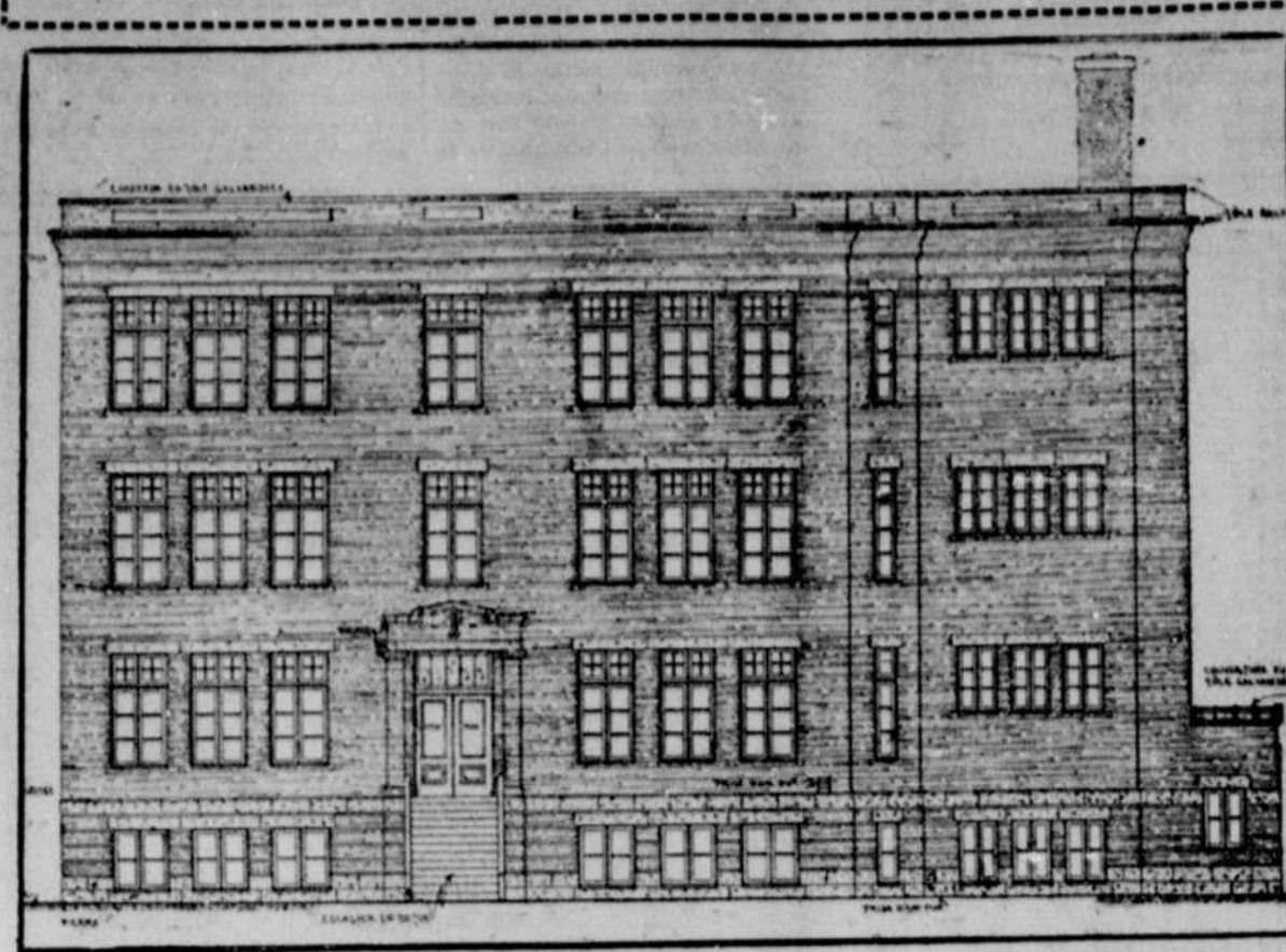
Plan de la nouvelle école que la Commission scolaire va construire dans la paroisse de St-François d'Assise de Québec. Ces plans ont été préparés par MM. Tanguay et Chénier.
