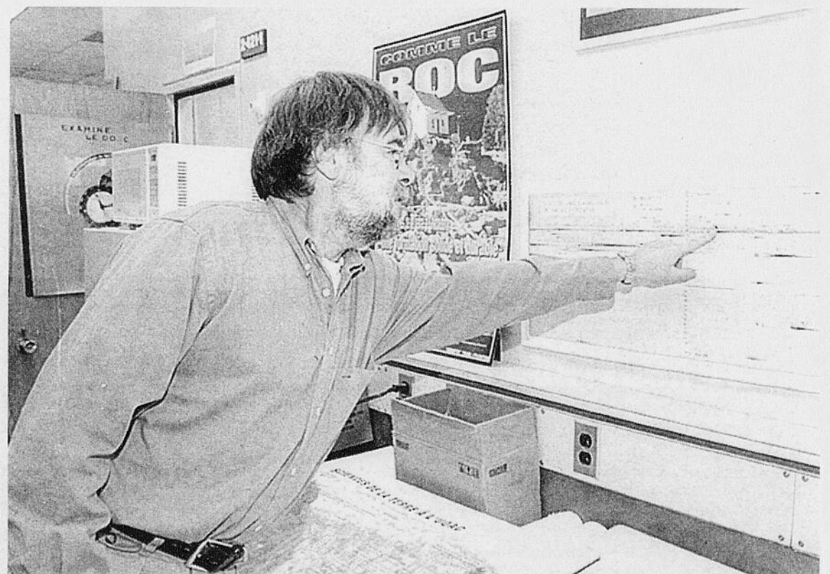
RISQUES - Selon Raynald Duberger, les tremblements de terre comportent des risques pour des infrastructures lourdes comme les grands barrages, les centrales nucléaires et les usines de produits chimiques.
