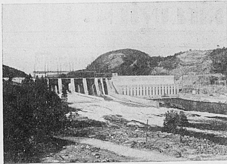
Vue d'aval du barrage et de la centrale électrique de la St. Maurice Power Corporation à La Tuque. P. Q. L'aménagement initial comprend quatre générateurs de 44,500 h.p., qui fonctionneront tous à la fin de l'année. L'usine peut recevoir six générateurs d'une capacité de 267,000 h.p.
