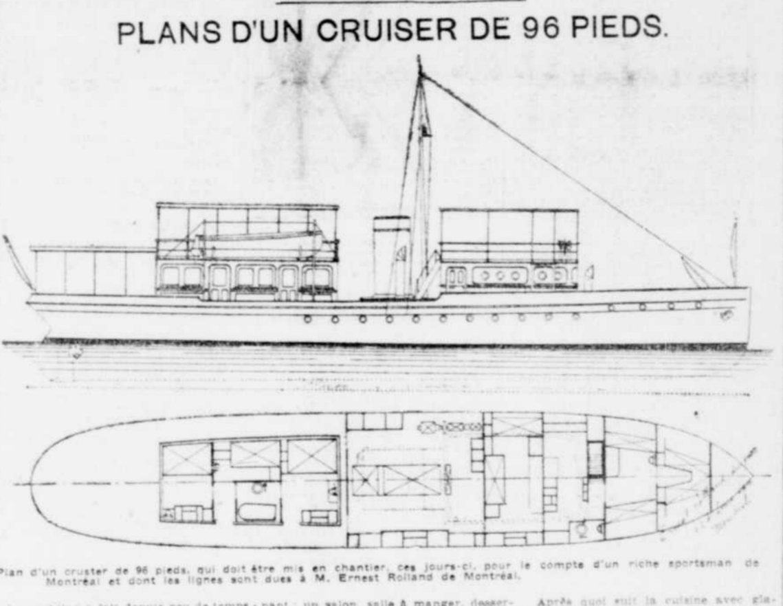
Plan d'un cruiser de 96 pieds, qui doit être mis en chantier ces jours-ci, pour le compte d'un riche sportsman de Montréal et dont les lignes sont dues à M. Ernest Roland de Montréal.
