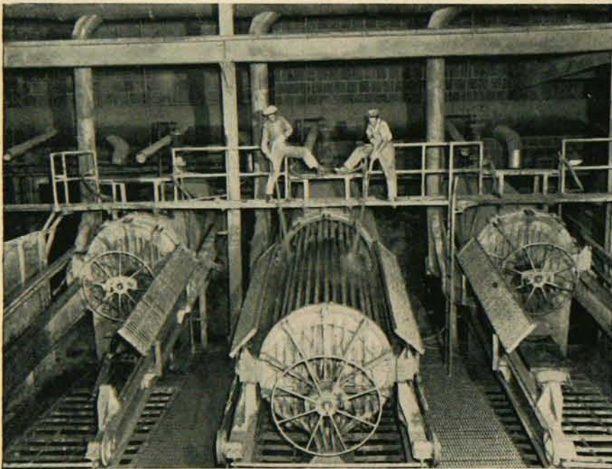
Une des phases préliminaires d'une métallurgie fort compliquée. L'extraction de l'aluminium suppose de nombreuses opérations échelonnées sur 50 à 60 heures.
