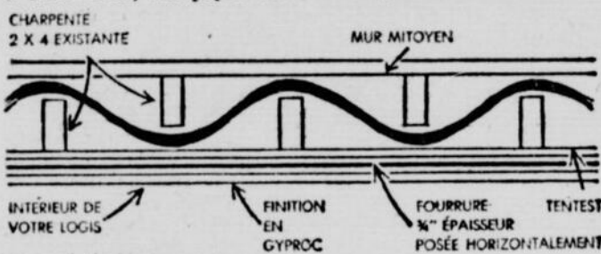
Plan d'un mur mitoyen avec insonorisation
