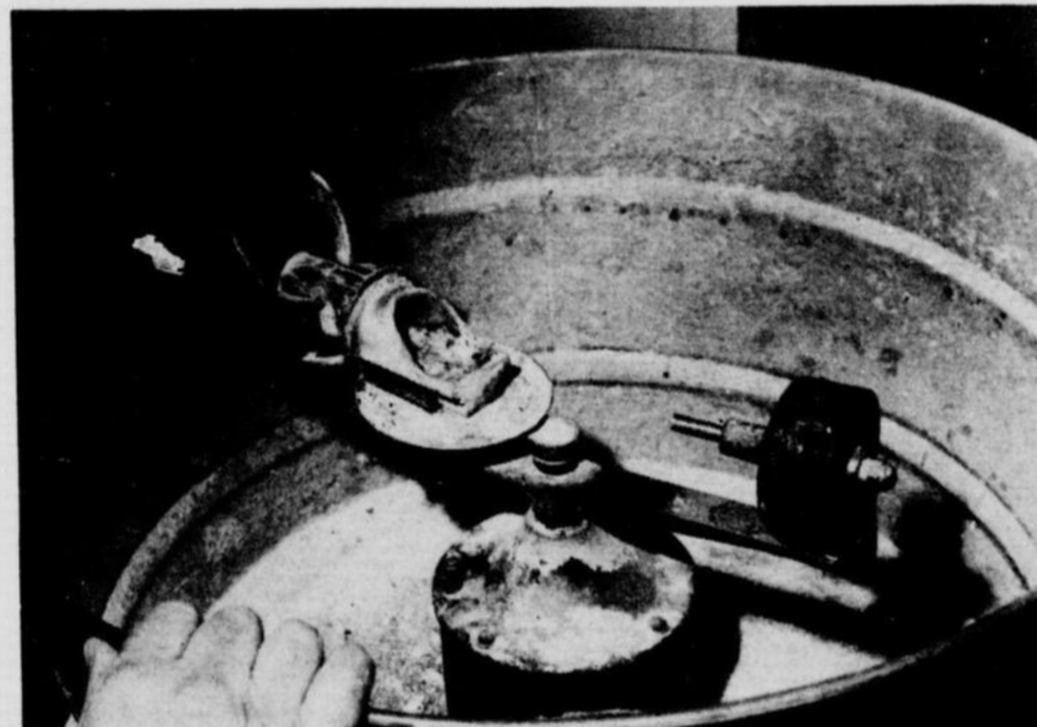
A l'aide d'une centrifugeuse, on projette le métal liquide dans les cavités laissées par la cire fondue. Quand on casse le plâtre, la pièce est complétée.
