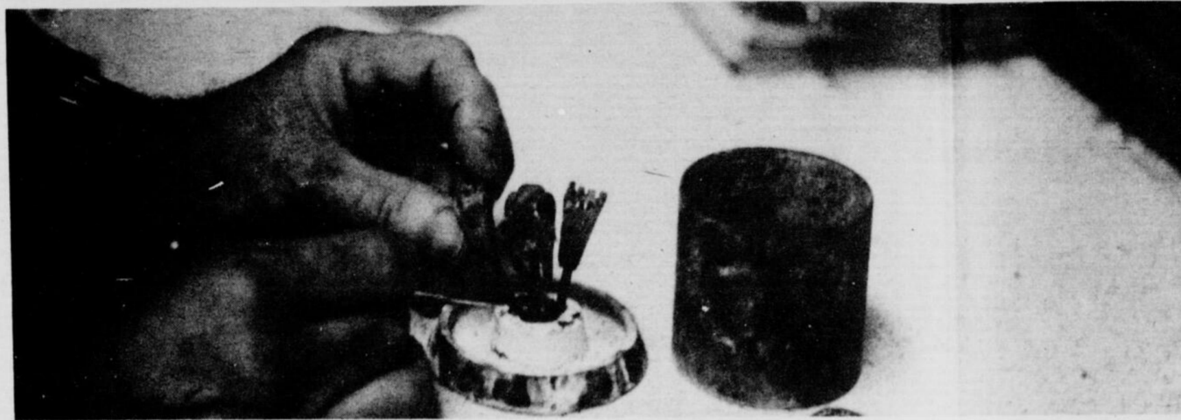
On élabore la pièce avec de la cire et on ajoute une tige. Puis on moule dans le plâtre et on fait fondre la cire.
