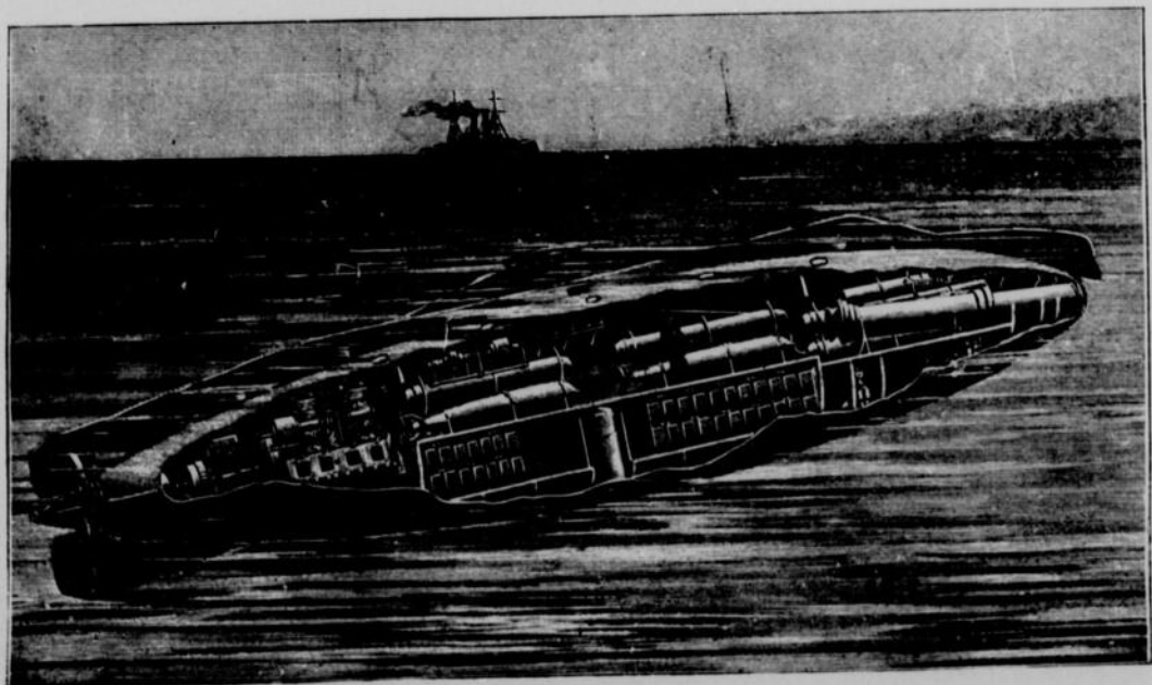
Le sous-marin "Fulton" acheté dernièrement aux Etats-Unis par la Russie. Ce navire vient, en manœuvrant, d'être avarié à Cronstadt. Notre gravure montre longitudinalement les appareils et machines, tels qu'ils sont à bord du "Fulton" en cours de route libre.
