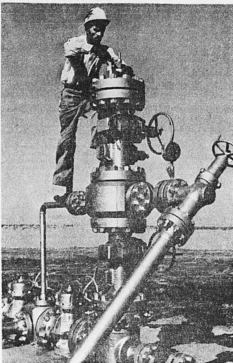
Un séparateur du genre appelé "arbre de Noël" en fonction sur l'emplacement d'un puits de pétrole, près de Dammam, en Arabie Saoudite.
